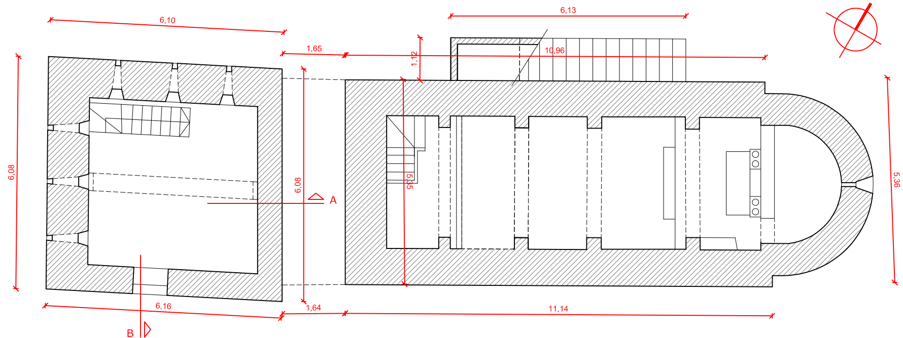
PLANTA COR DEL CONJUNT
