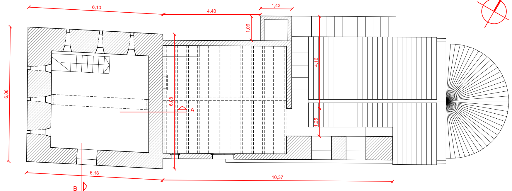
PLANTA RECTORIA DEL CONJUNT
