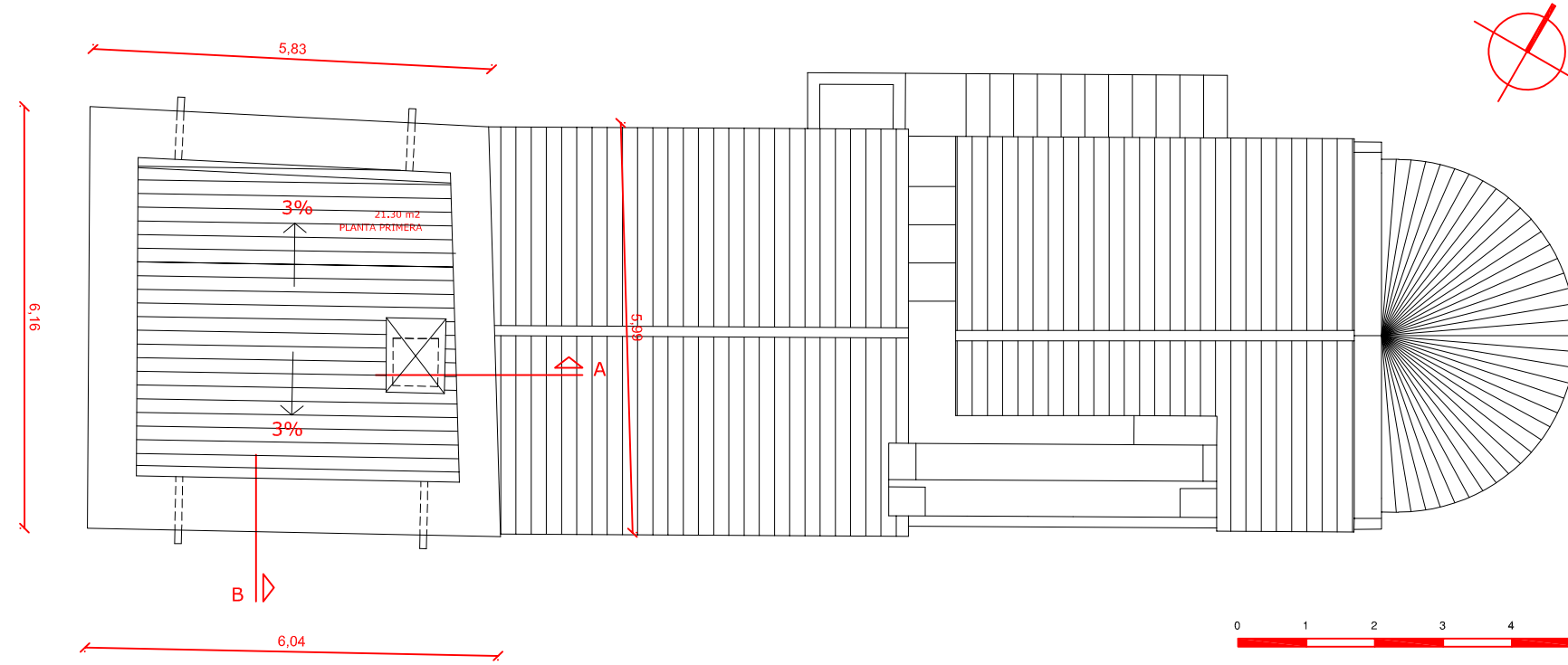
PLANTA COBERTA DEL CONJUNT
