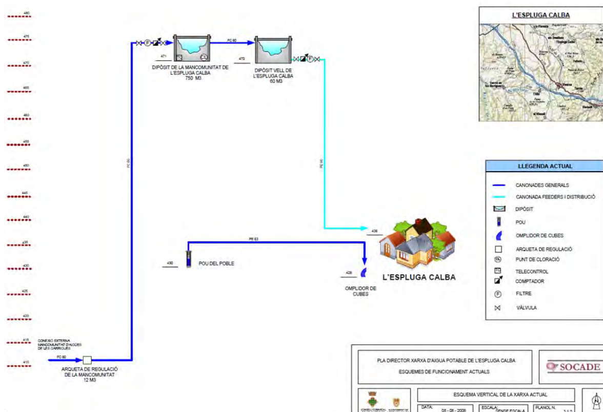
Esquema vertical de la xarxa actual. Font: Pla Director d'Aigua Potable de L'Espluga Calba
