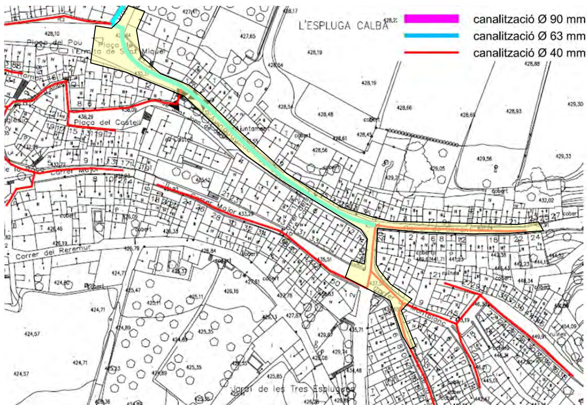
Imatge desplegament gas canalitzat
