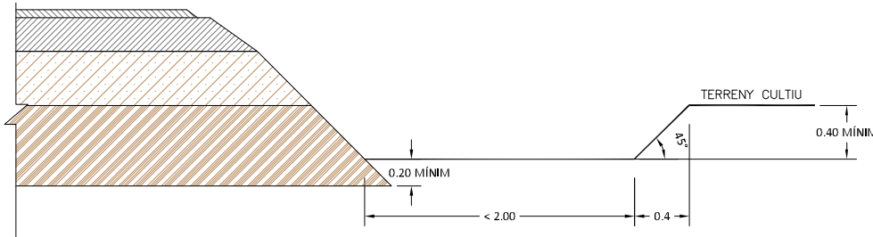
CUNETA FINS A 2M
