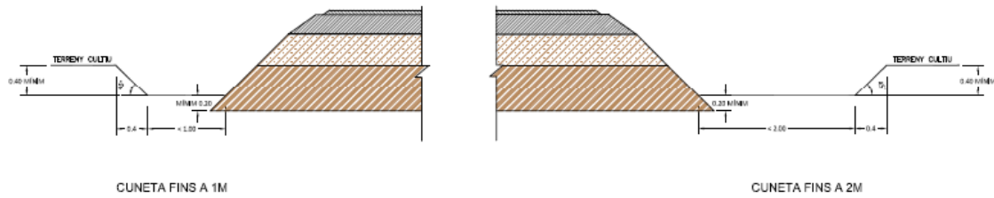
Figura 6. Secció tipus. Font: elaboració pròpia.
