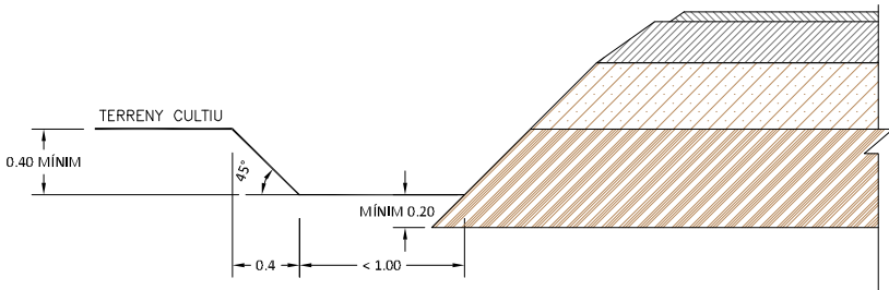
CUNETA FINS A 1M
