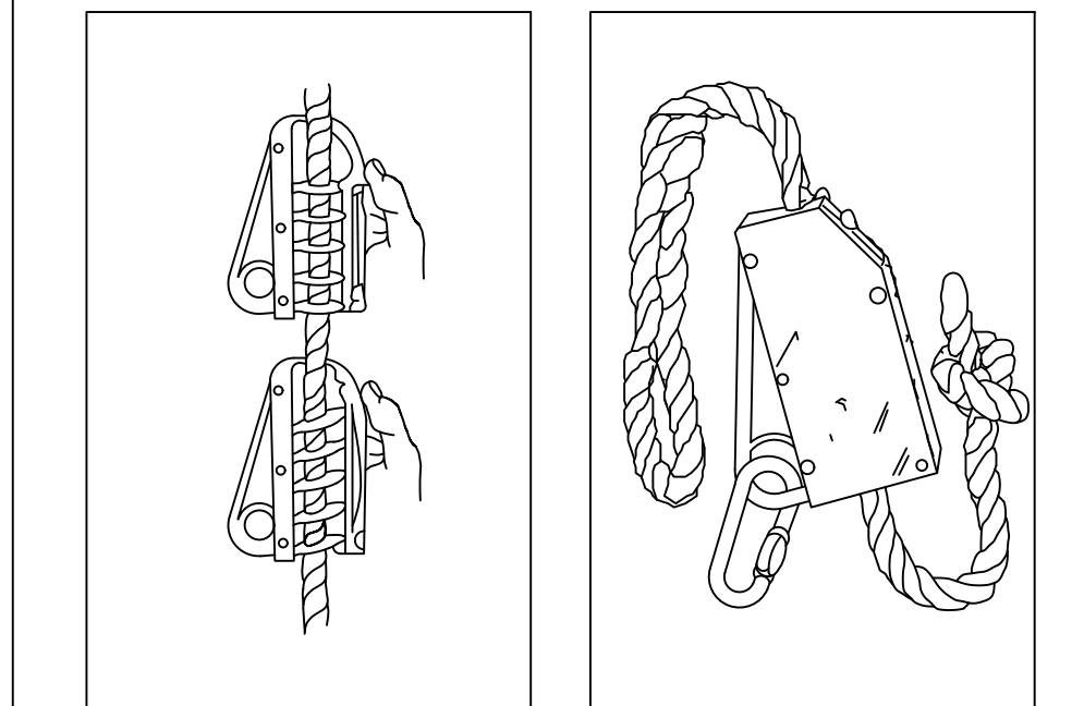
Ancoratge cinturó de seguretat (segur d'ancoratge mòbil)
