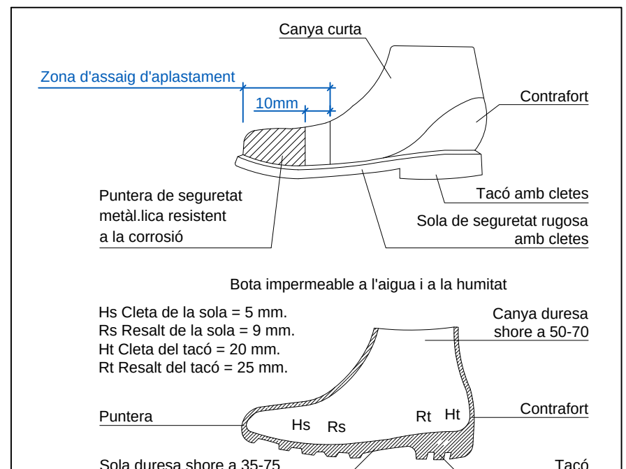
Bota de seguretat classe III
