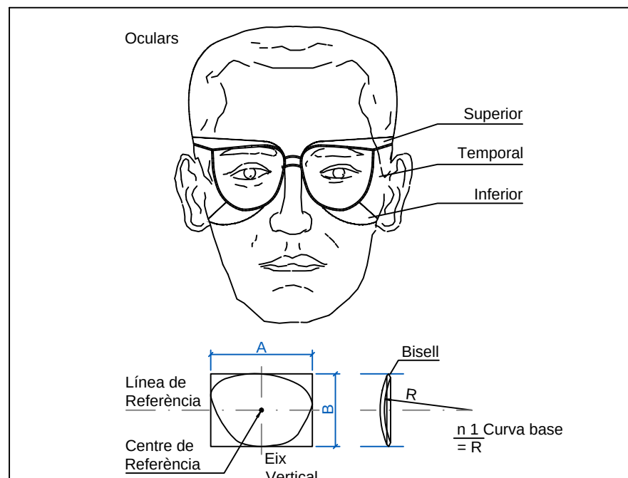
Proteccions individuals (ulleres de seguretat)
