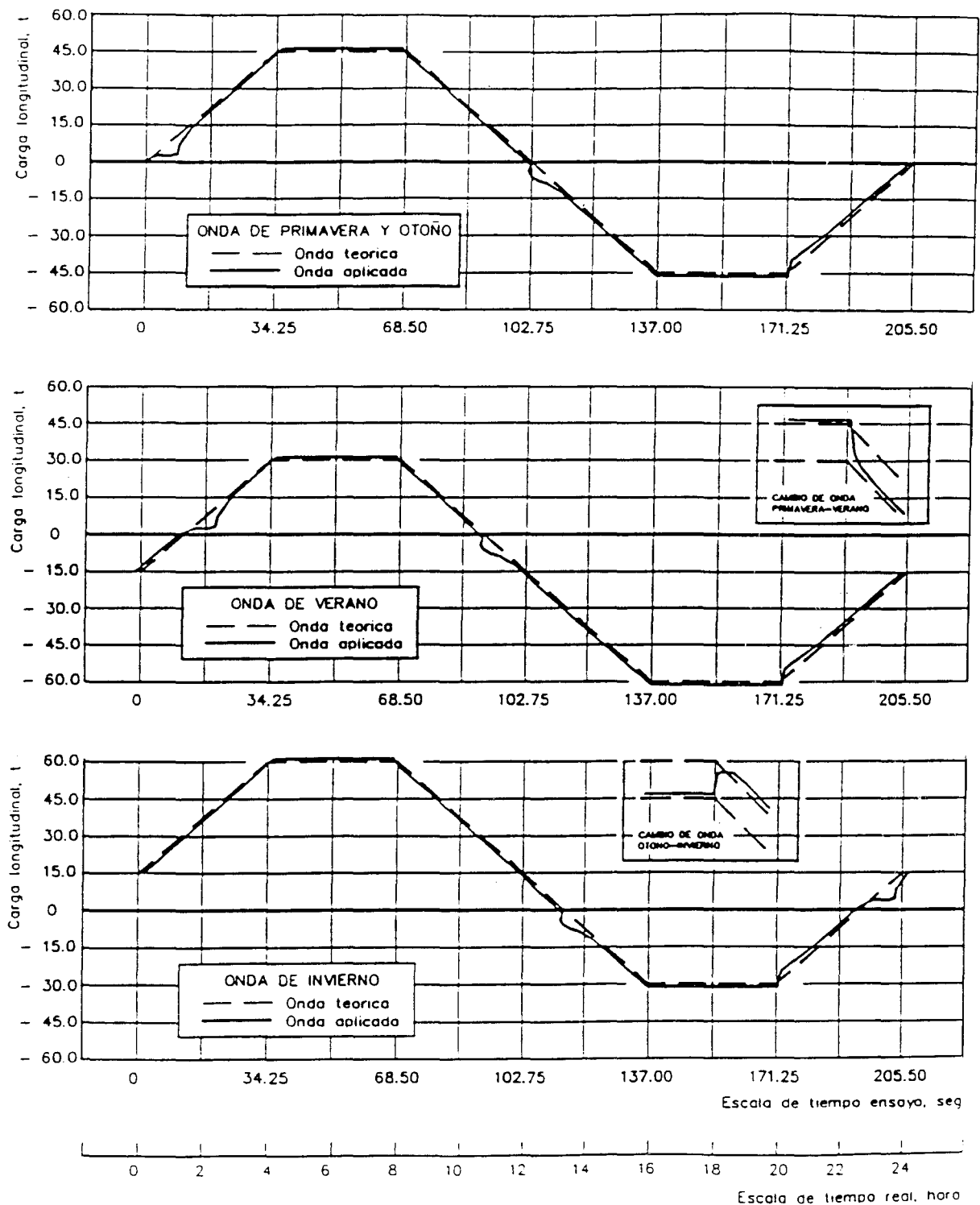
Ondas de carga longitudinal teoricas y realmente aplicadas (Carril UIC-60)
