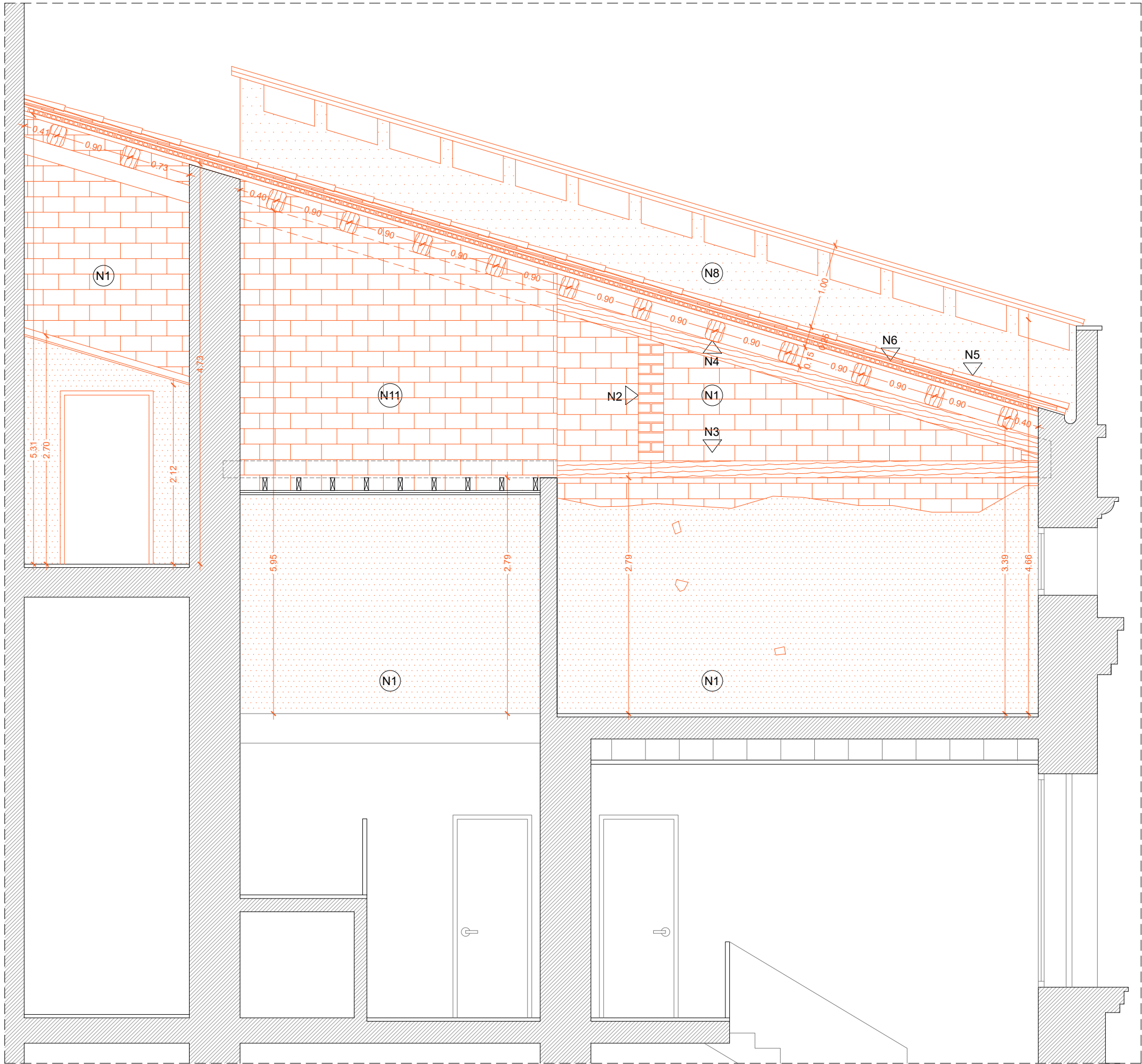
SECCIÓ TRANSVERSAL ST1
