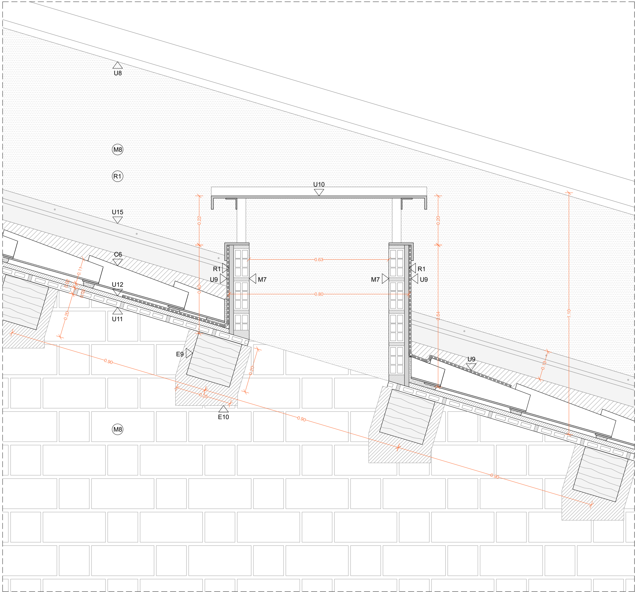
DETALL D02
