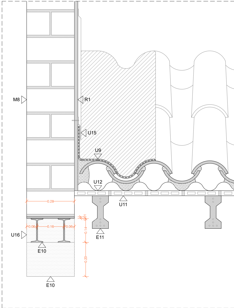
DETALL D07
