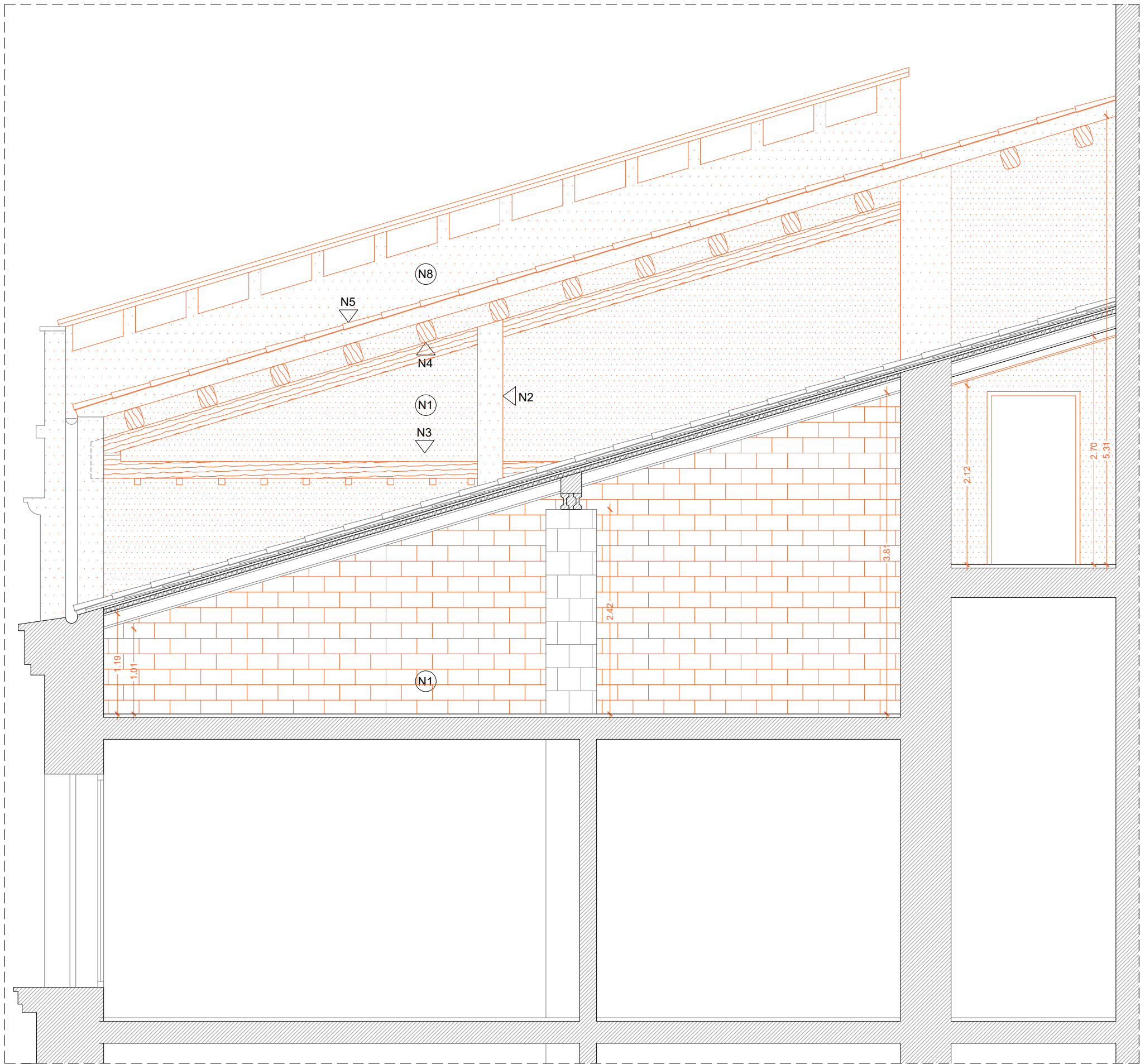
SECCIÓ TRANSVERSAL ST2
