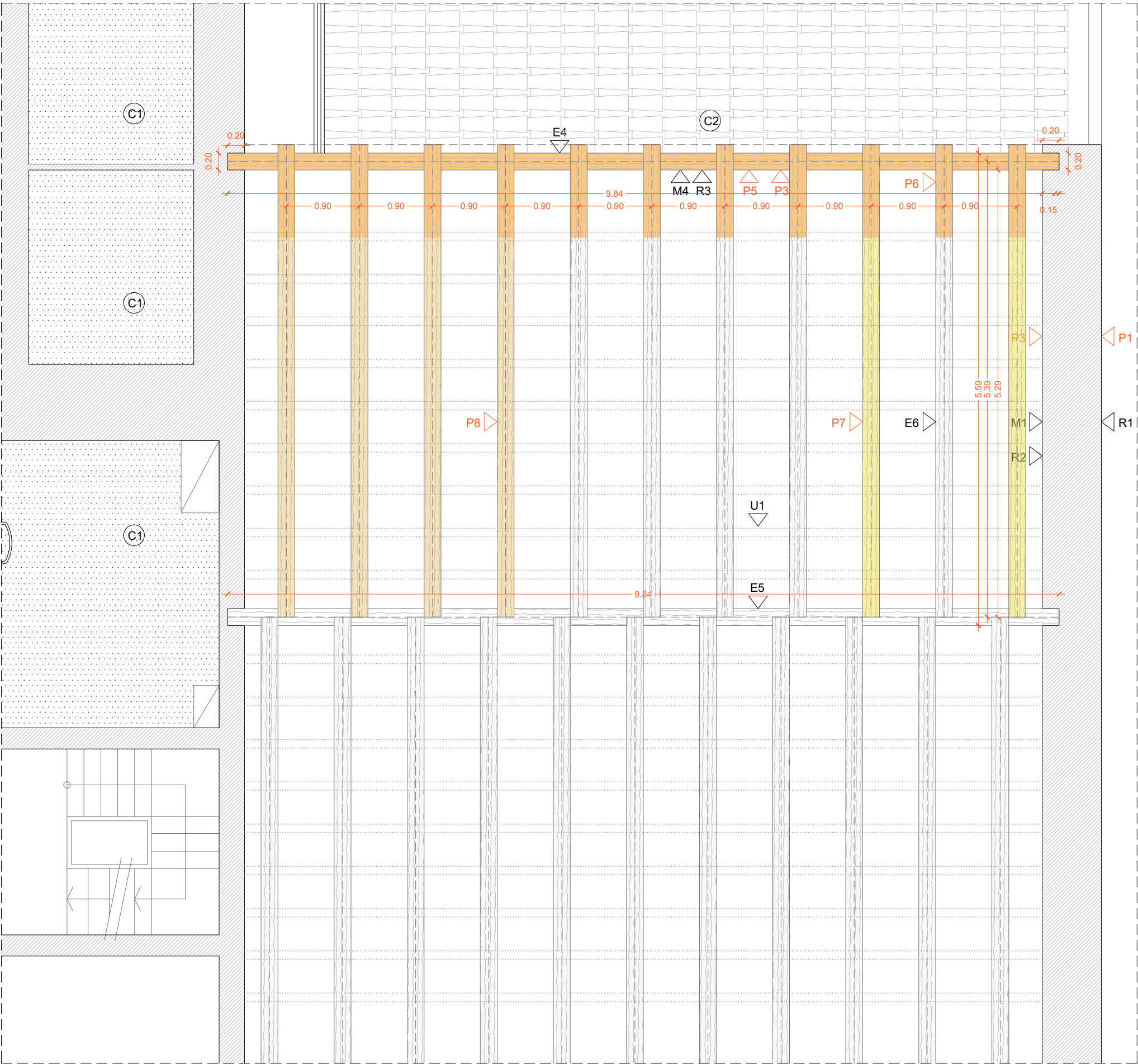
SOSTRE PLANTA SEGONA DETALL
