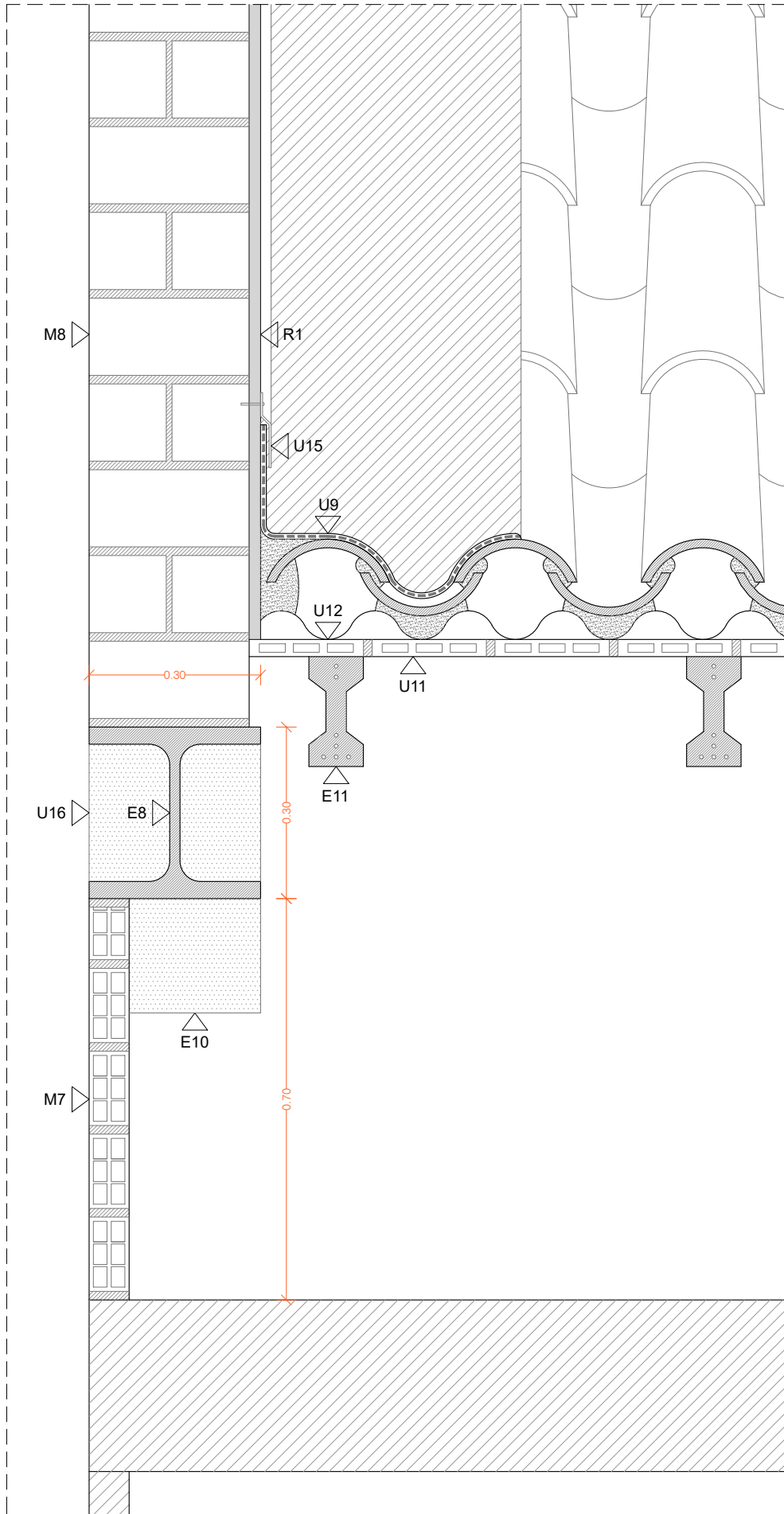
DETALL D05
