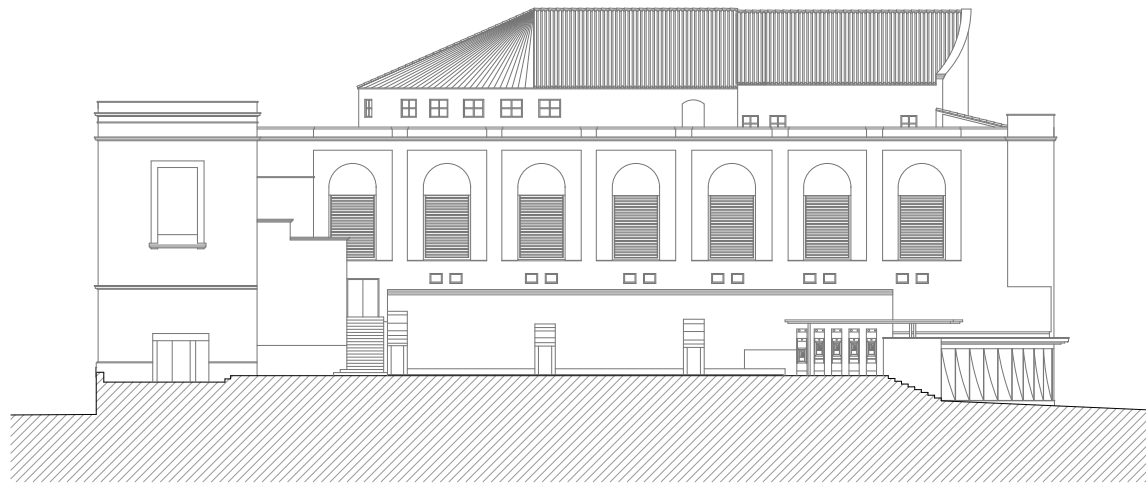
ALÇAT EST - PLAÇA SANT DOMÈNEC
