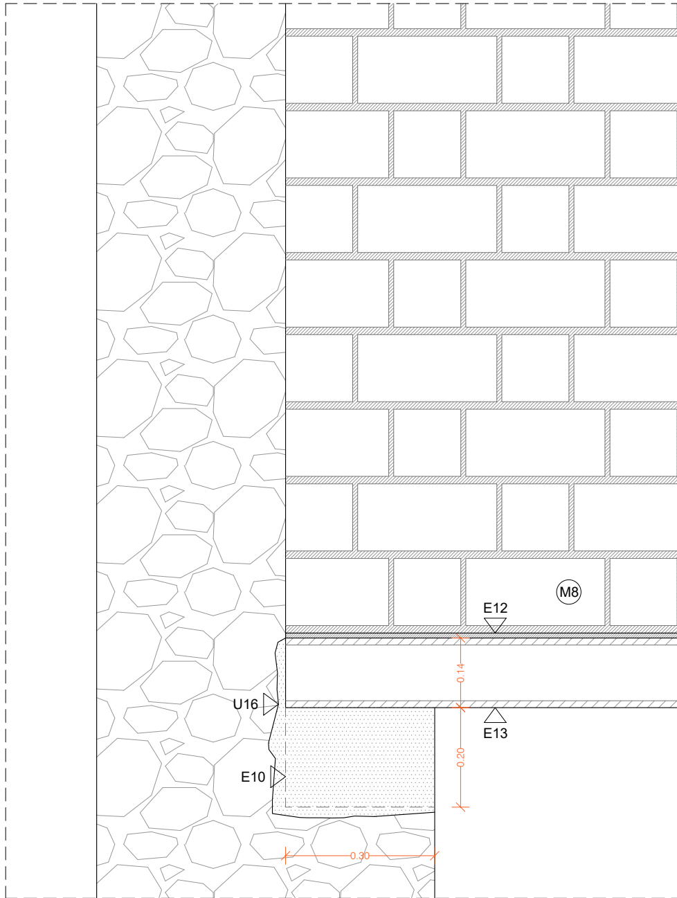
DETALL D08
