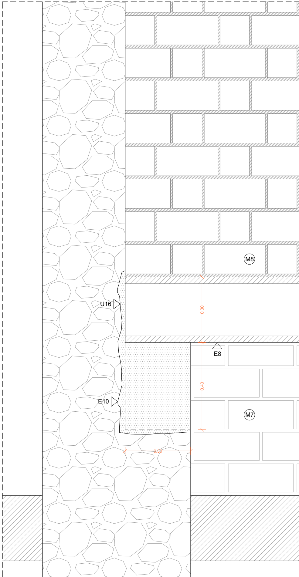
DETALL D06
