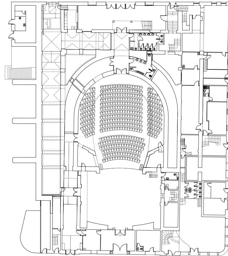
PLANTA BAIXA
