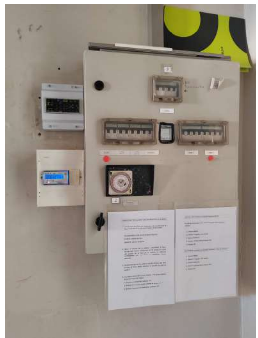
Quadre caldera
