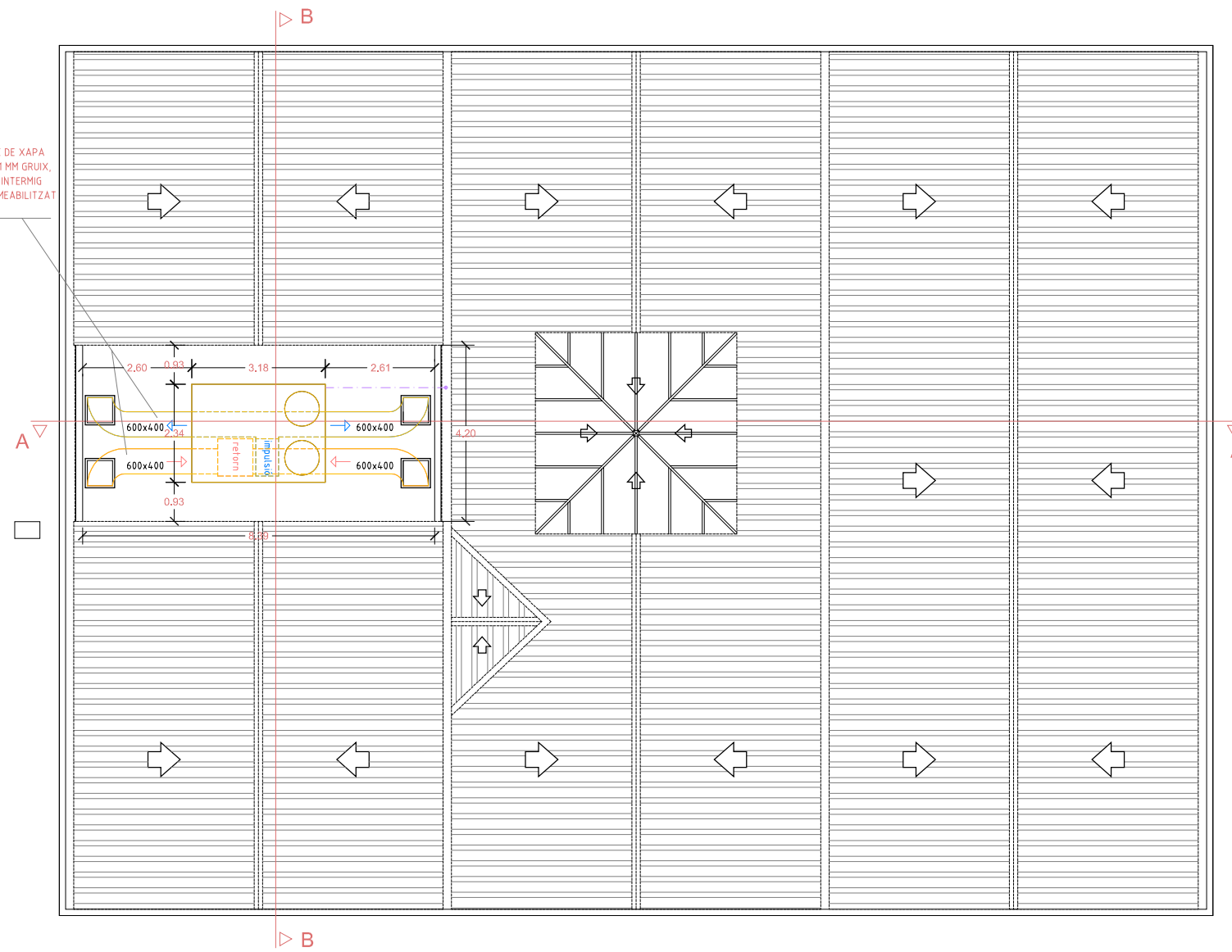
PLANTA COBERTA
