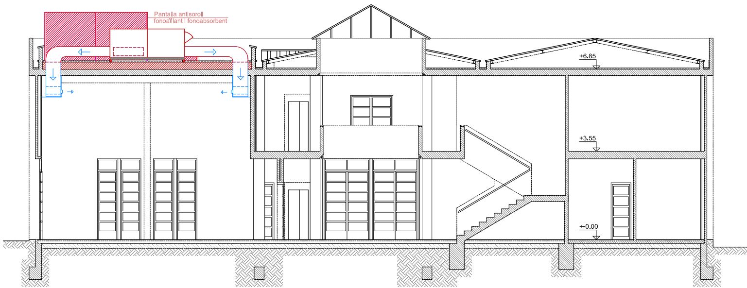
Secció A-A'
