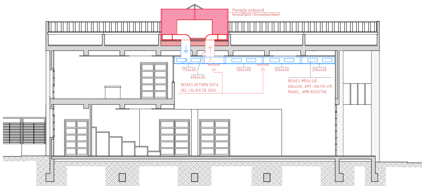
Secció B-B'
