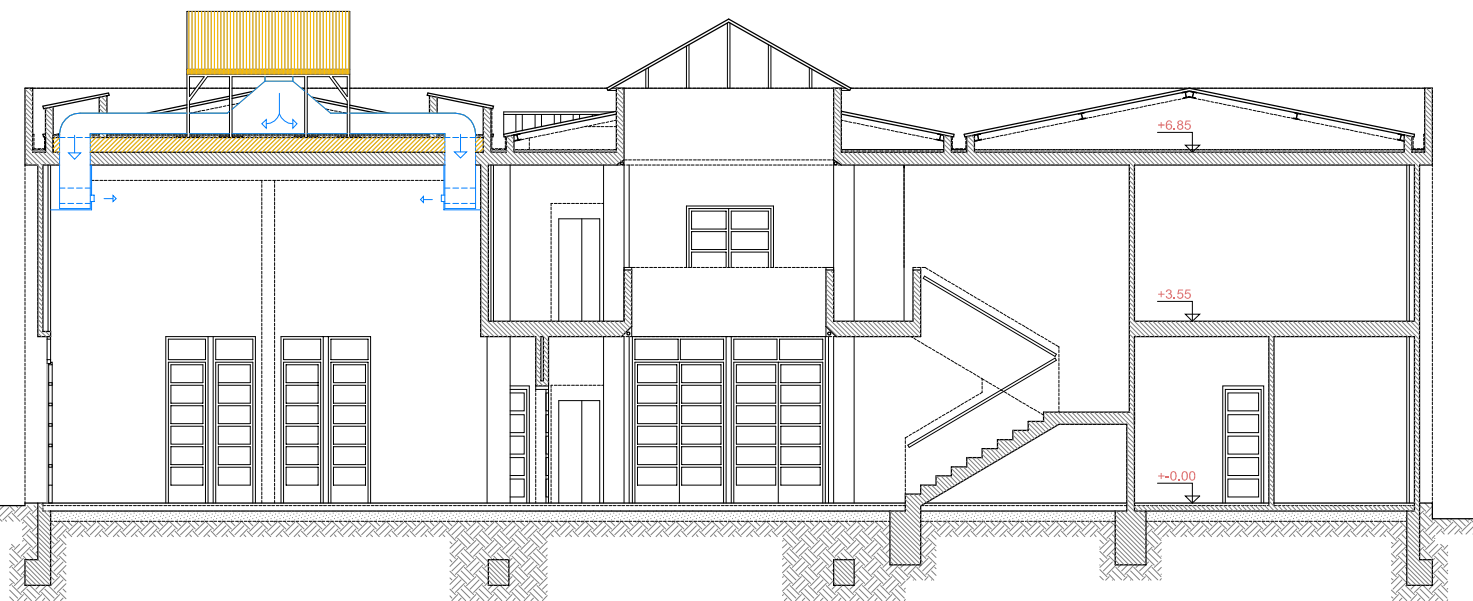
Secció A-A'
