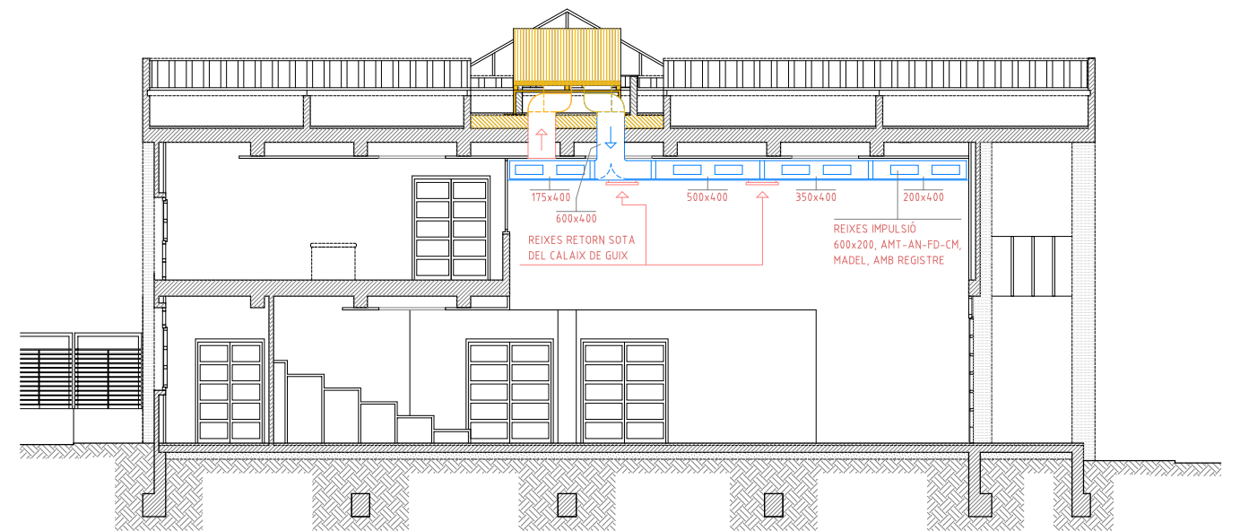
Secció B-B'
