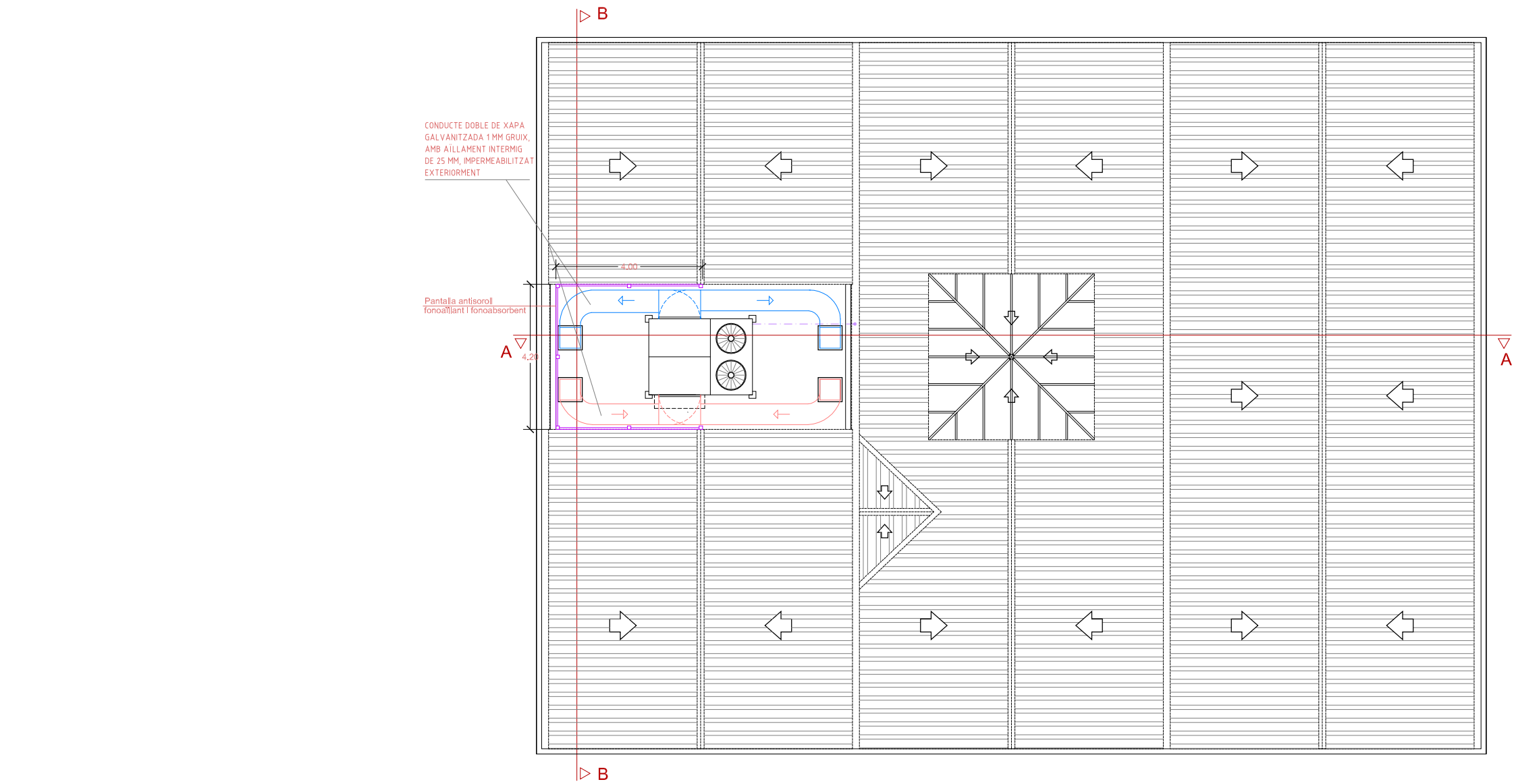
PLANTA COBERTA
