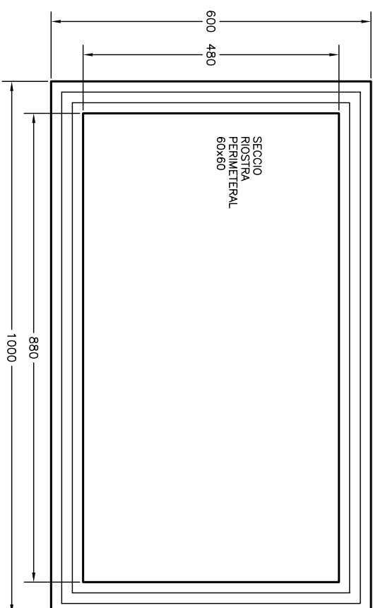
PLANTA FONAMENTS
