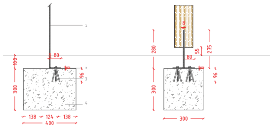
ANCORATGE PEU COR-TEN Escala 1:10
