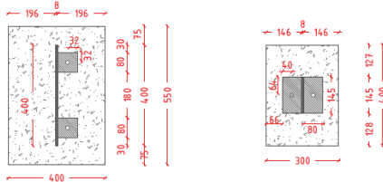
ANCORATGE PEU COR-TEN Escala 1:10
