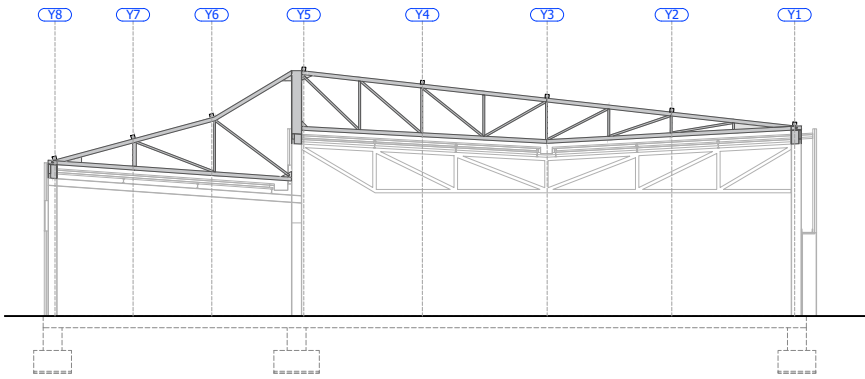
SECCIÓ TRANSVERSAL ESTRUCTURA A-A'
