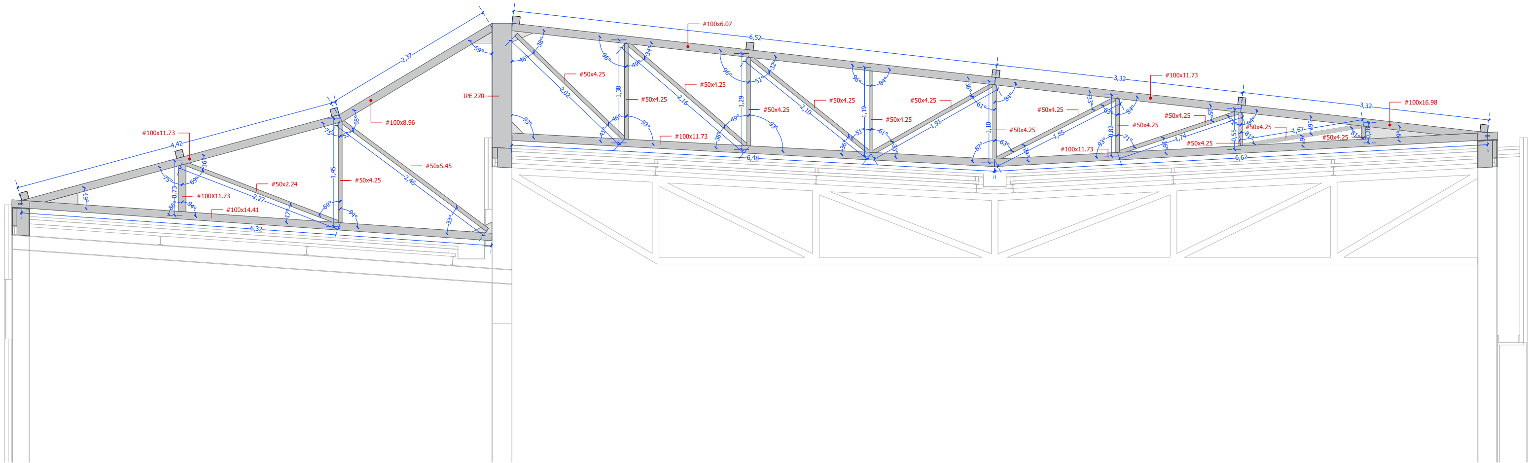
DETALL SECCIÓ TRANSVERSAL A-A'
