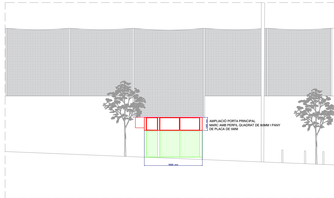
ALÇAT ENTRADA PRINCIPAL
