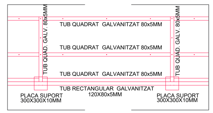
DETALL ESTRUCTURA
