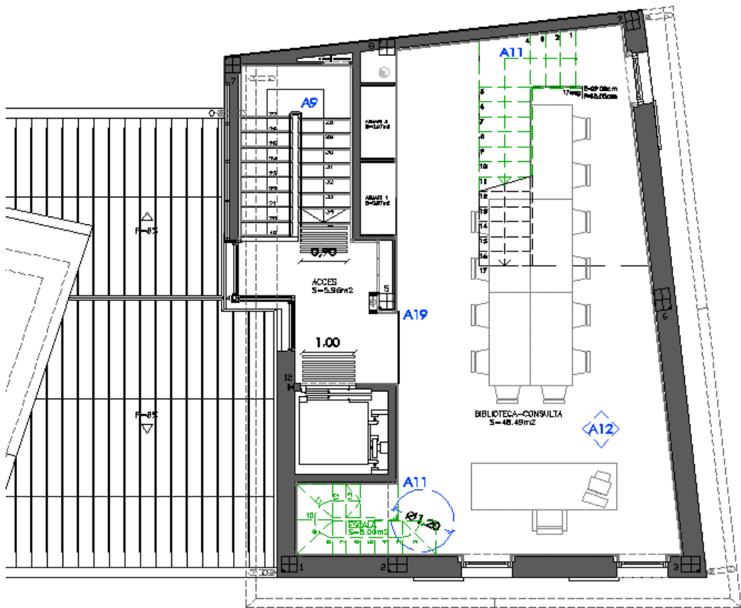
PLANTA SEGONA
