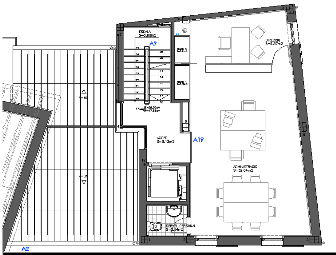
PLANTA SEGONA
