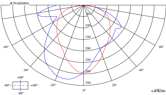
Curvas polares
