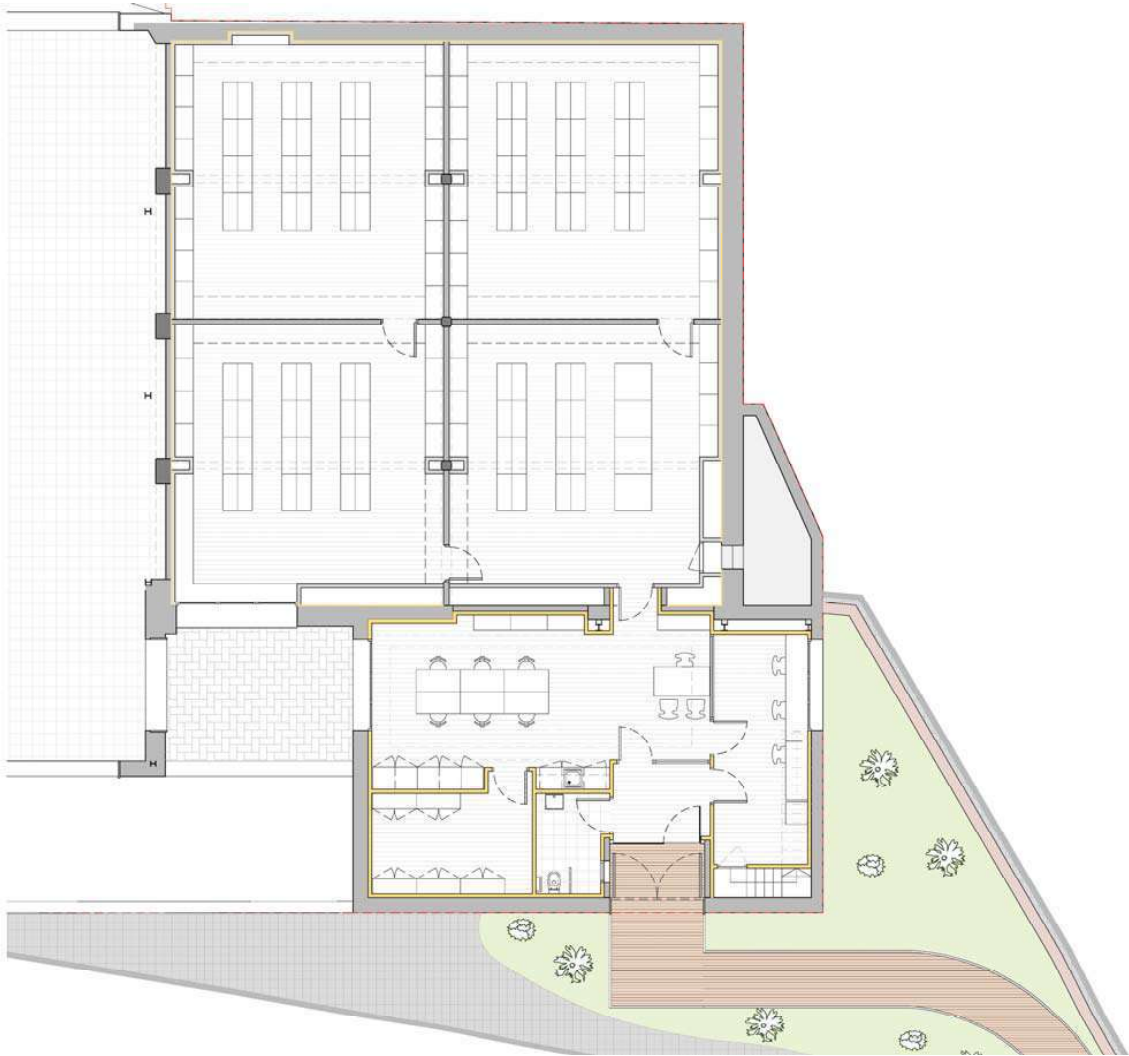
Proposta per a l'adequació d'una zona de l'edifici com a arxiu municipal.
