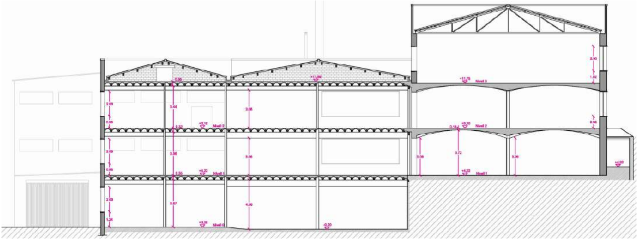
Secció de l'edifici actual.
