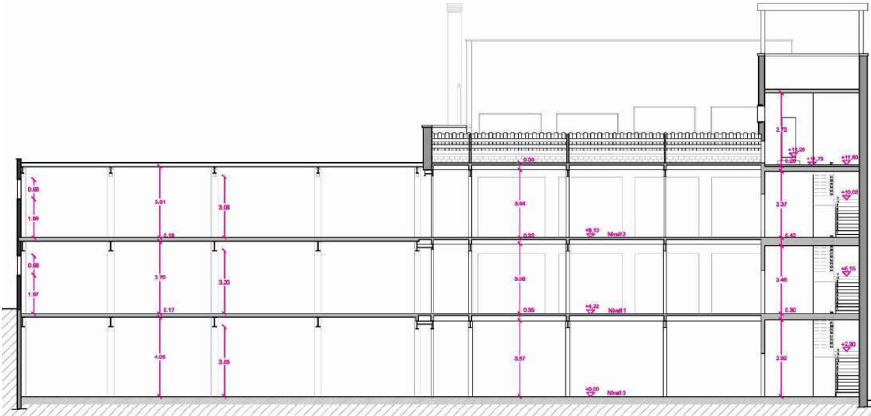
Secció de l'edifici actual.
