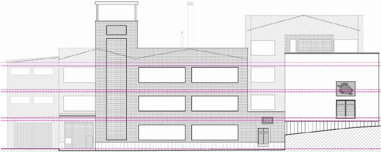
Actual façana nord-est de l'edifici.
