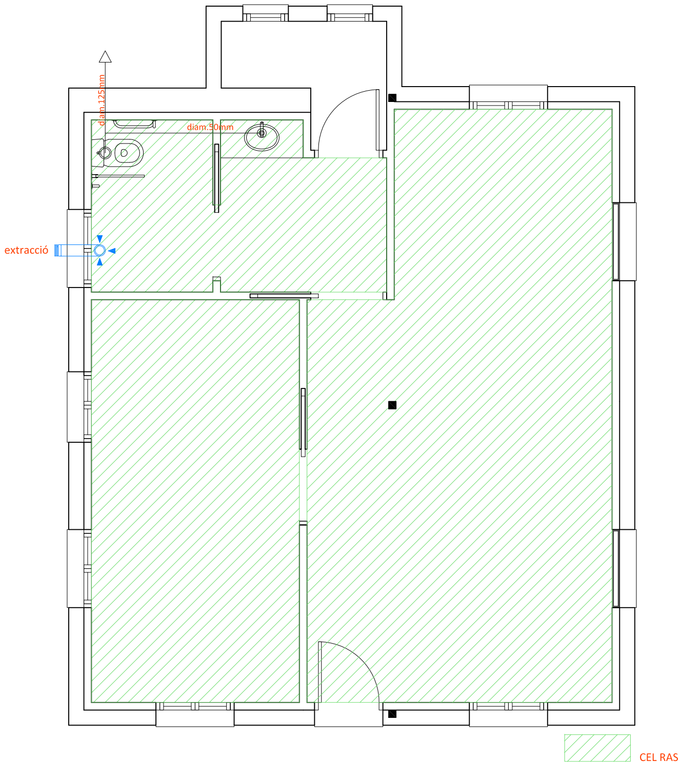
Planta baixa - Estat modificat
