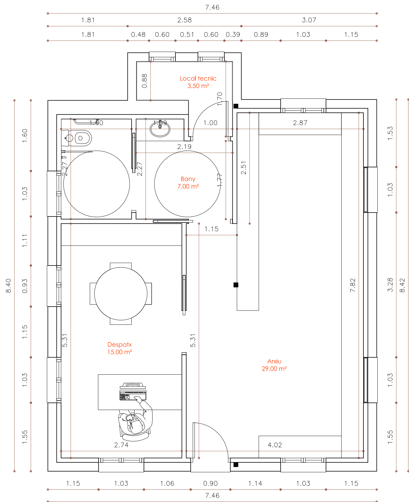
Planta baixa - Estat modificat
