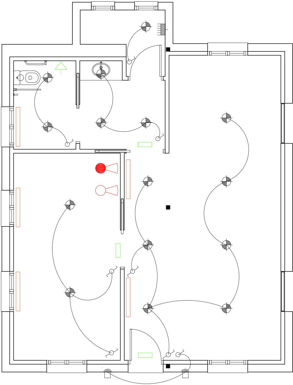
Planta baixa - Electricitat
