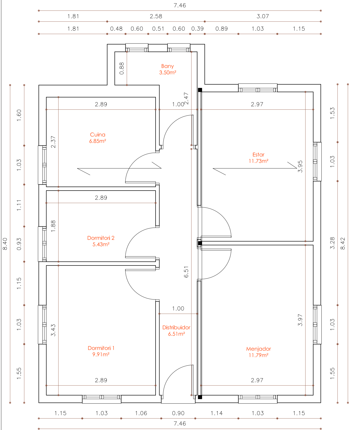
Planta baixa - Estat actual
