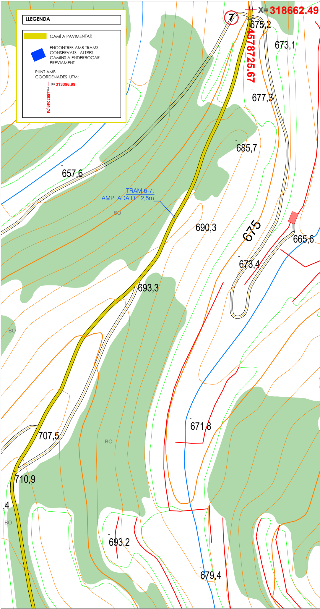
CAMÍ DE LA GARRIGA PLANTA ACTUACIÓ | E:1/1500
