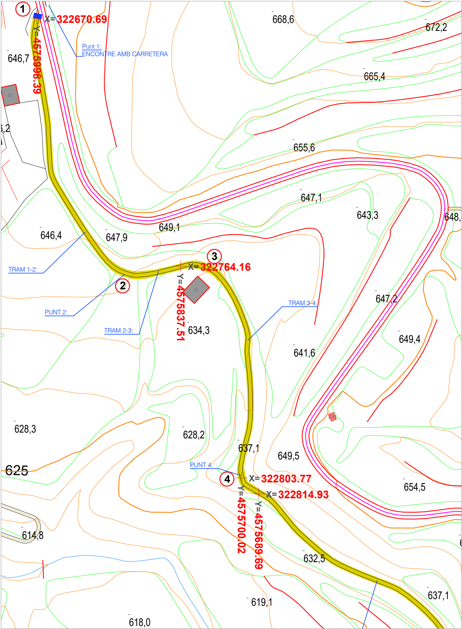
CAMÍ VELL DE CORNUDELLA PLANTA ACTUACIÓ | E:1/1500
