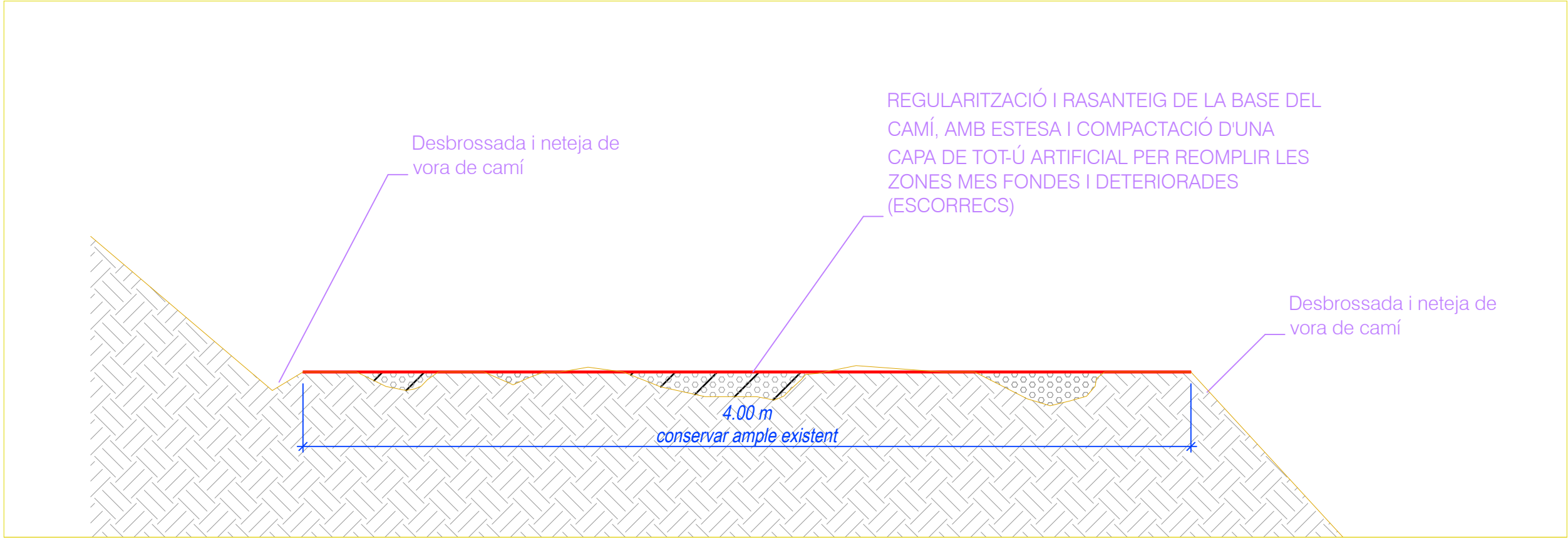
CAMÍ DE LA GARRIGA DETALL SECCIÓ FERM | E:1/120
