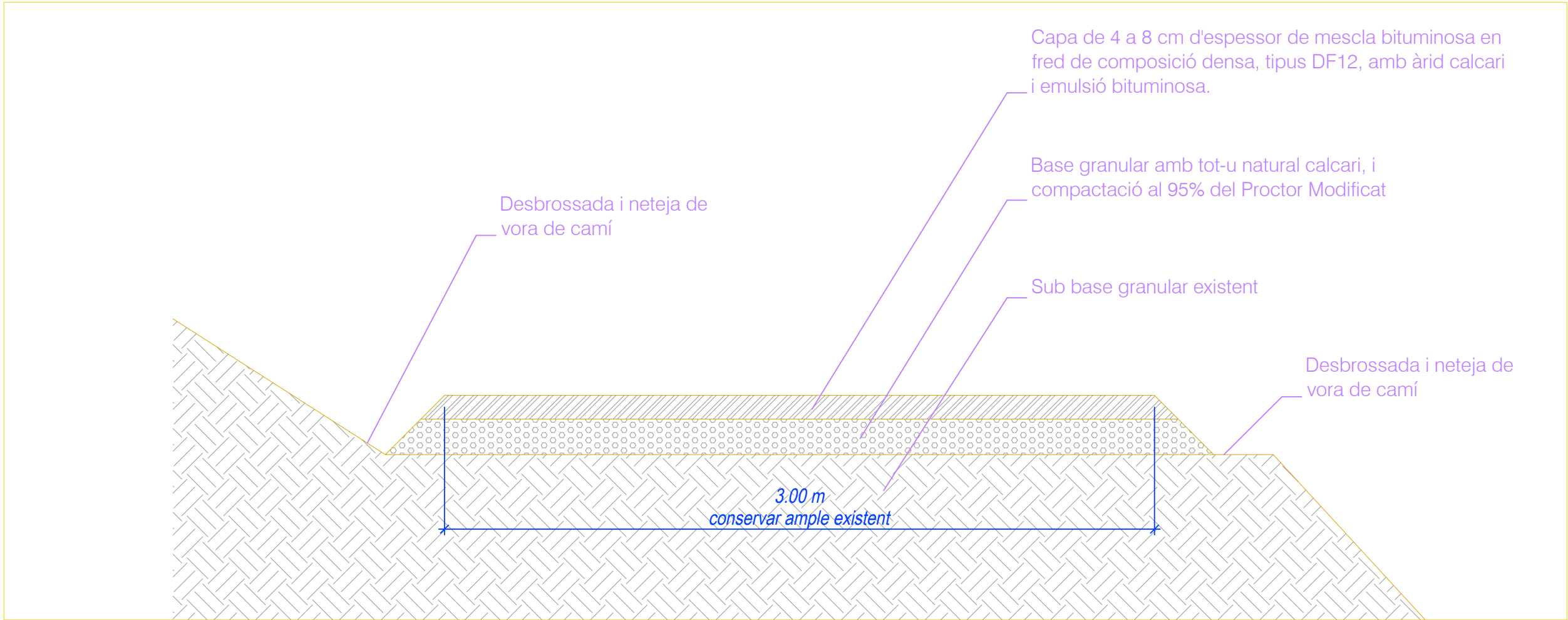
CAMÍ VELL DE CORNUDELLA DETALL SECCIÓ FERM | E:1/120
