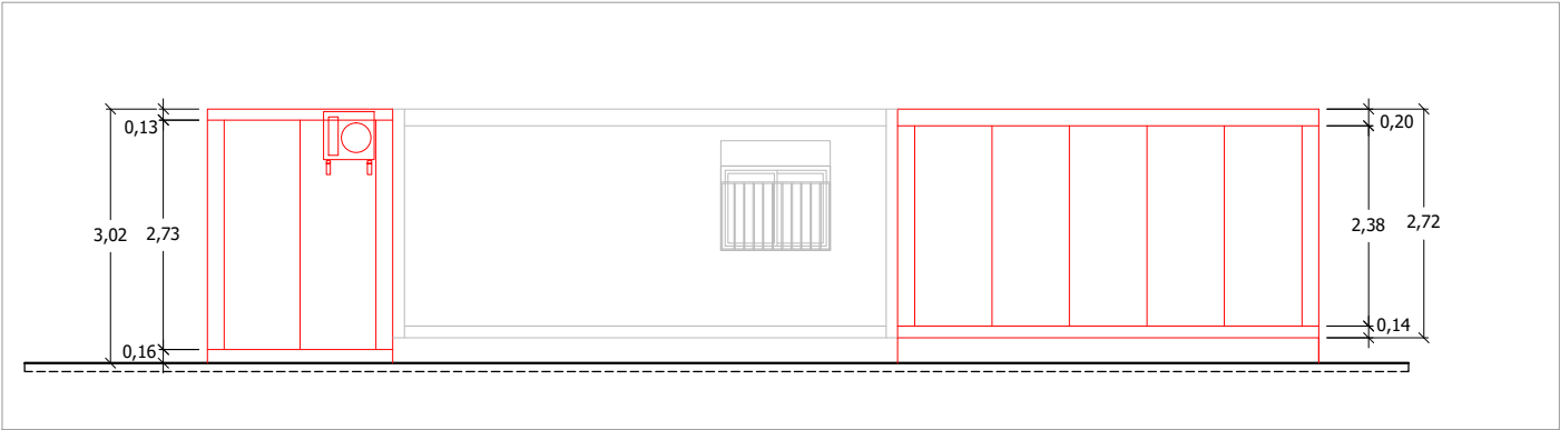
alçat 1
