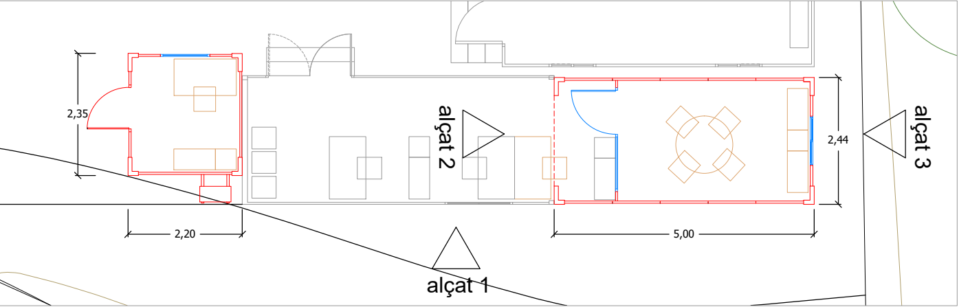
planta proposta
