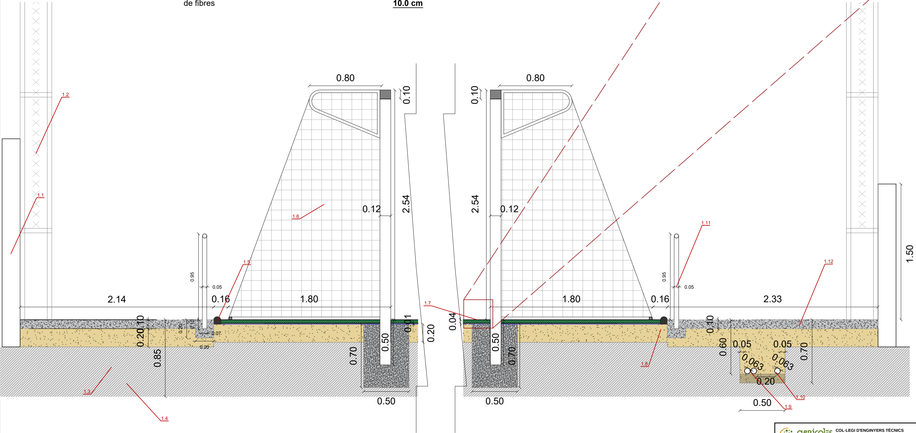
SECCIÓ LONGITUDINAL CONSTRUCTIVA
