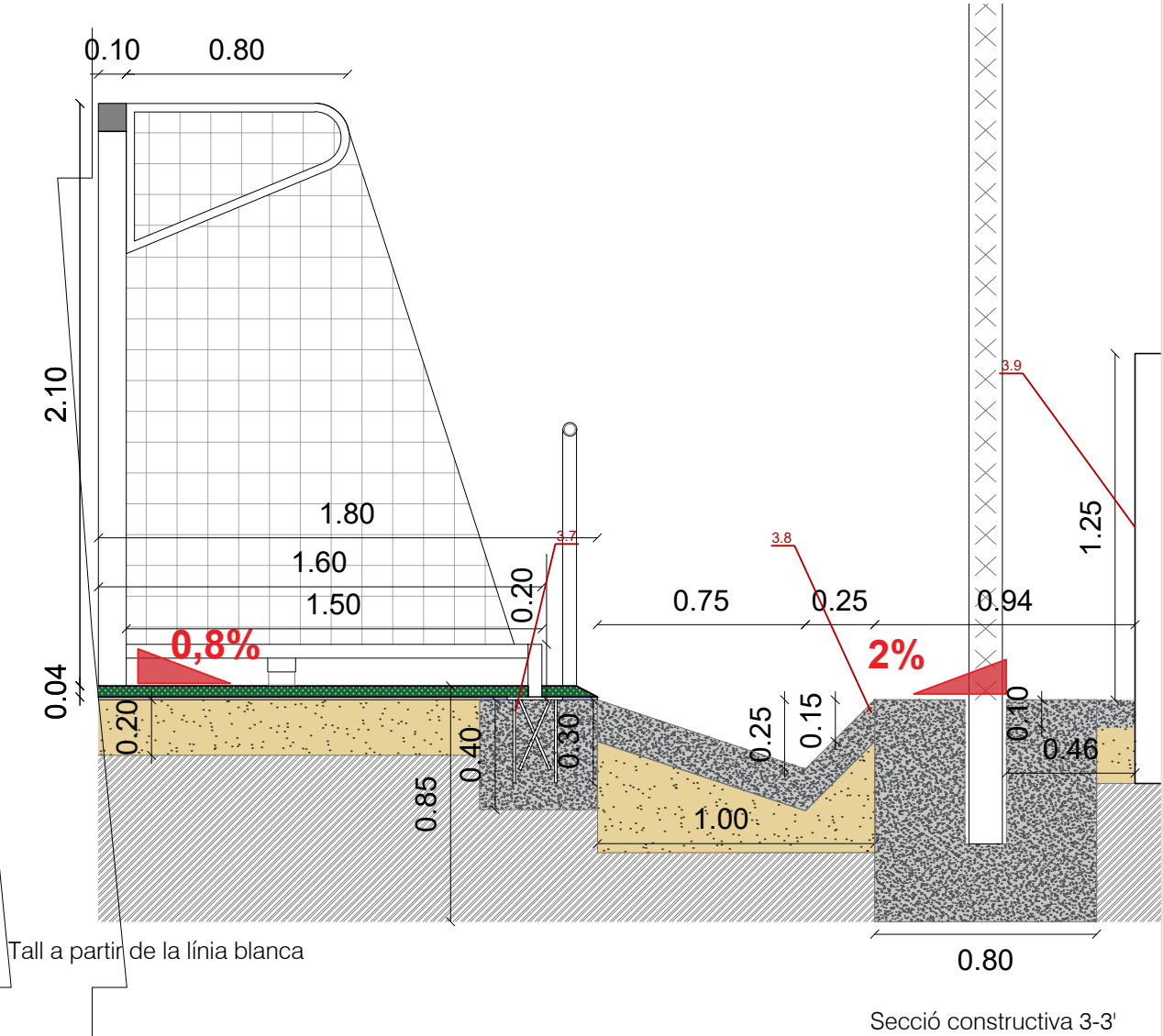
Secció constructiva 3-3'
