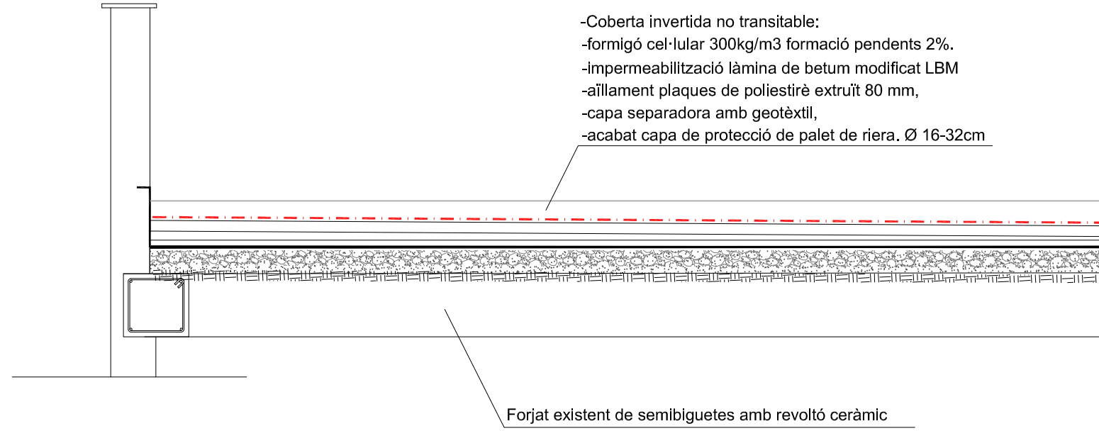
DETALL COBERTA INVERTIDA MODIFICADA
