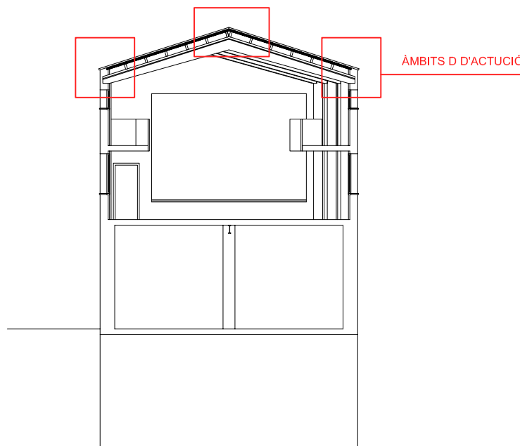
SECCIÓ A-A
