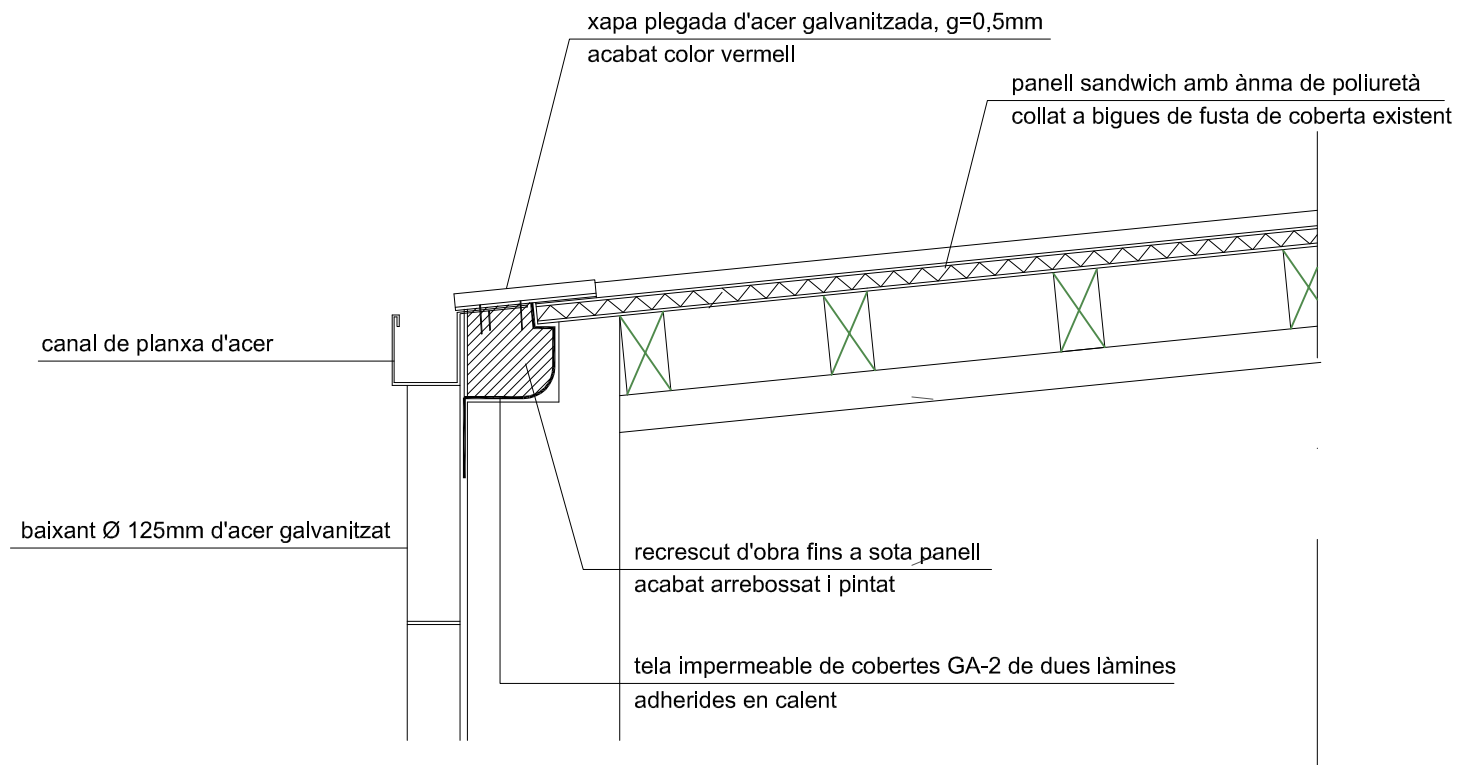
DETALL CANALERA MODIFICADA
