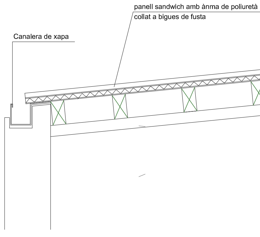
DETALL CANALERA ESTAT ACTUAL
