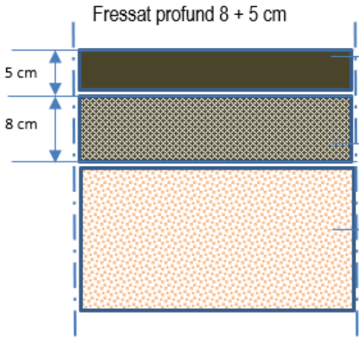
DETALL REFORÇ PROFUND
