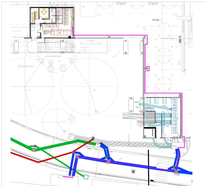
Recorregut temporal del cable d'alimentació al quadre d'enllumenat existent
