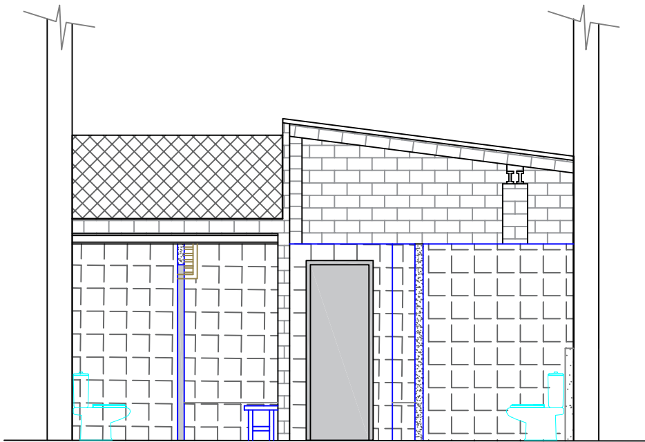
SECCIÓ C
