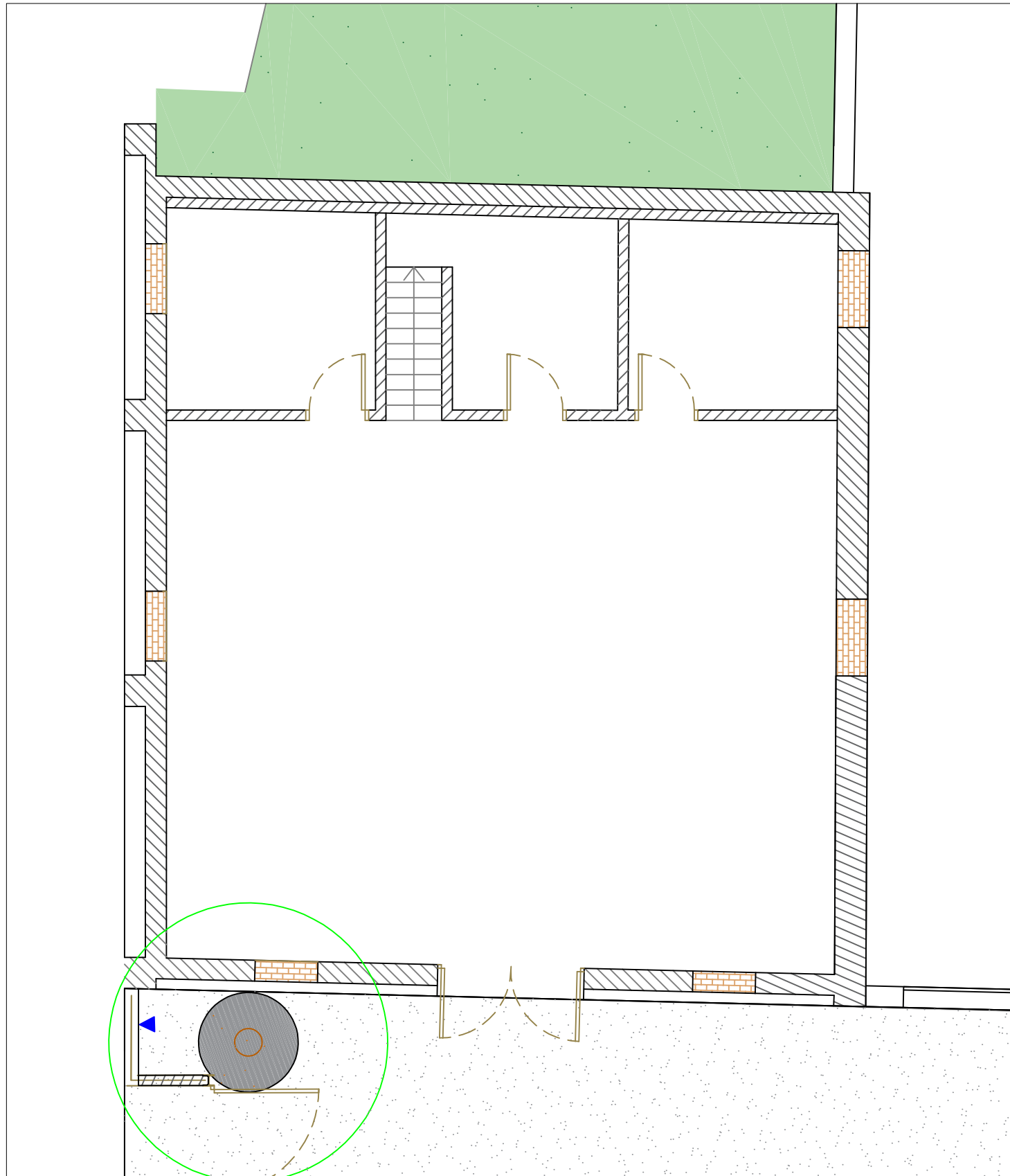
PLANTA BAIXA E:1/75
