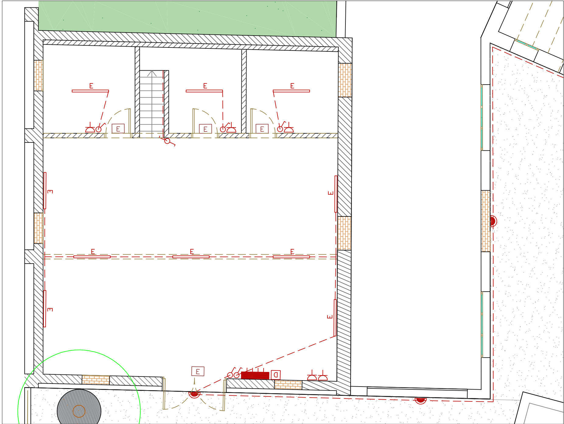
PLANTA BAIXA E:1/75
