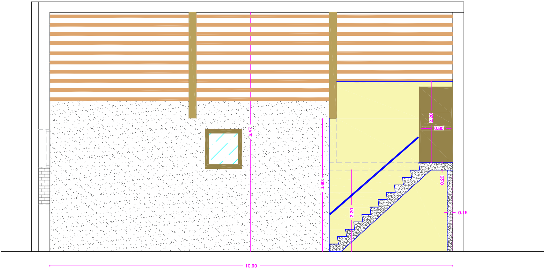
SECCIÓ A
