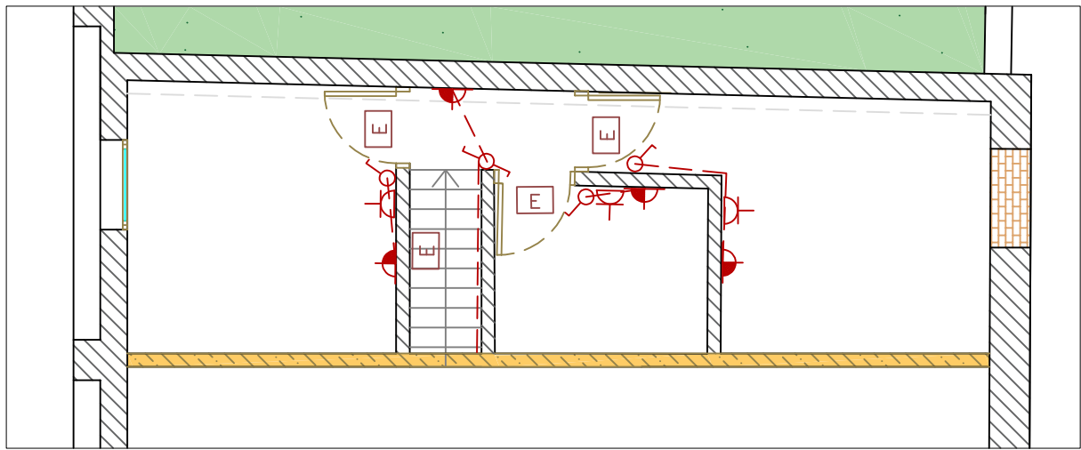
PLANTA ATELL E:1/75
