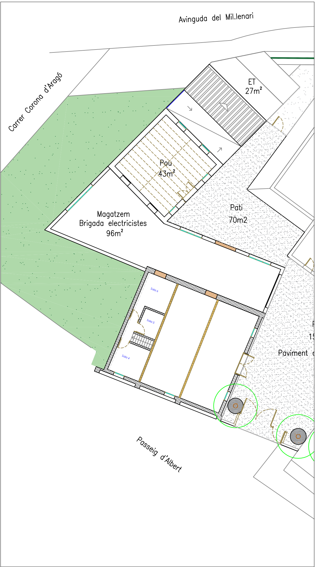
PLANTA SUPERIOR
