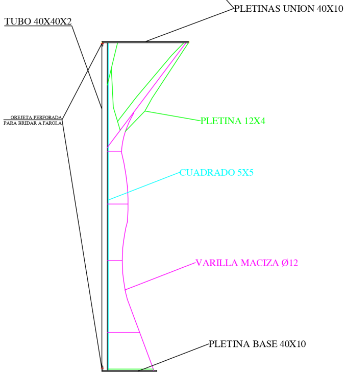
DESPIECE DE ESTRUCTURA
