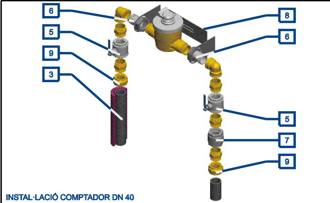
INSTAL·LACIÓ COMPTADOR DN 40
