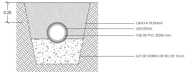
TUB DE DRENATGE - E:1/20
