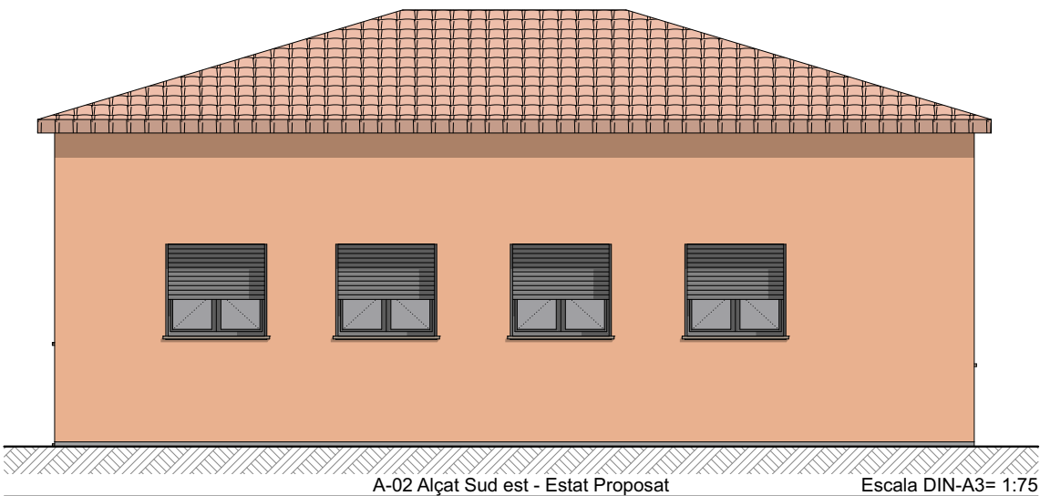
A-02 Alçat Sud est - Estat Proposat
