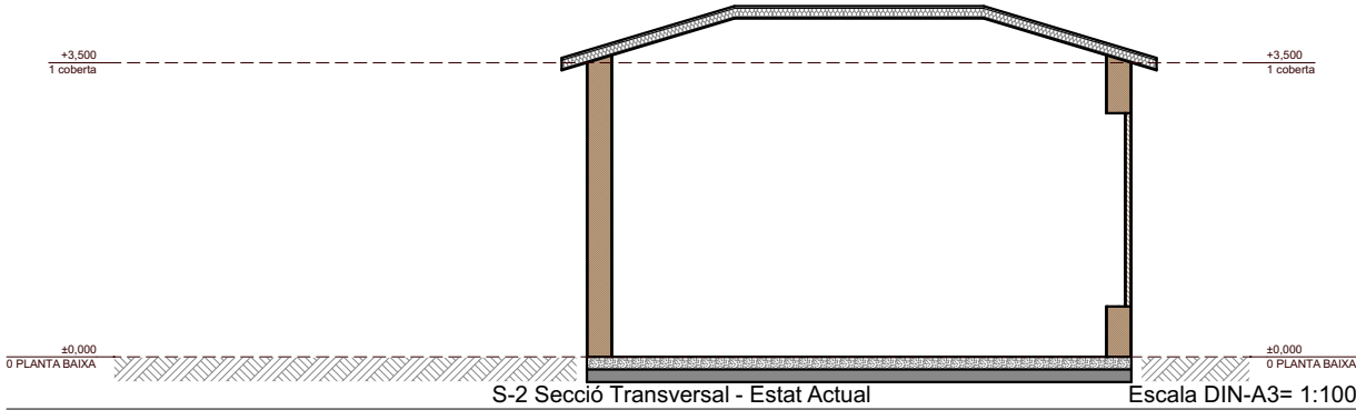
S-2 Secció Transversal - Estat Actual Escala DIN-A3= 1:100
