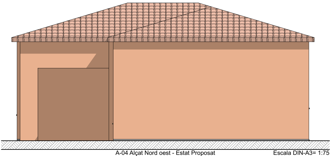
A-04 Alçat Nord oest - Estat Proposat
