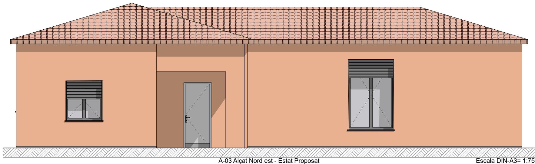
A-03 Alçat Nord est - Estat Proposat
