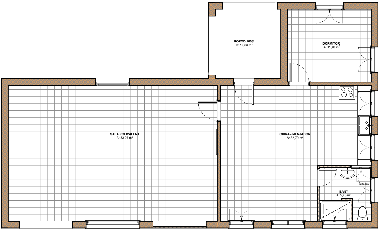
DISTRIBUCIÓ PLANTA BAIXA Estat Actual Escala DIN-A3= 1:100
