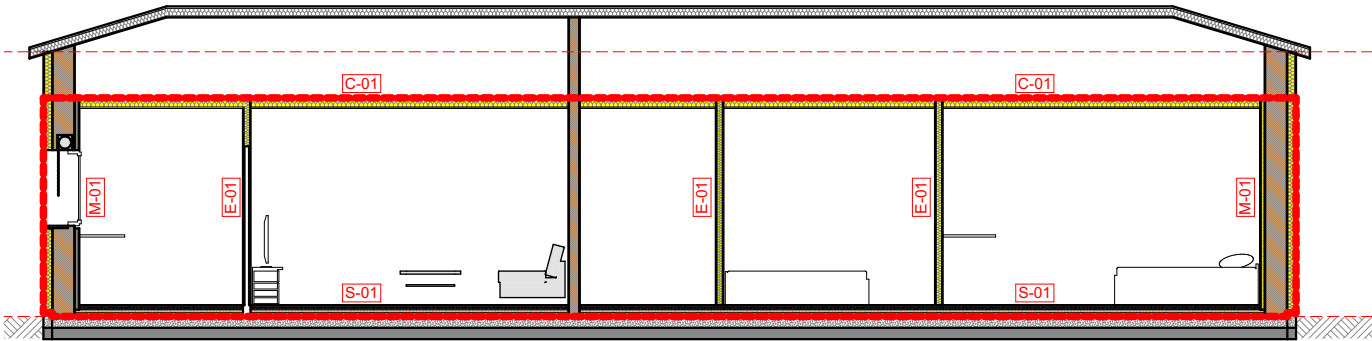
ENVOLVENT TÈRMICA SECCIÓ S-1
