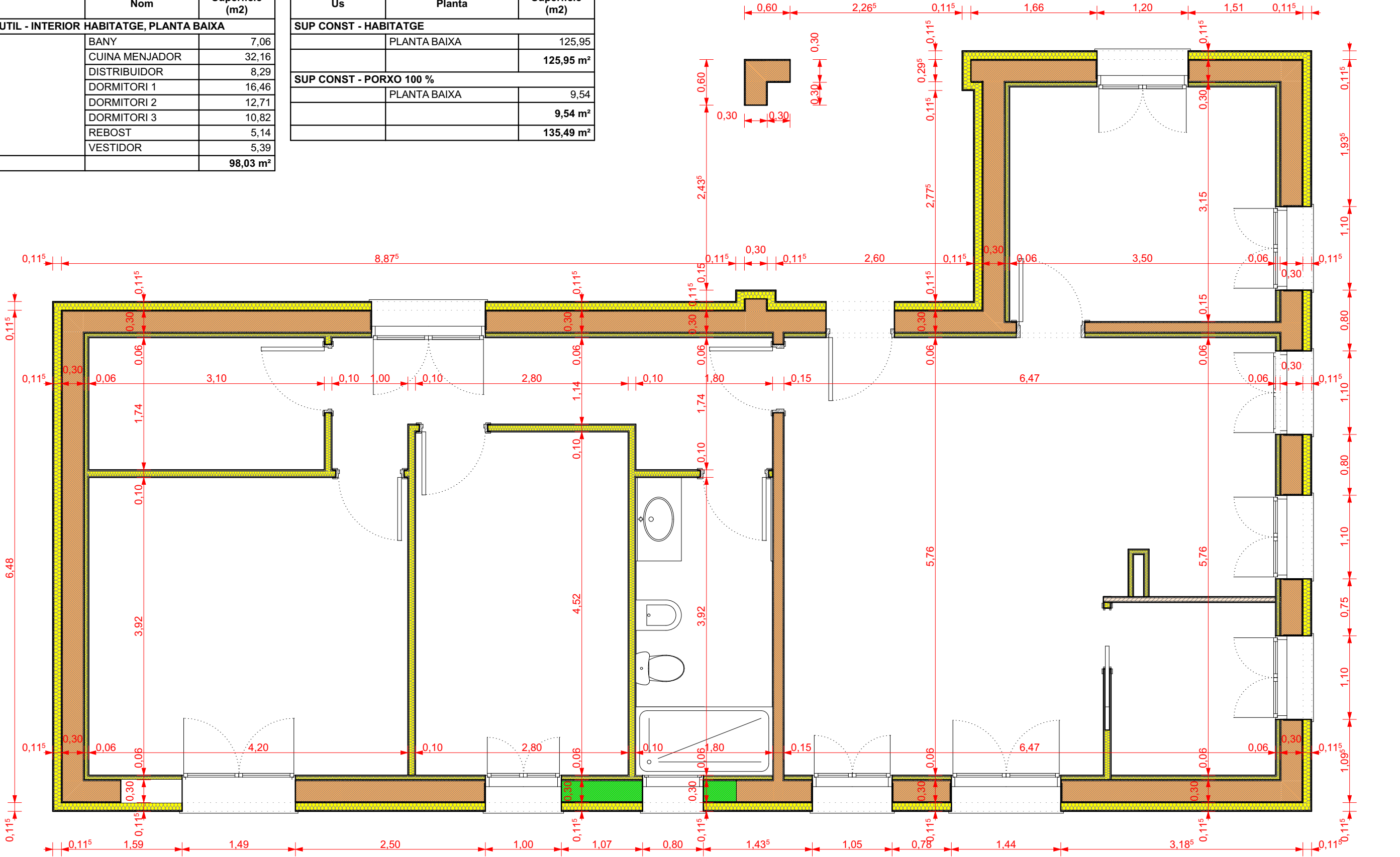
COTES PLANTA BAIXA
