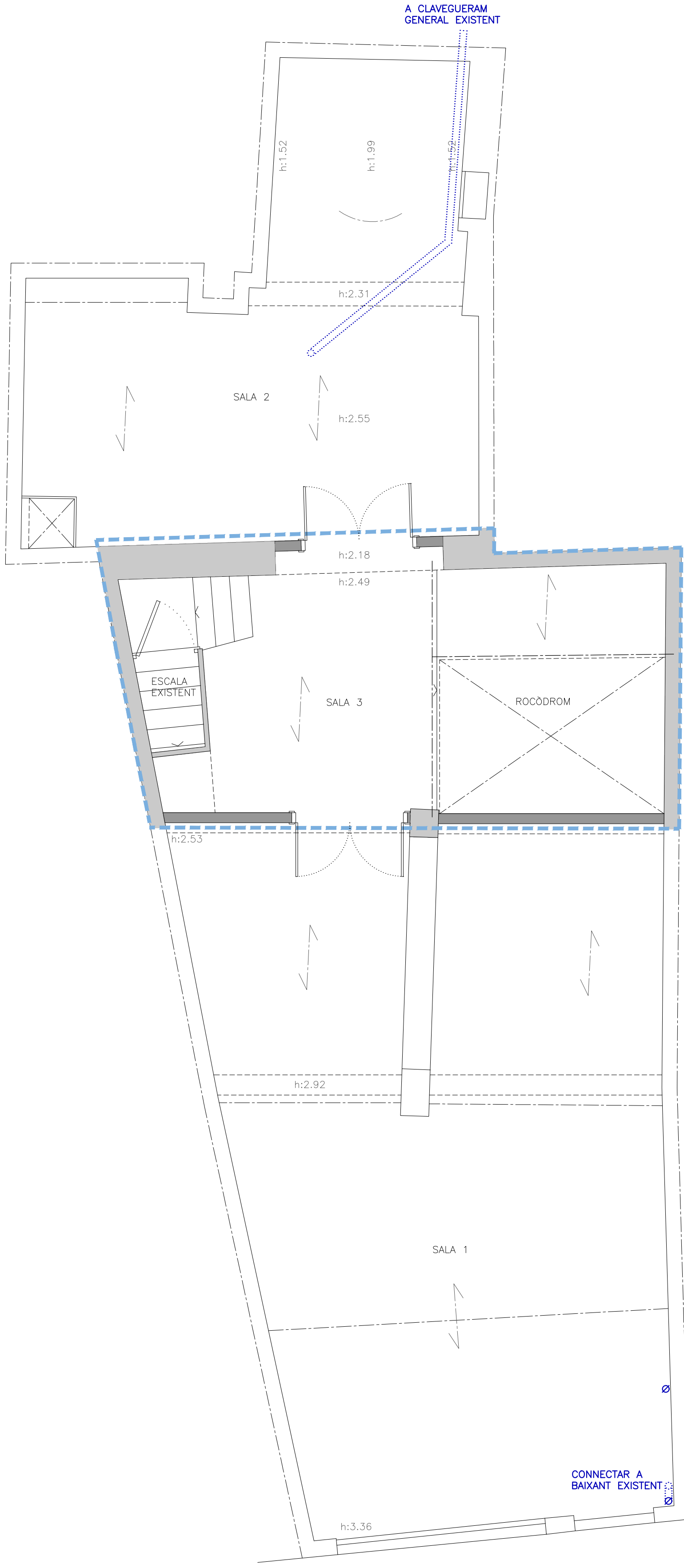
PLANTA SEMISOTERRANI
