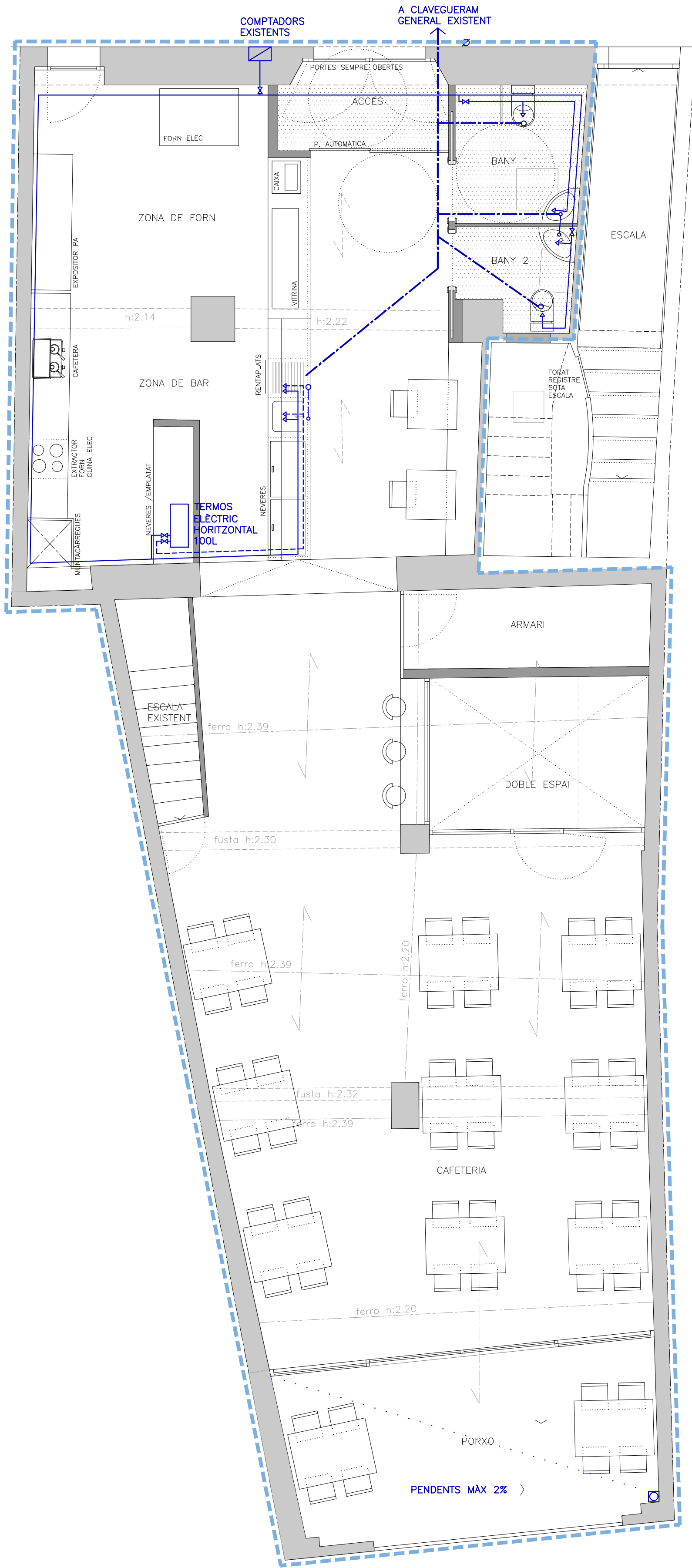
PLANTA BAIXA
