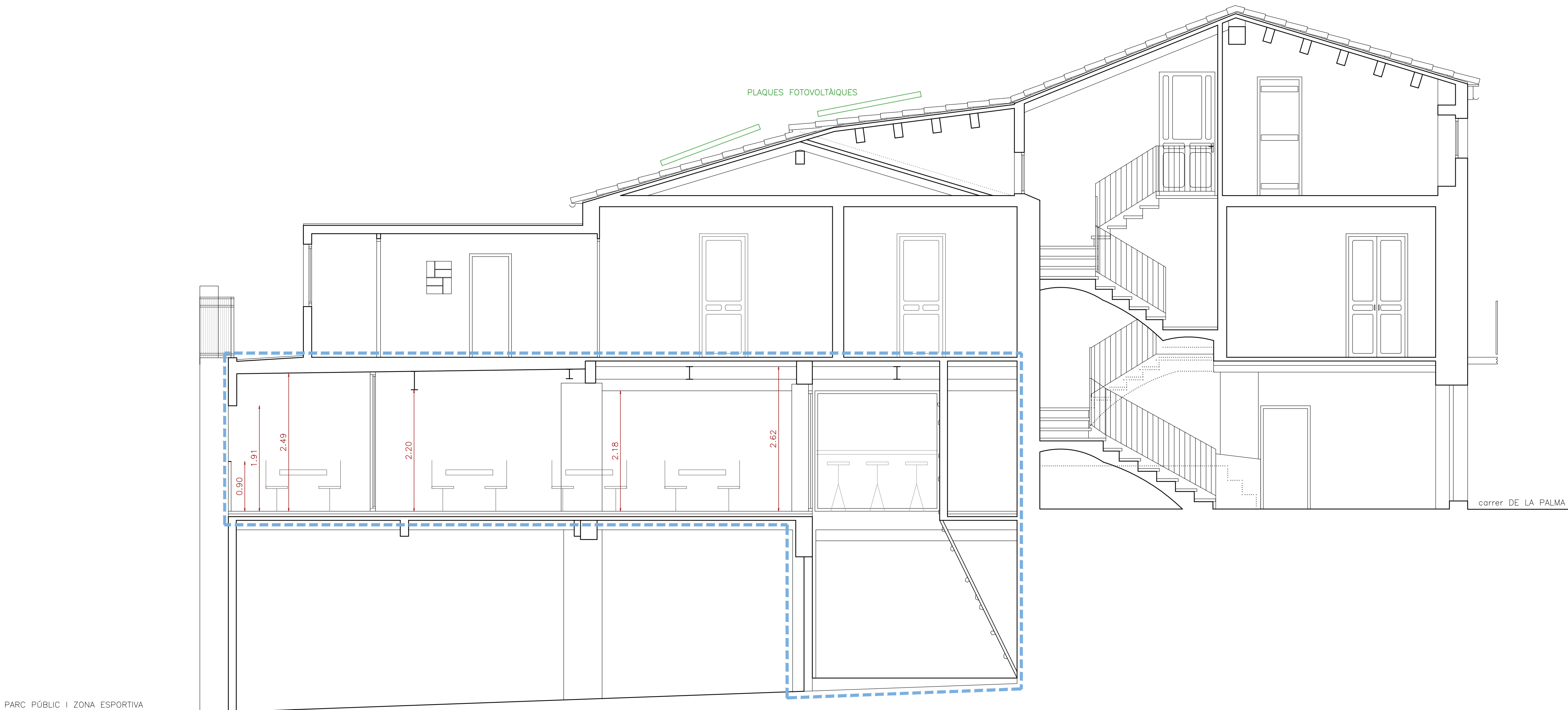
SECCIÓ A
