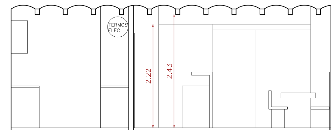
SECCIÓ D
