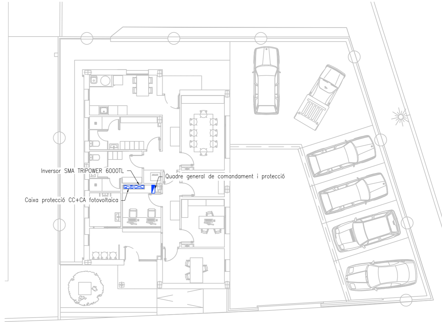
PLANTA BAIXA
