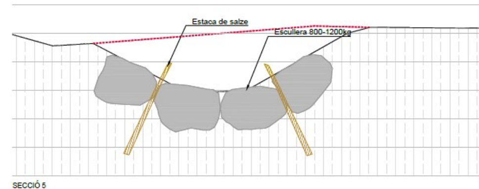
Figura 12. Secció de la protecció d'escullera vegetada a la desembocadura del torrent innominat.
