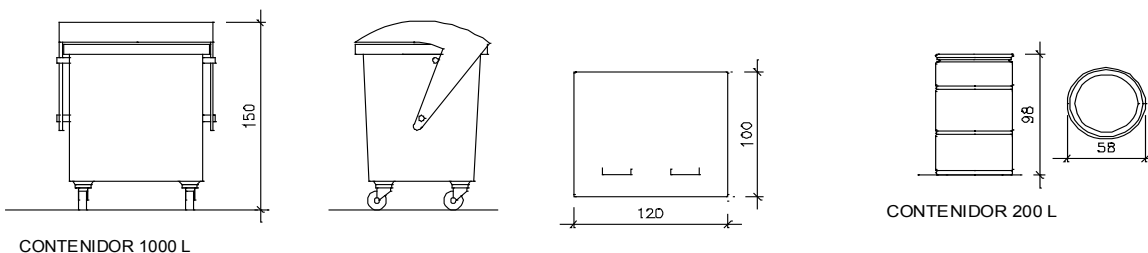
CONTENIDOR 1000 L
