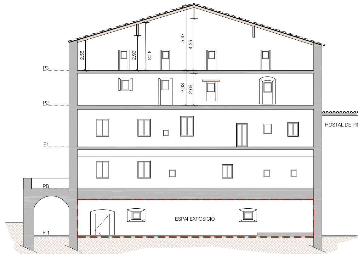
SECCIÓ LONGITUDINAL
