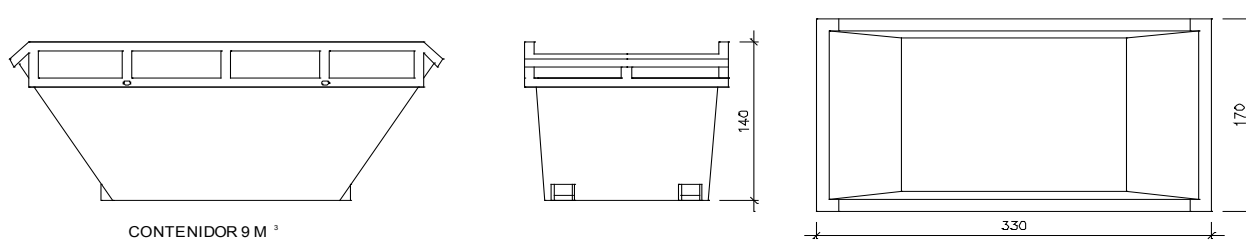
CONTENIDOR 9 M 3
