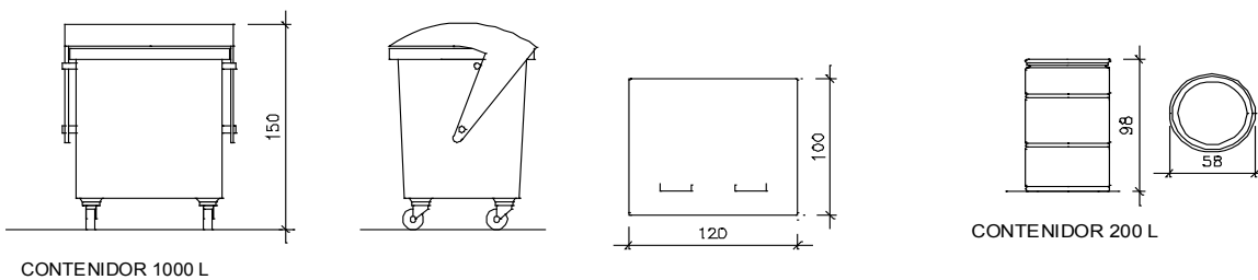
CONTENIDOR 1000 L
