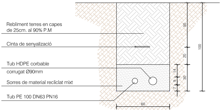
DETALL RASA PER A PAS D'INSTAL·LACIONS (ESCALA 1:25 - COTES EN CM)
