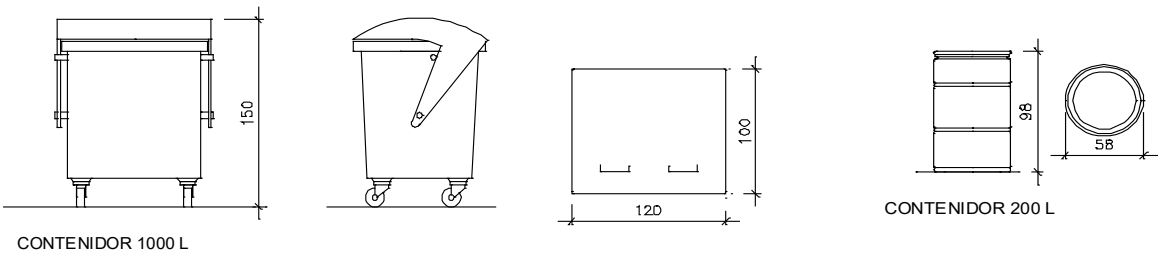
CONTENIDOR 1000 L
