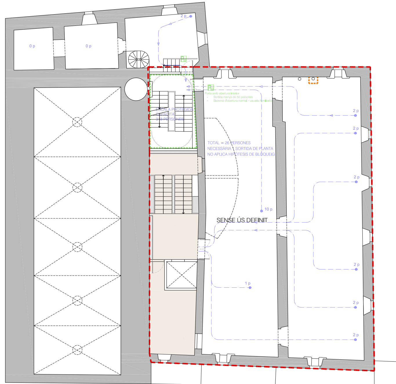
PLANTA 2
