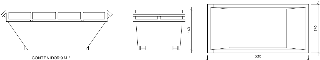
CONTENIDOR 9 M 3
