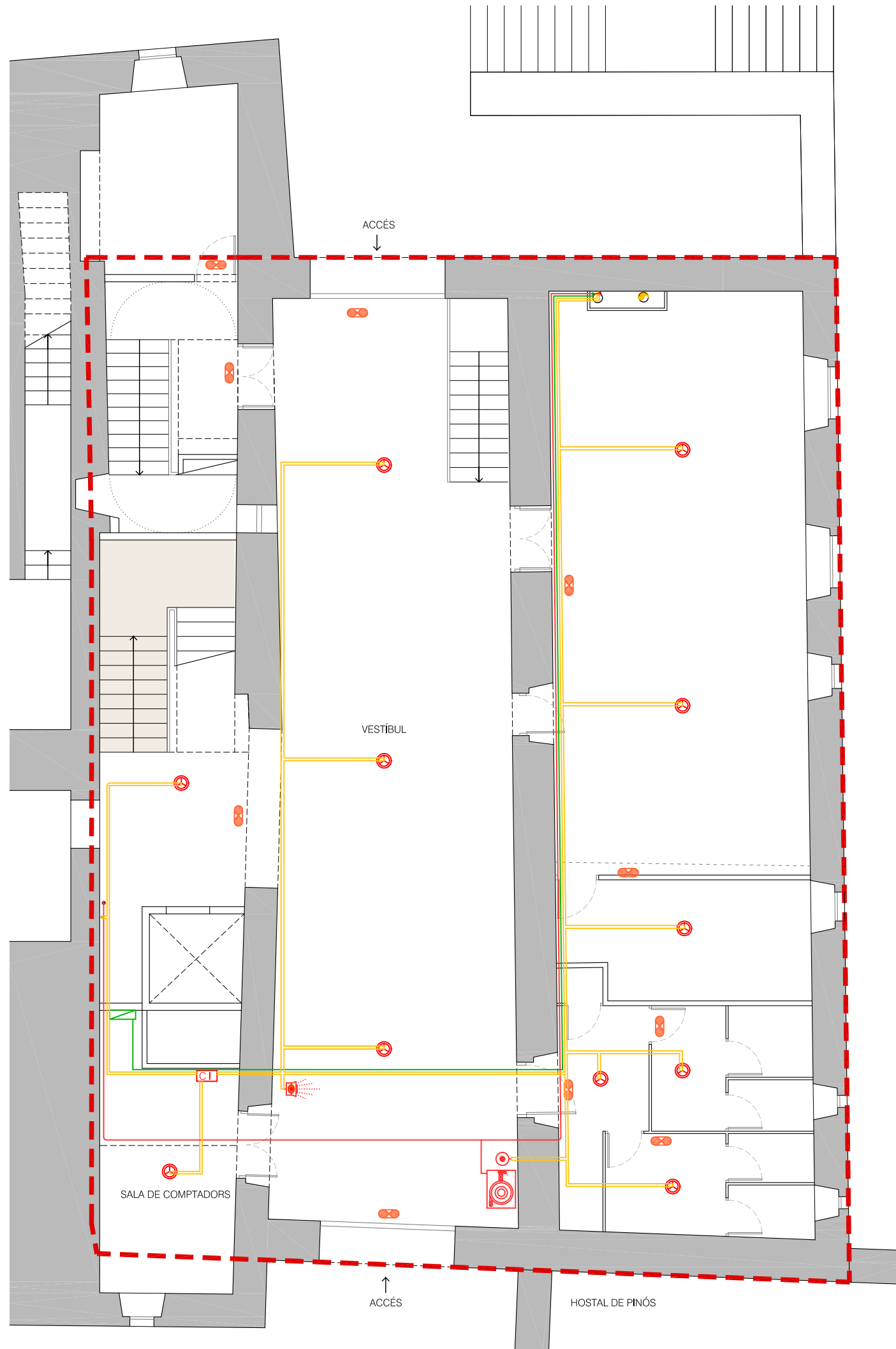
PLANTA BAIXA
