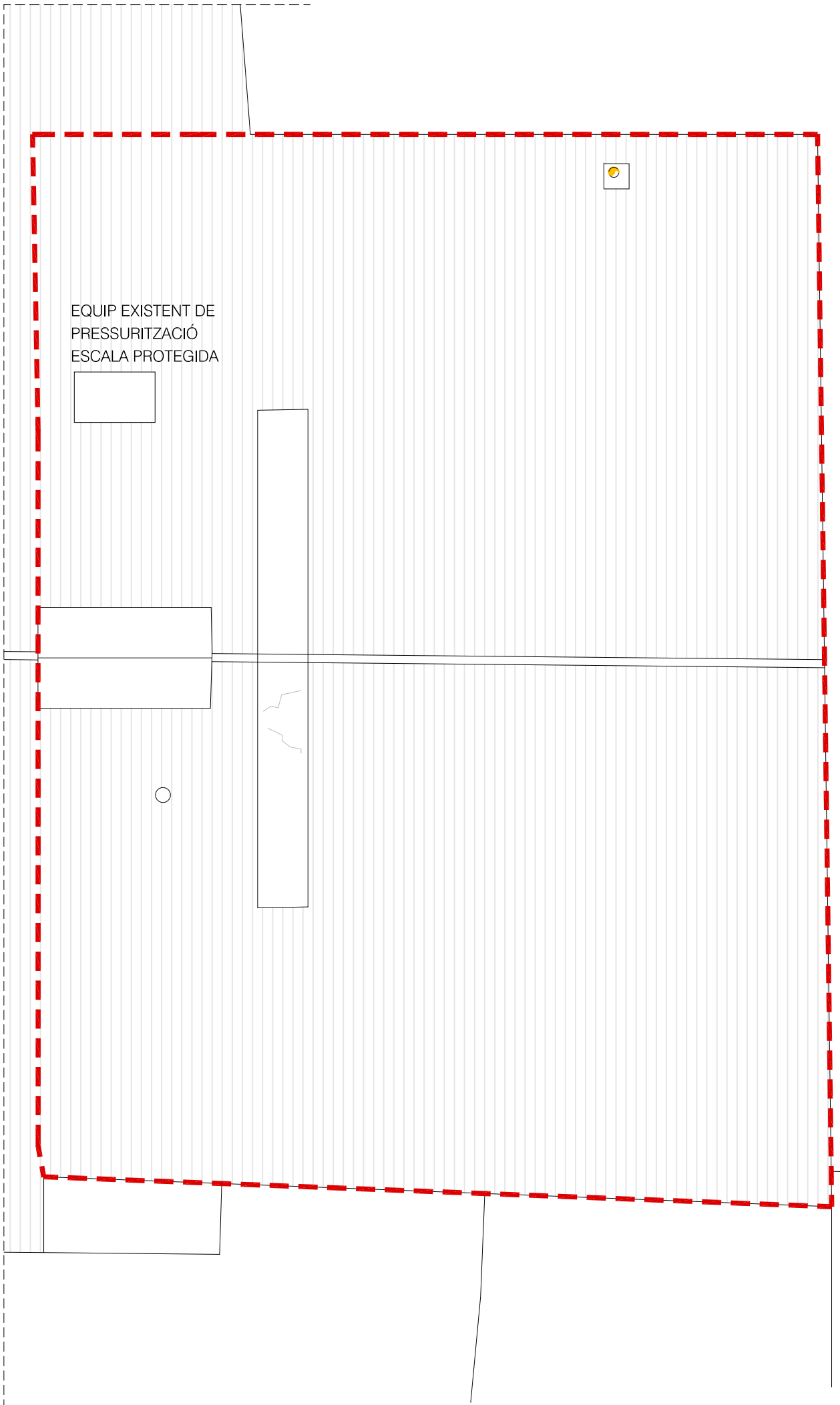
PLANTA COBERTA
