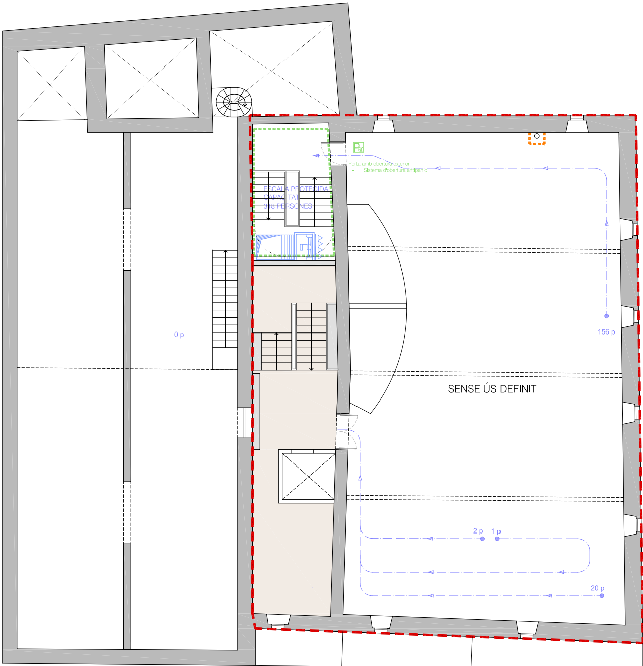
PLANTA 3
