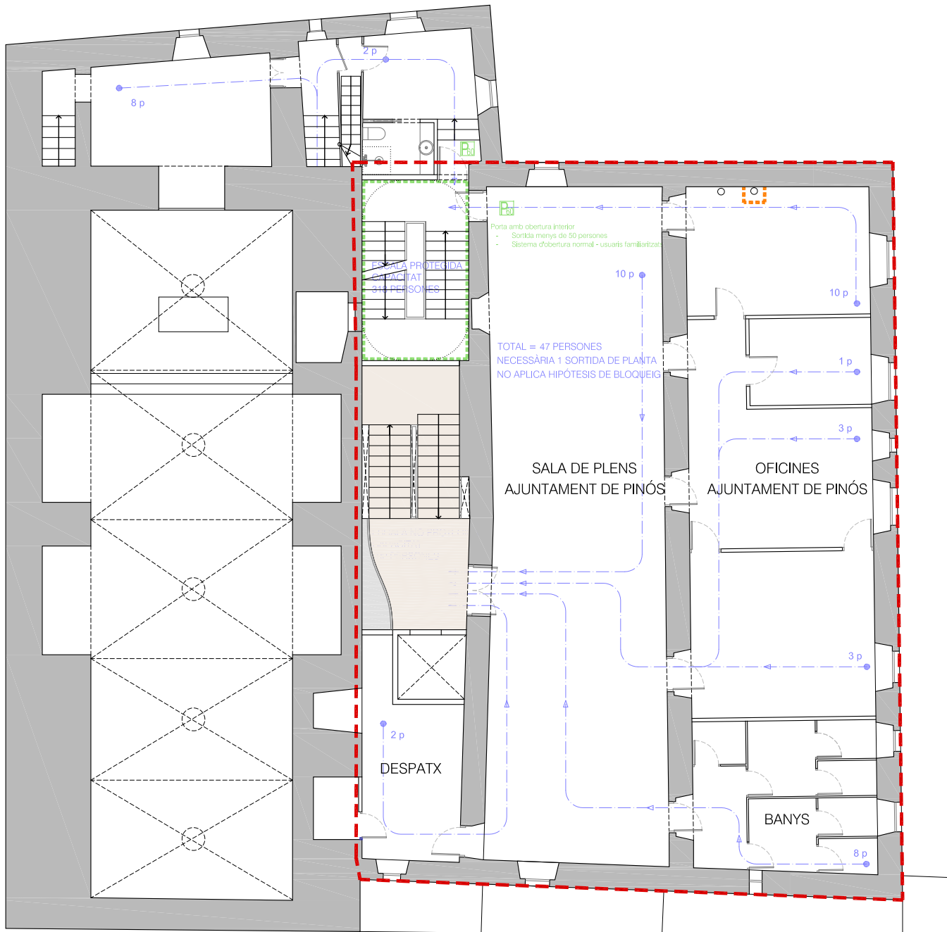
PLANTA 1
