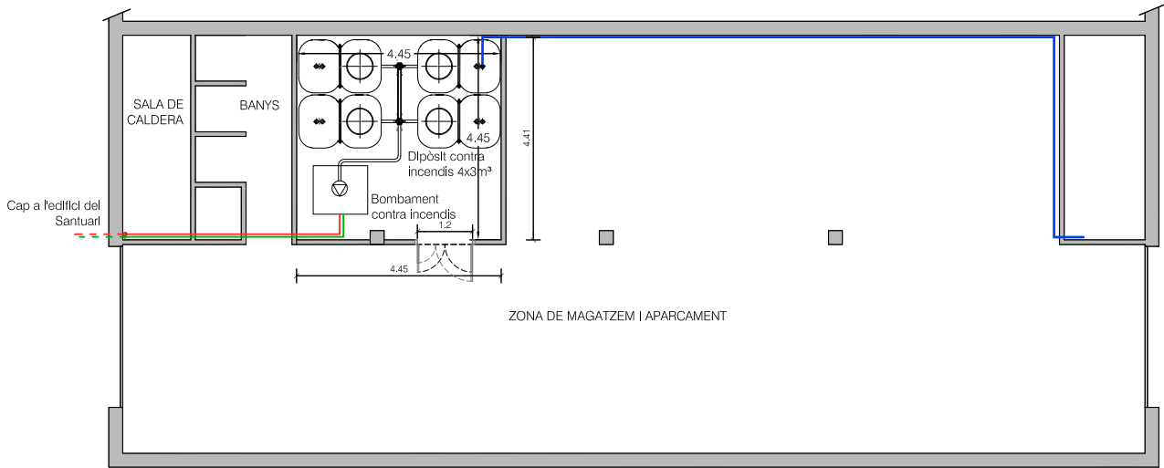
PLANTA SEMISOTERRADA - LOCAL SOCIAL Localització dipòsits aigua contra incendis Escala 1:150
