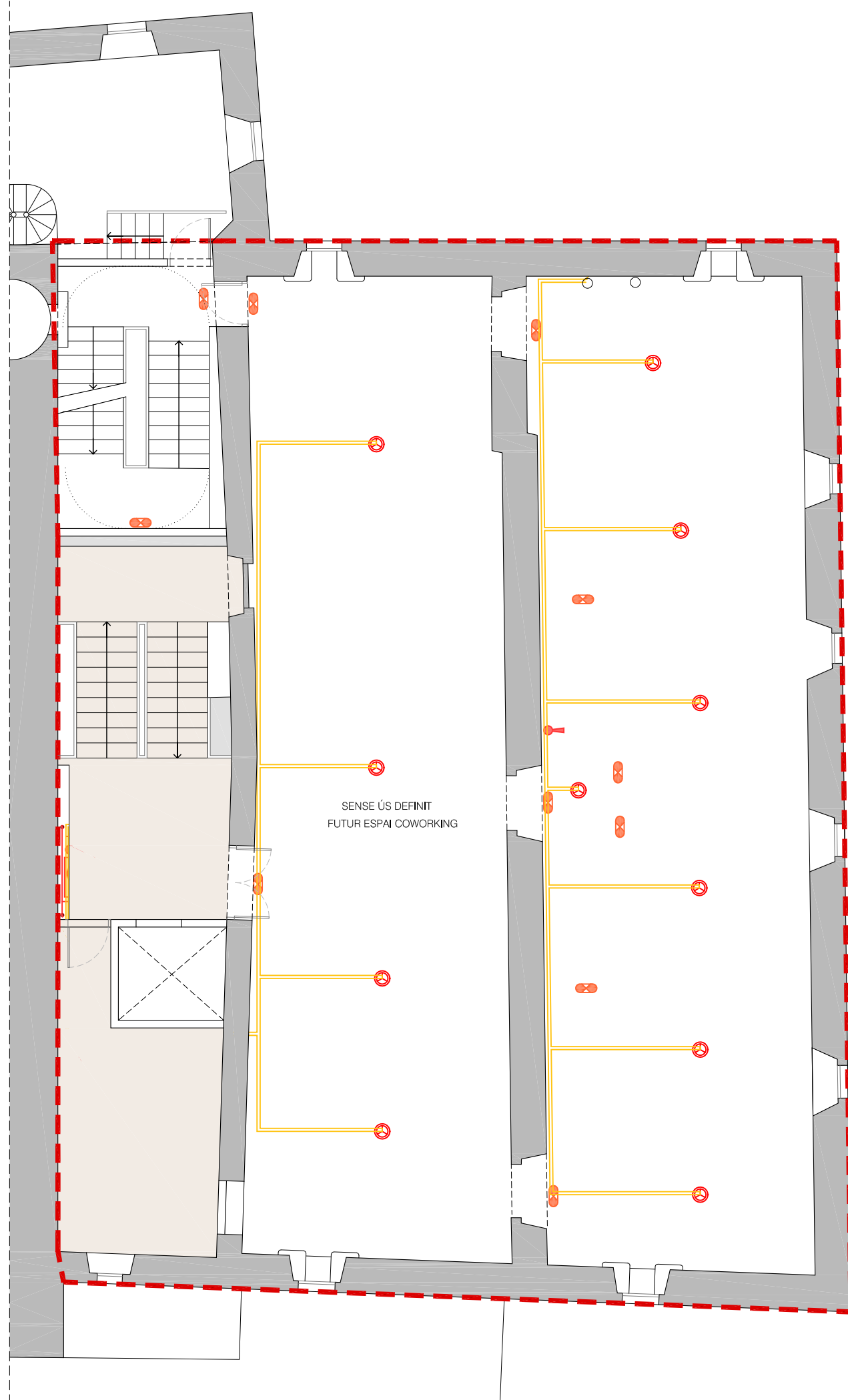
PLANTA 2
