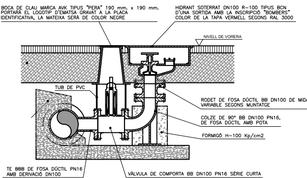
HIDRANT SOTERRAT TIPUS
