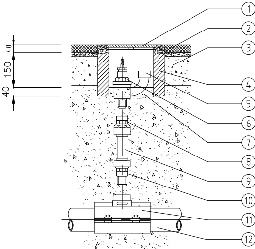
INSTAL·LACIÓ BOCA DE REC
