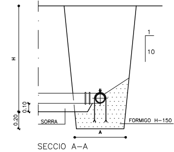
SECCIO A-A
