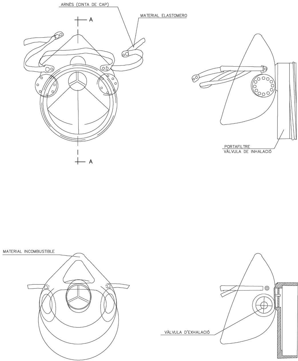
SECCIÓ A-A
