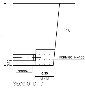
SECCIO D-D
