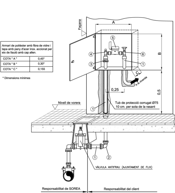
ESCOMESA D'AIGUA
