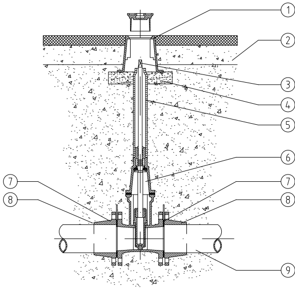
INSTAL·LACIÓ VÀLVULA PER CANONADES DE PEAD I FIBROCIMENT
