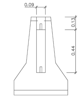
ALÇAT TRANSVERSAL
