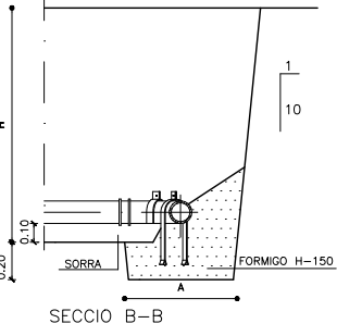
SECCIO B-B
