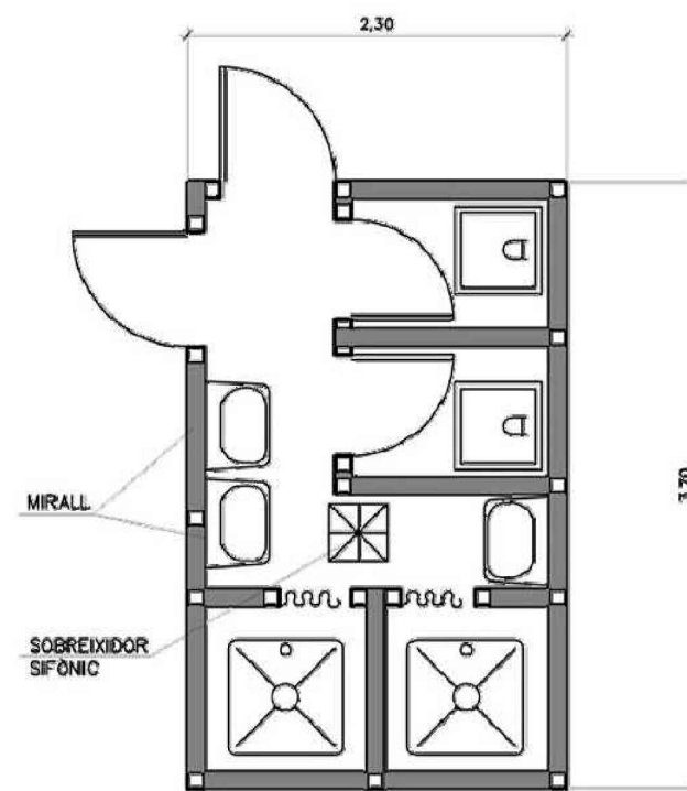
SERVEIS
