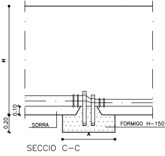
SECCIO C-C
