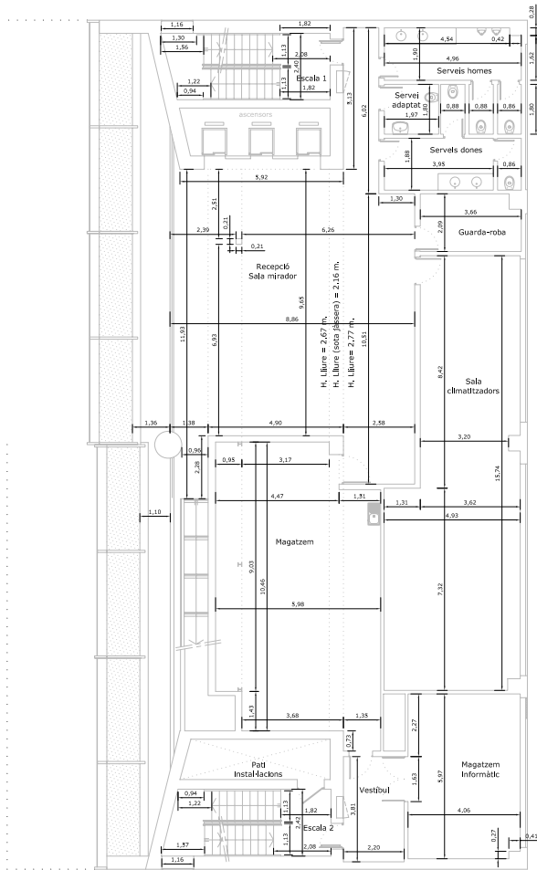
P.QUARTA
