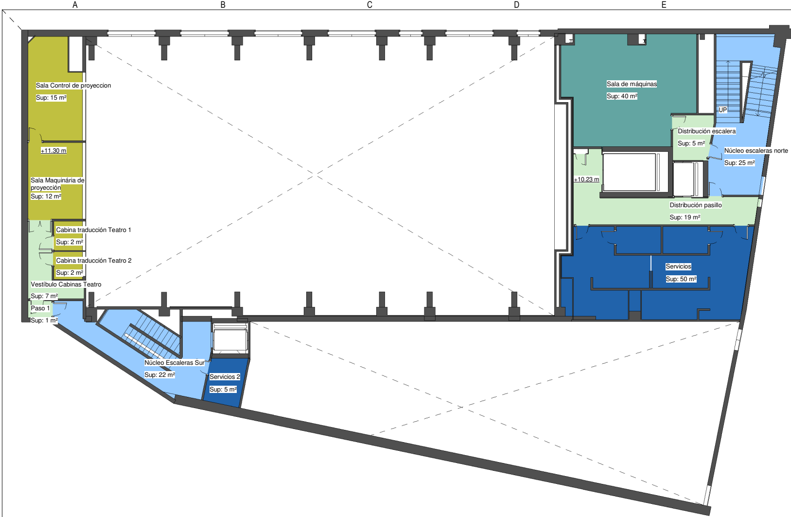
PLANTA SEGUNDA \ 1 : 100
