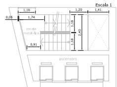
P.ENTREPLANTA Escala 1
