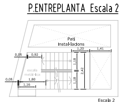
P.ENTREPLANTA Escala 2
