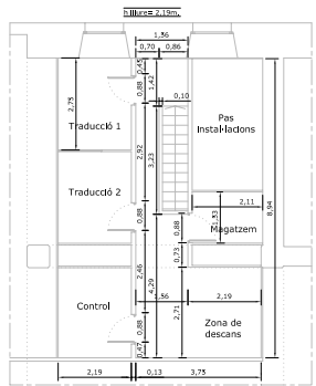
P.ENTRESOLAT
