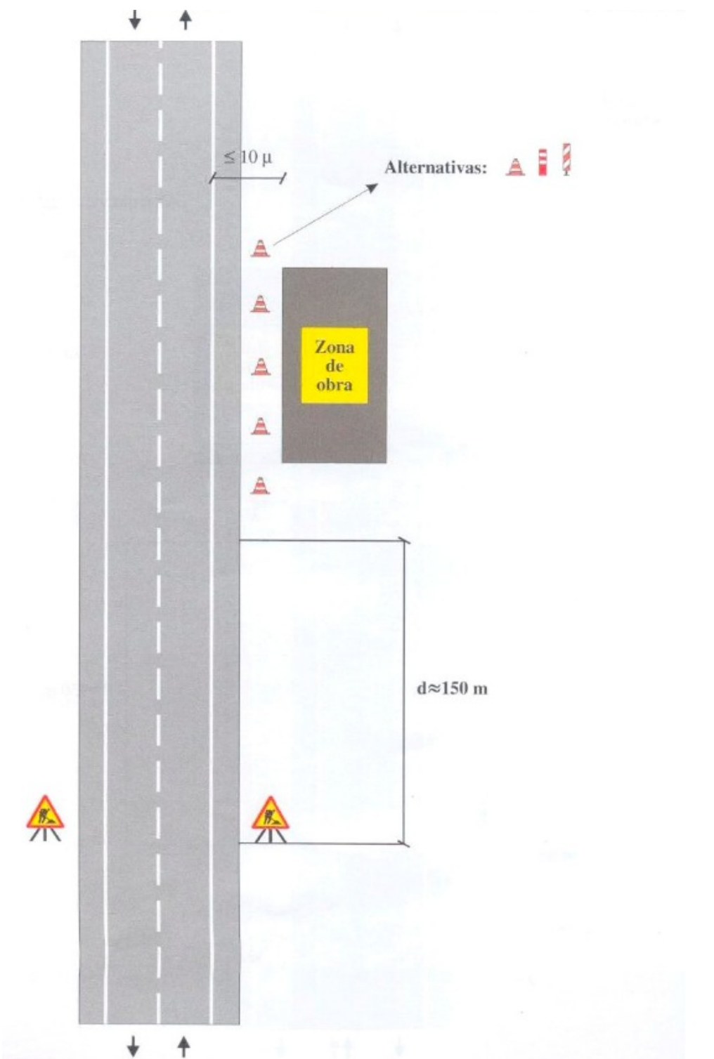
DETALL VIA DE DOBLE SENTIT DE CIRCULACIÓ CALÇADA ÚNICA AMB 2 CARRILS. ZONA DE L'OBRA EXTERIOR A LA PLATAFORMA
