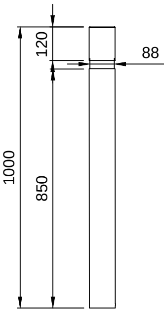
DETALL E 1/20 (A3) PILONA TIPUS BARCELONA 92 C-43
