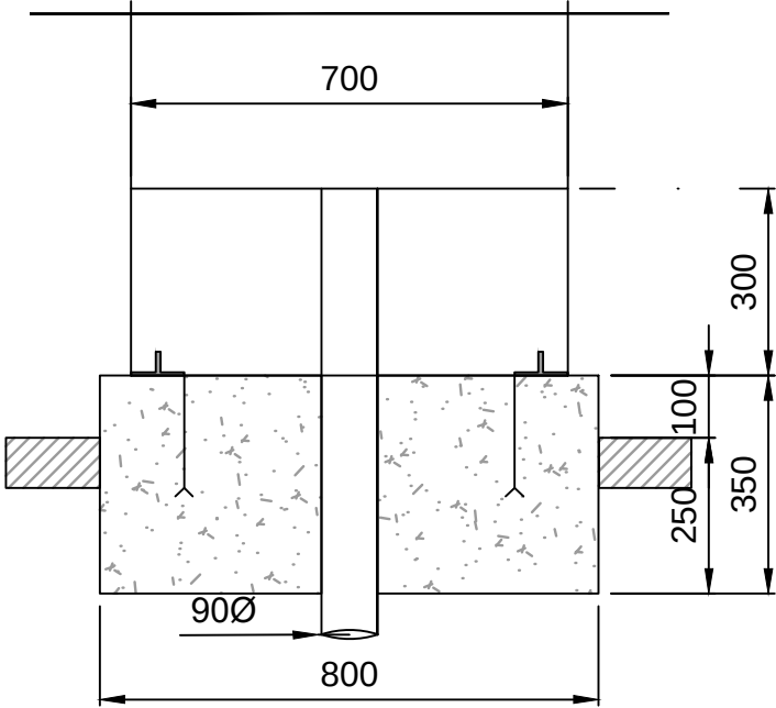
DETALL 1/20 (A3) BASAMENT DE L'EdRR
