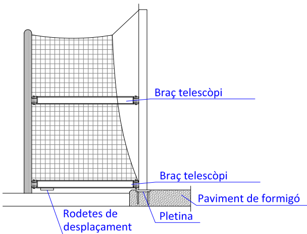
PORTERIA DE FUTBOL 7 LATERAL
