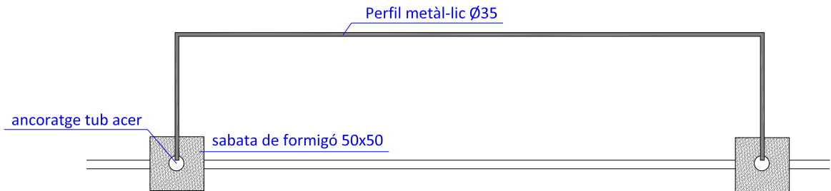
PORTERIA DE FUTBOL 11 PLANTA
