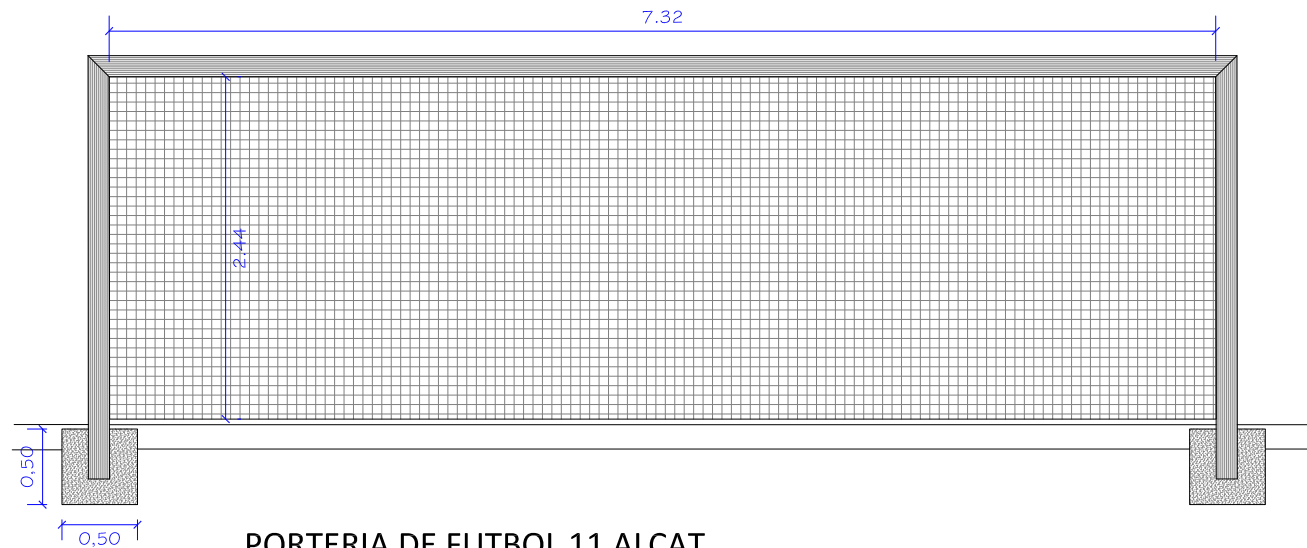
PORTERIA DE FUTBOL 11 ALÇAT
