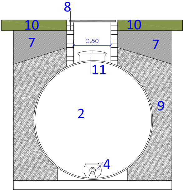
SECCIÓ TRANSVERSAL
