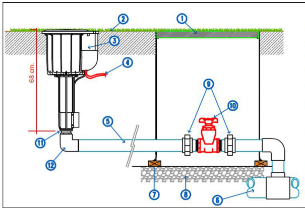
DETALL ASPERSOR
