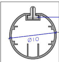
DETALL PERFIL D'ALUMINI DE PALS I TRAVESSER
