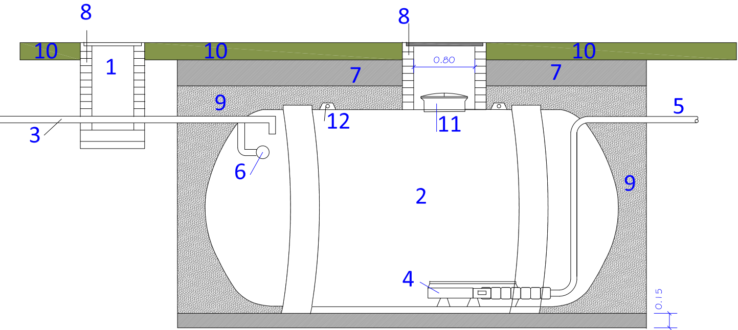
SECCIÓ LONGITUDINAL
