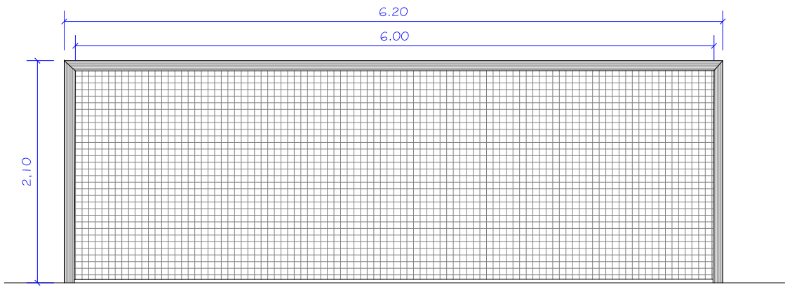
PORTERIA DE FUTBOL 7 ALÇAT
