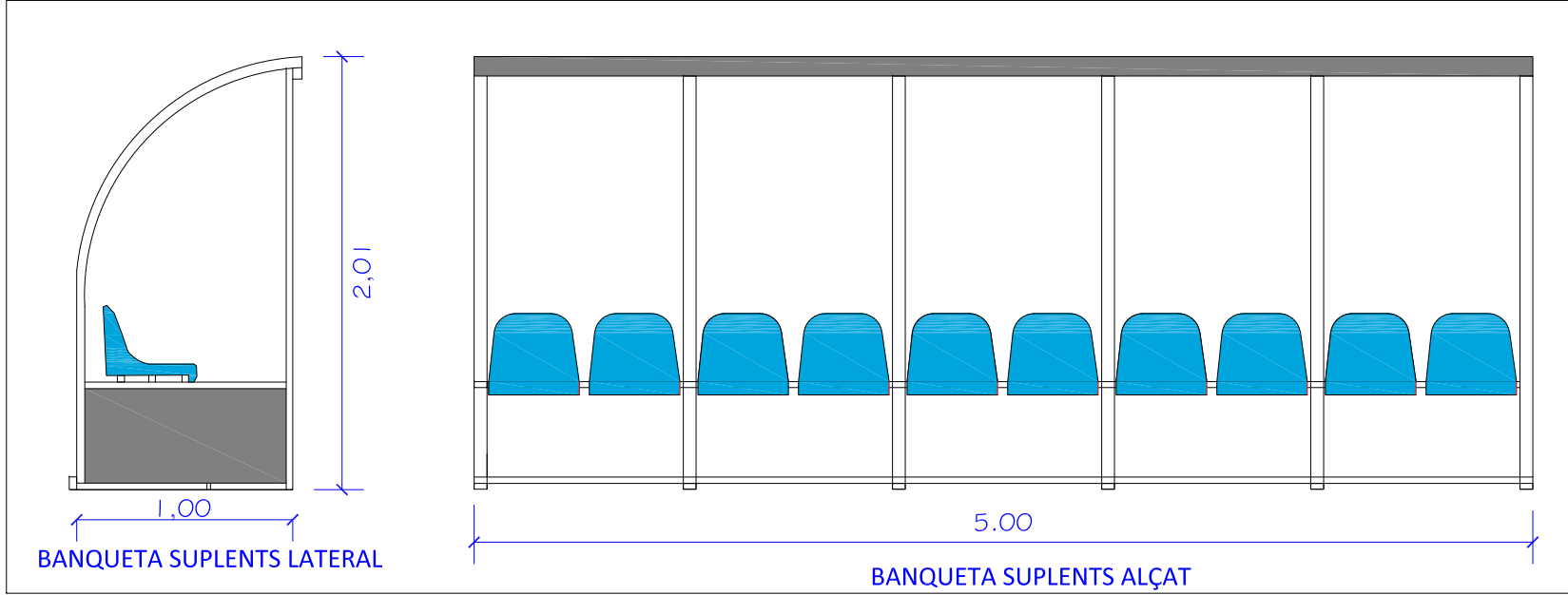
DETALL BANQUETES ESC 1/30
