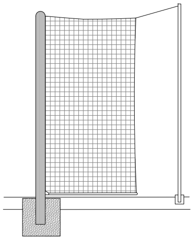
PROTERIA DE FUTBOL 11 LATERAL
