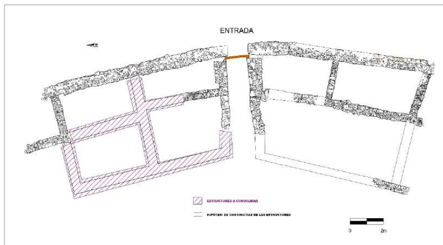
Fig. 54: Senyalització dels murs que s'hauran de consolidar
