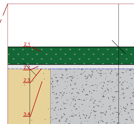
Detall D2 gespa E 1/5
