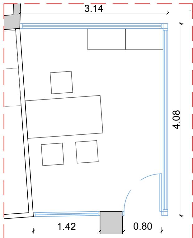
Planta acotada
