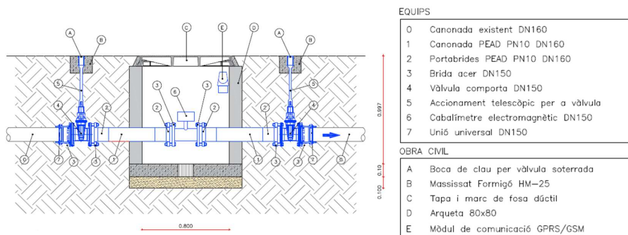
Figura 4. Detall arqueta cabalímetre. Obra civil i equips.
