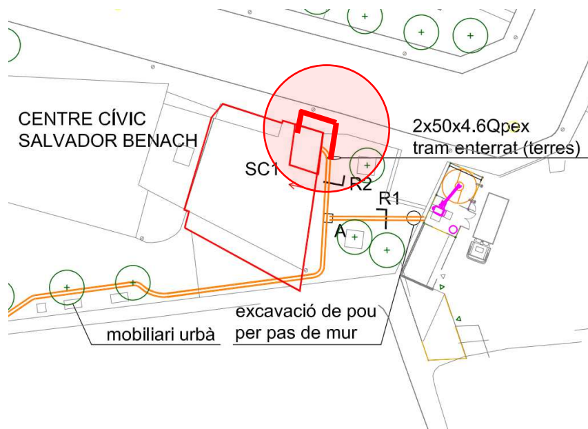
Planta millora del traçat accés sala de calderes centre cívic per evitar pas per cuina
