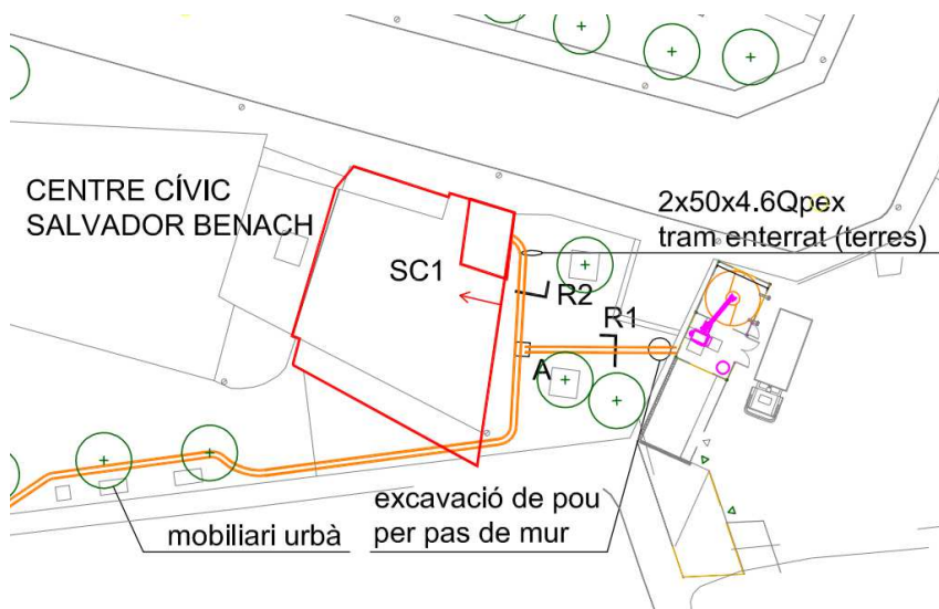
Planta del traçat millora accés sala de calderes centre cívica per evitar pas per cuina.
