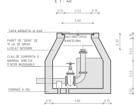
SECCIÓ E 1 : 40
