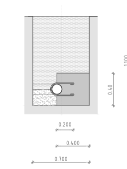
SECCIÓ
