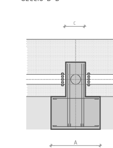
SECCIÓ B-B
