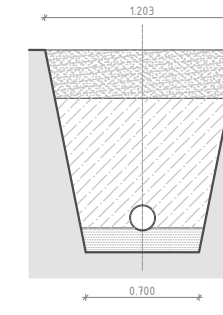
CONDUCCIÓ PROTEGIDA
