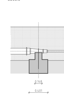
SECCIÓ
