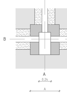
SECCIÓ B-B
