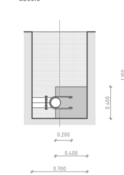
SECCIÓ
