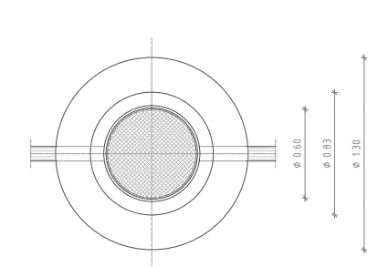
SECCIÓ E 1 : 40
