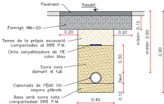
Figura 5. Detall rasa en paviment existent
