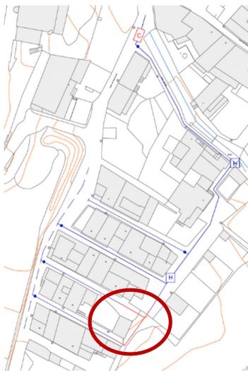
Figura 3. Mallat xarxa PEAD Ø90mm
