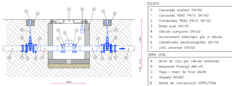
Figura 2. Detall arqueta cabalímetre. Obra civil i equips.
