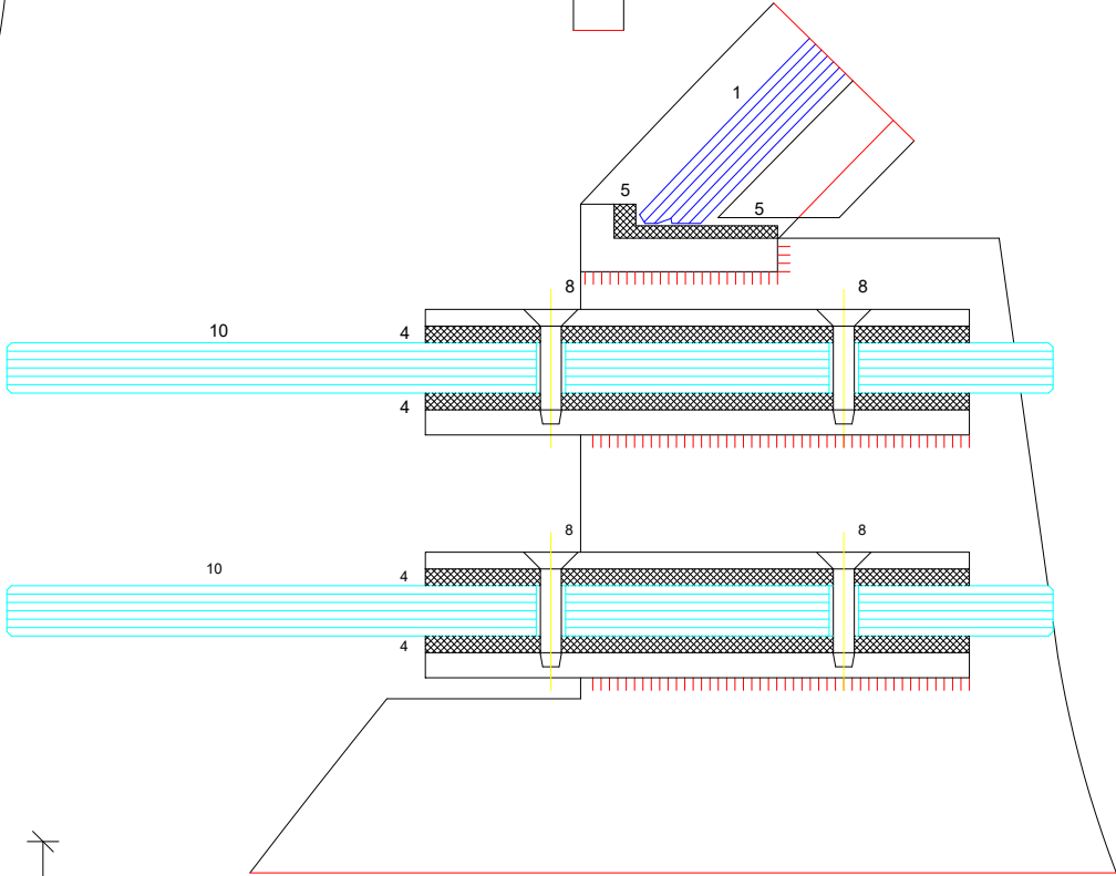
SECCIÓ A
