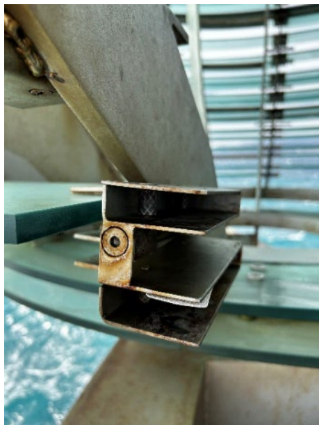
Xarnera tipus i xarnera porta d'accés a l'esfera
