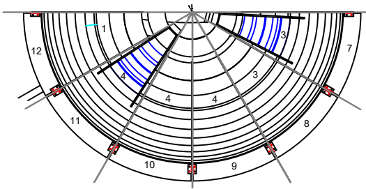
SECCIÓ HORIZONTAL 7-12
