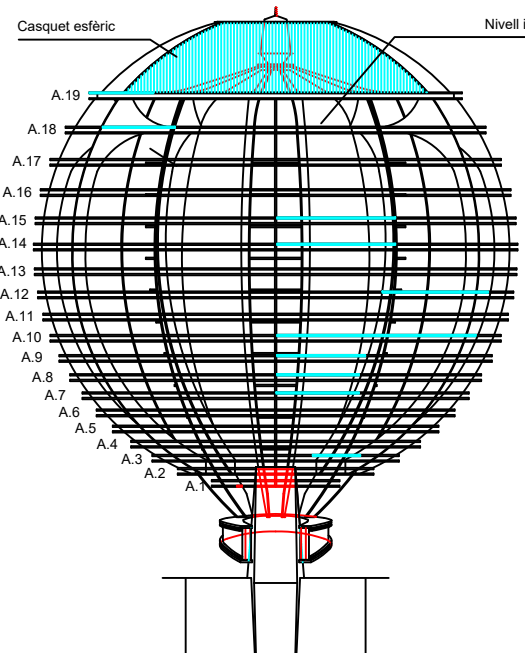
ALÇAT FRONTAL
