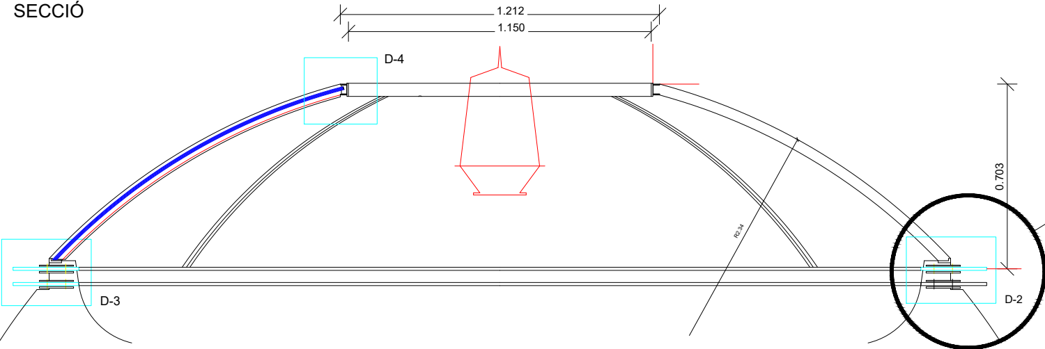
SECCIÓ
