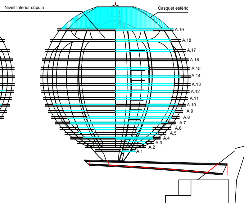
ALÇAT LATERAL
