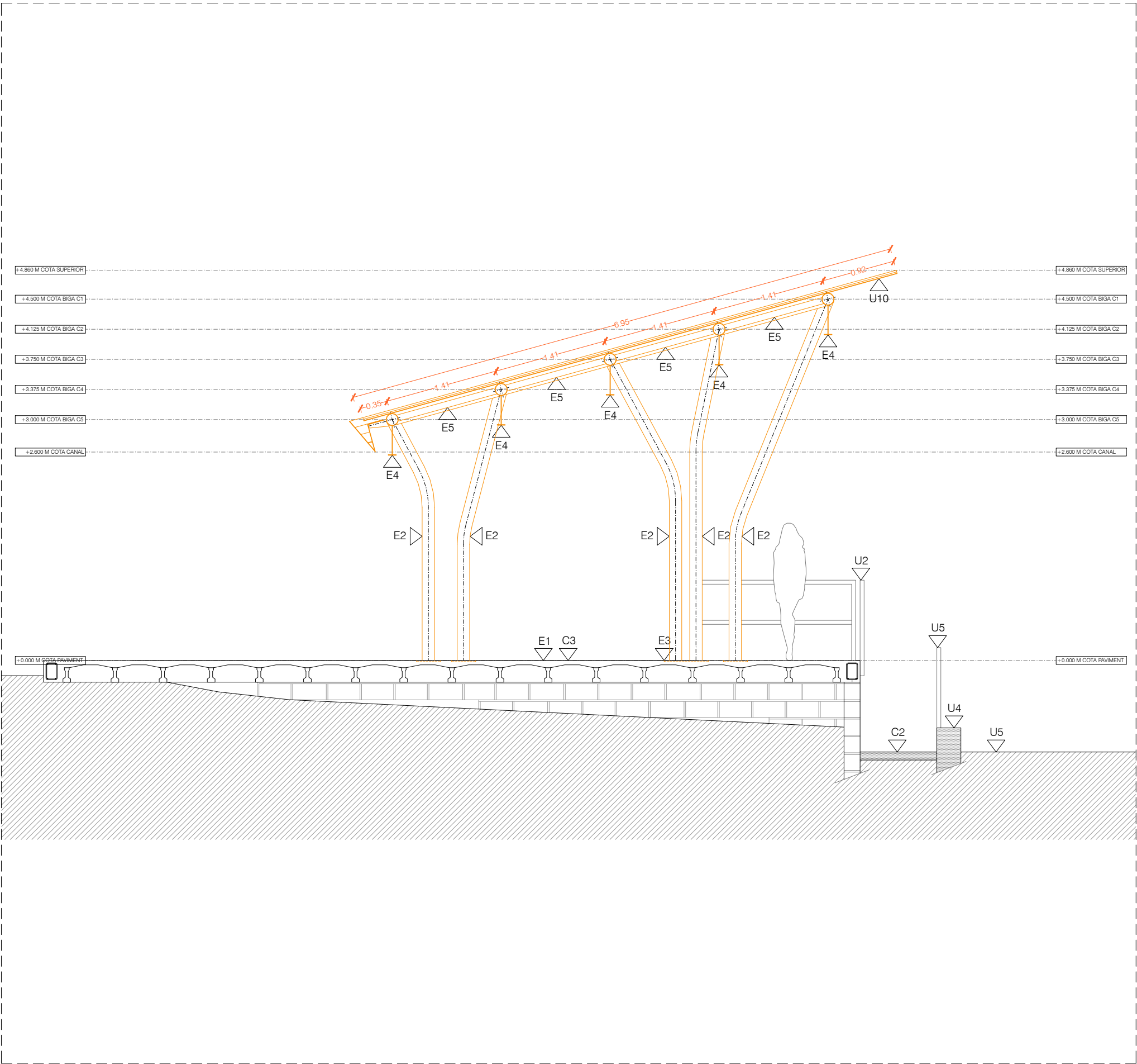
SECCIÓ LONGITUDINAL ST1
