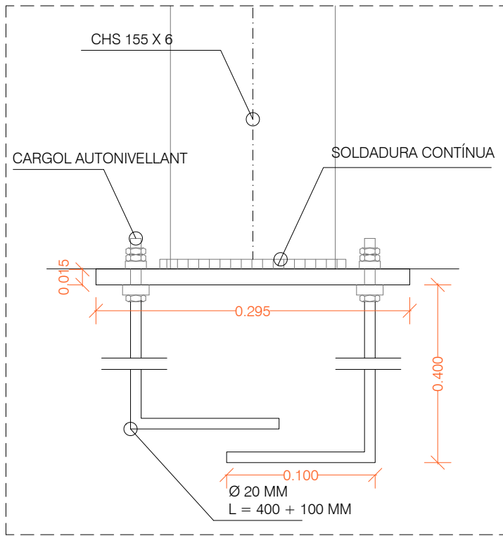
ANCORATGE PLATINA
