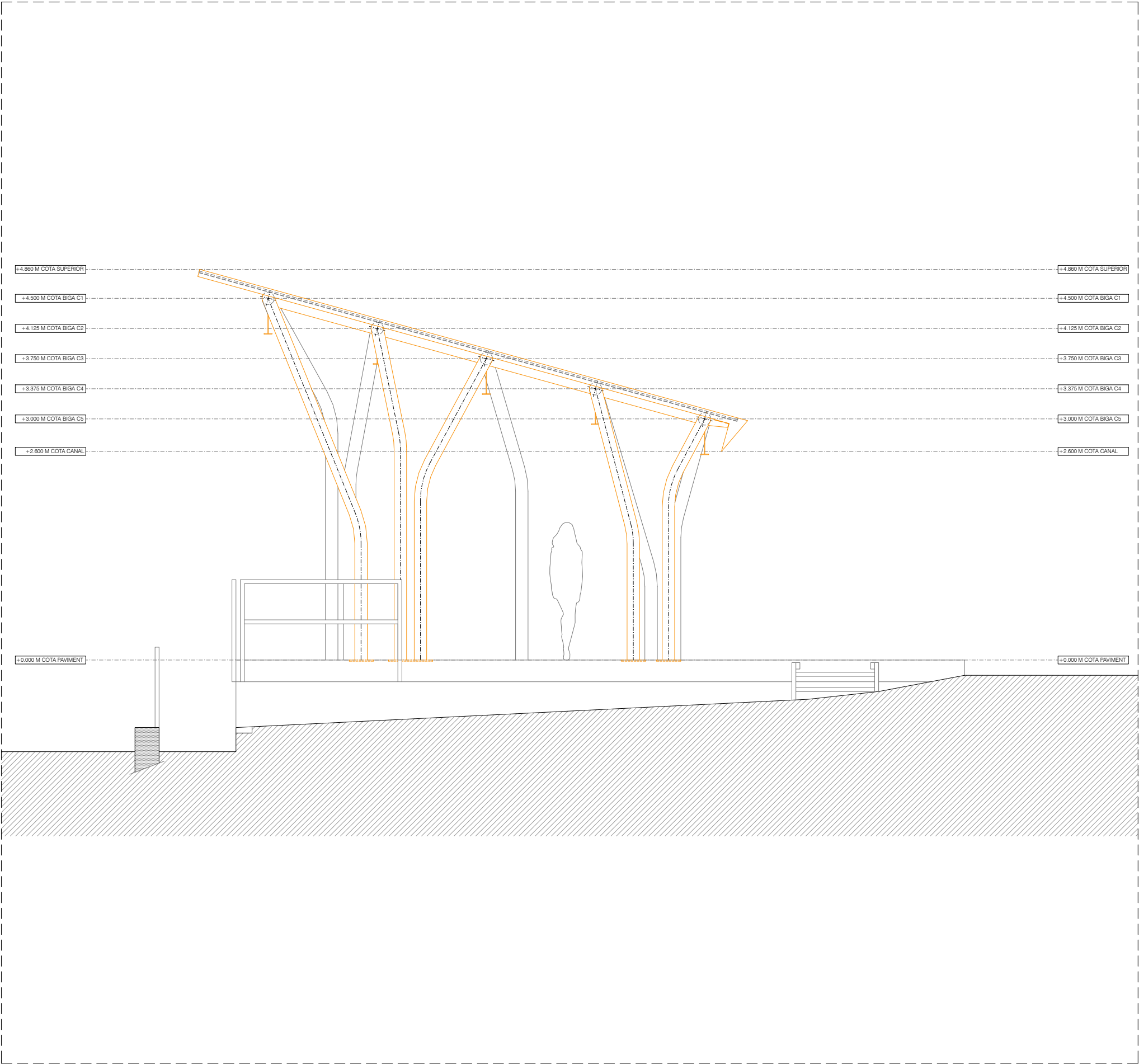
ALÇAT SUD-OEST
