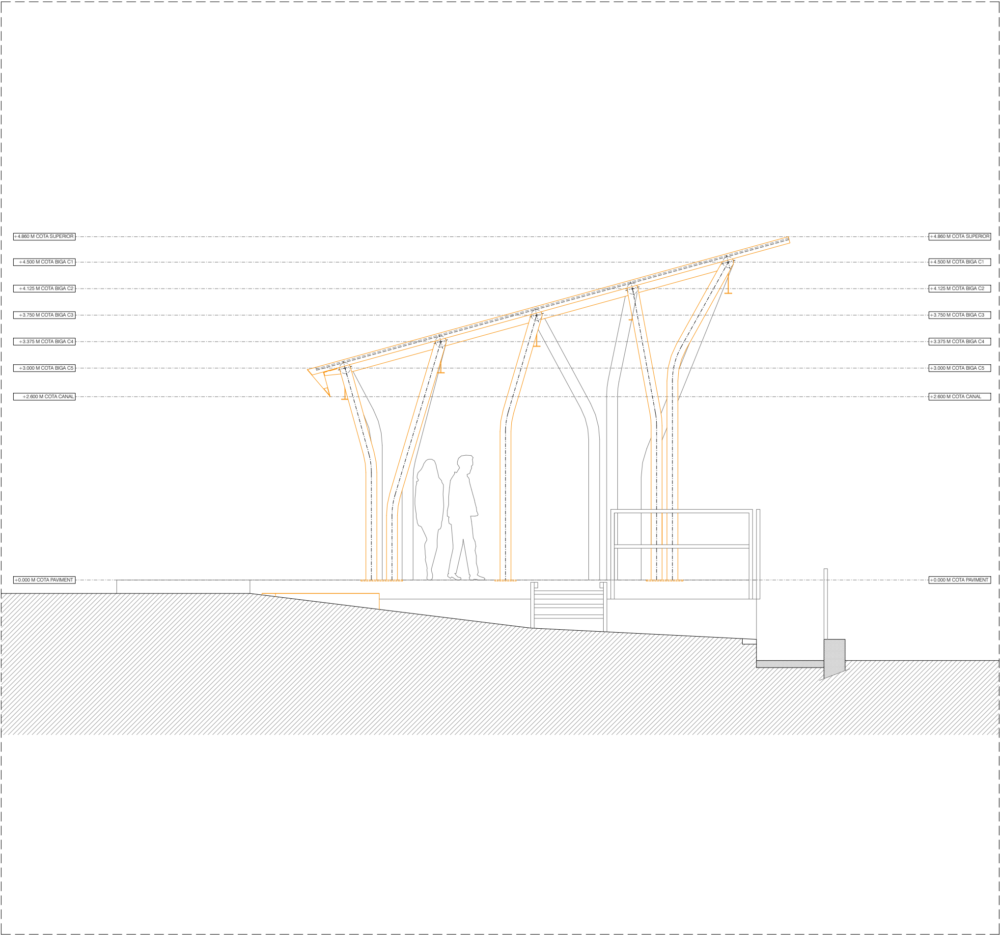
ALÇAT NORD-EST
