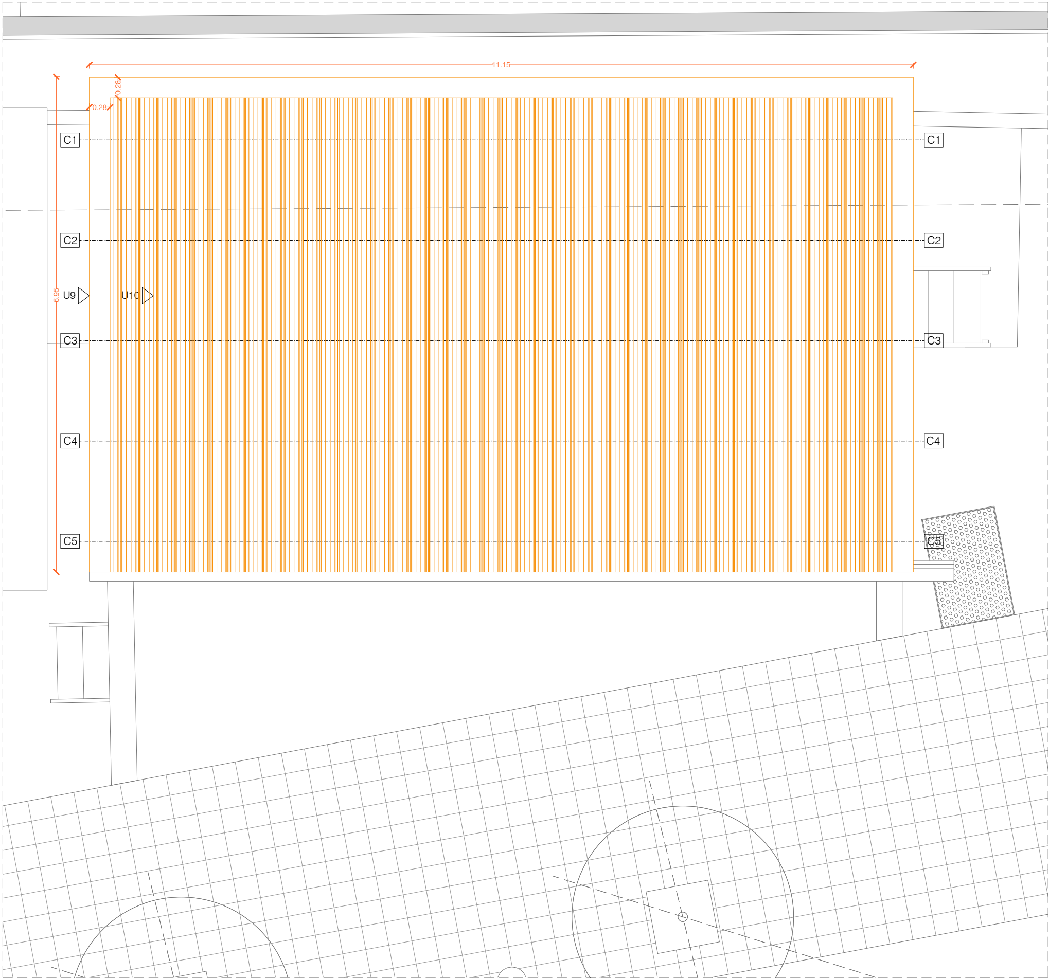
PLANTA COBERTA
