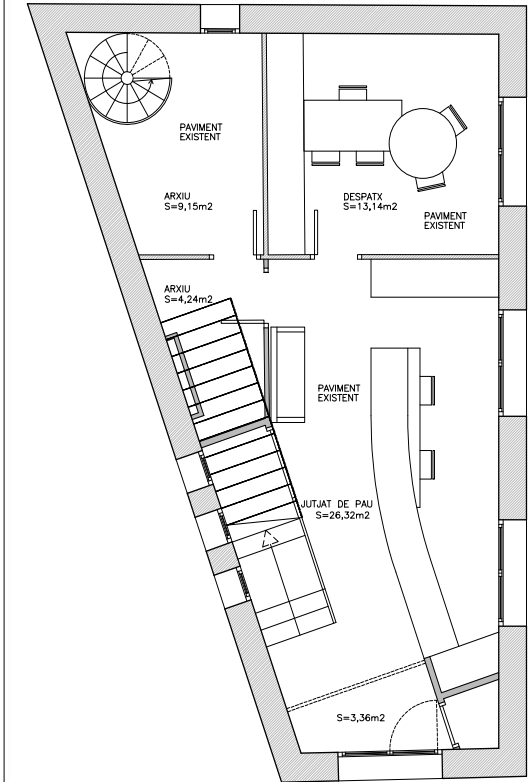
PLANTA BAIXA SUPERFICIE CONSTRUÏDA P.B 74,02m2
