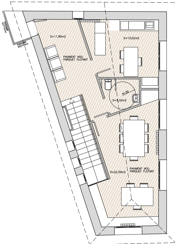
PLANTA PRIMERA SUPERFICIE CONSTRUÏDA P.1 74,02m2
