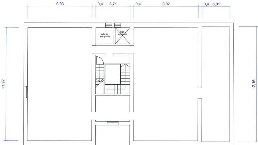
PLANTA GOLFES ESTAT ACTUAL
