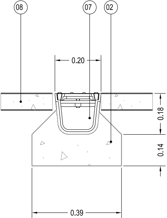
SECCIÓ
