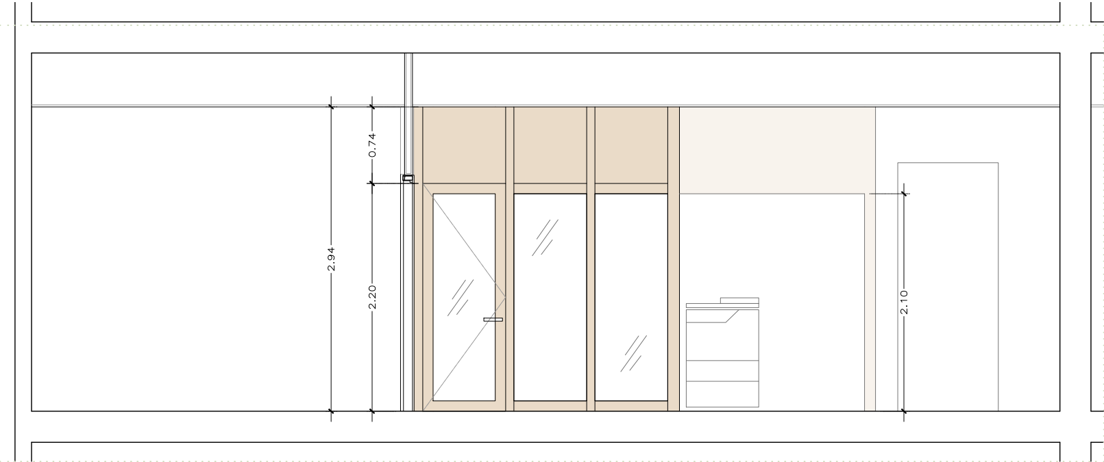
S1_SECCIÓ ACOTACIÓ
