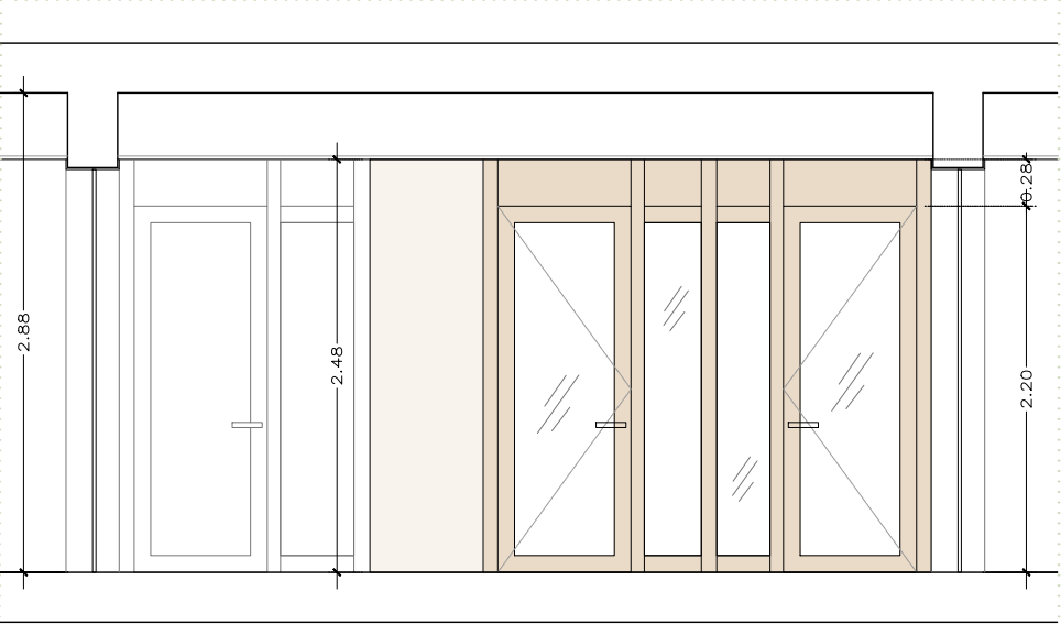
S2_SECCIÓ ACOTACIÓ
