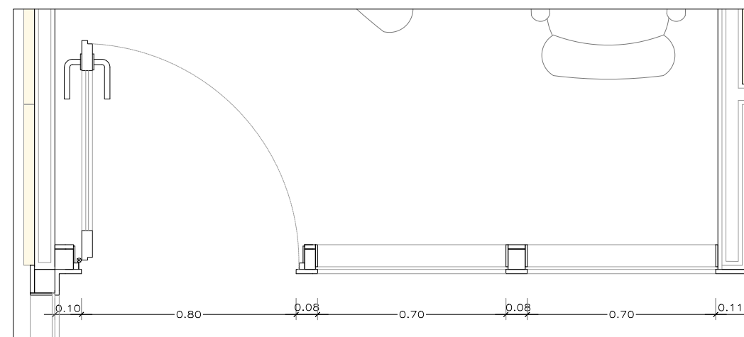
M2_MAMPARA
