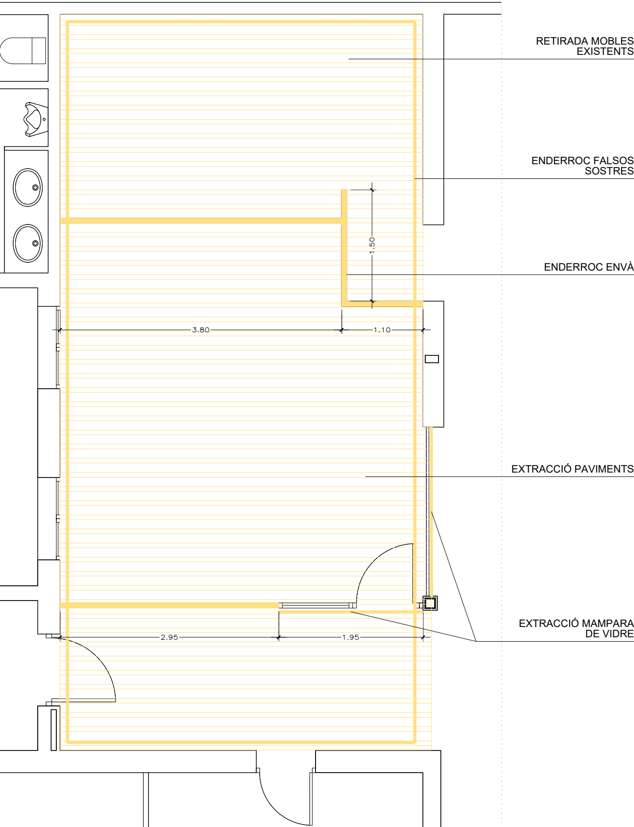
P2_ENDERROCS
