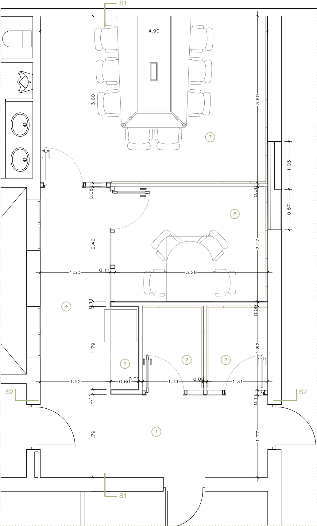
P3_PLANTA ACOTACIÓ
