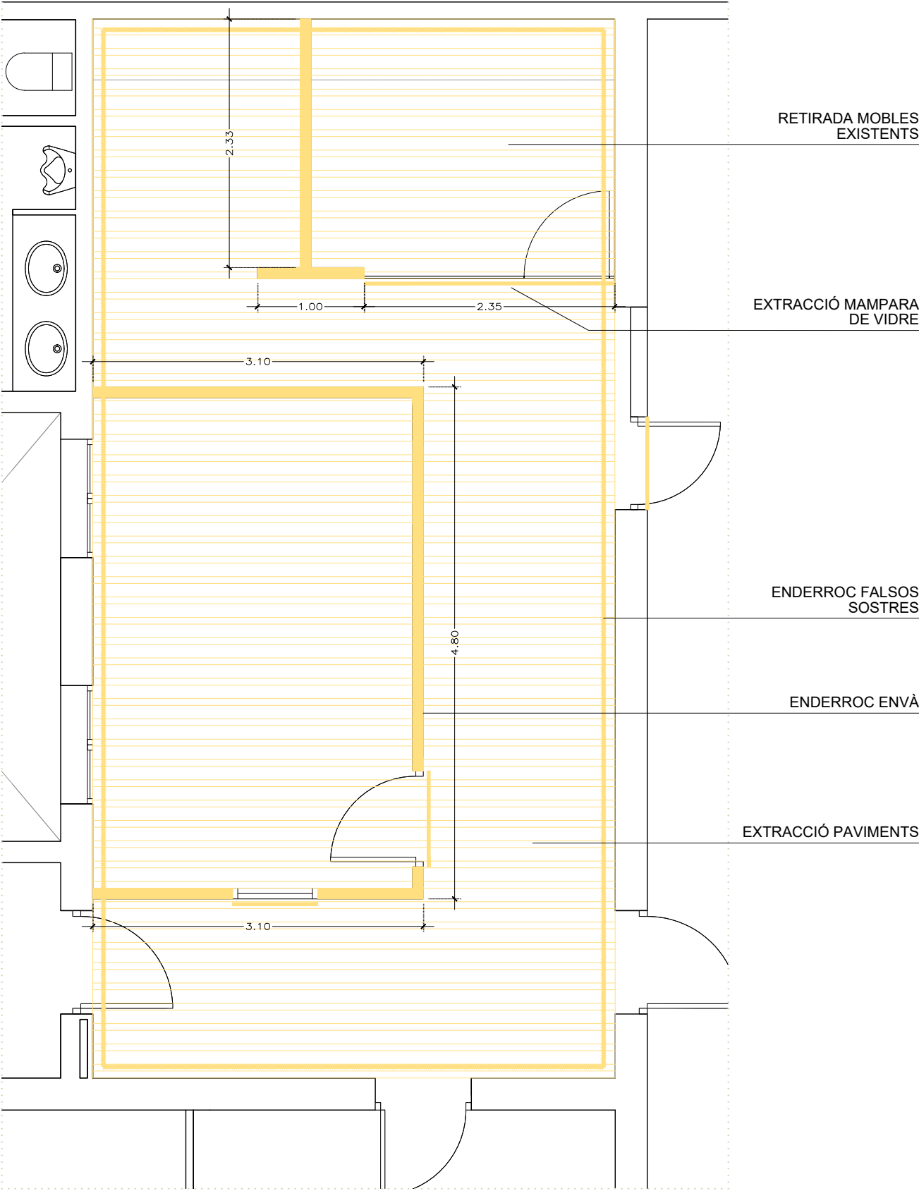
P3_ENDERROCS
