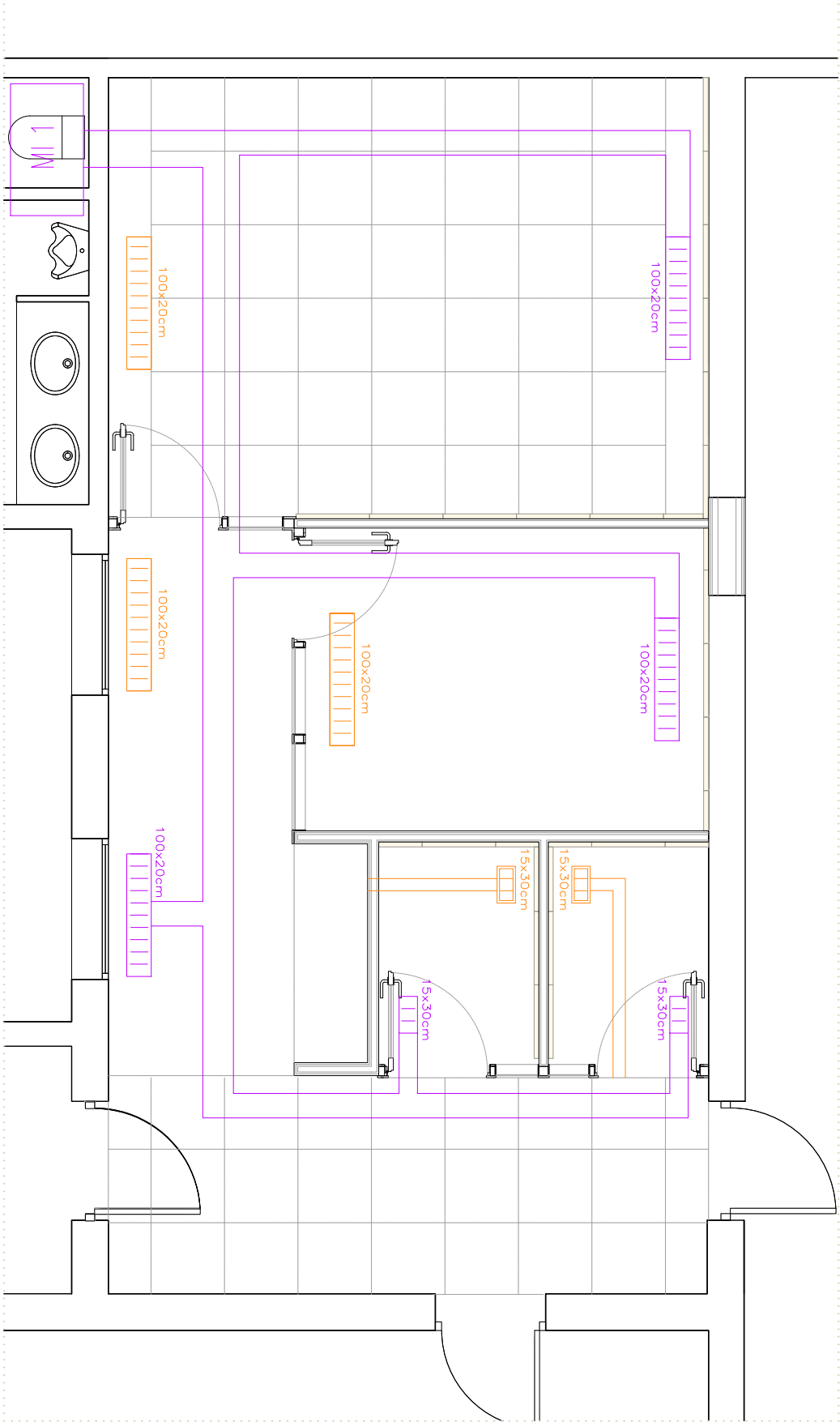
P1 / P2 / P3 _PROPOSTA CLIMA
