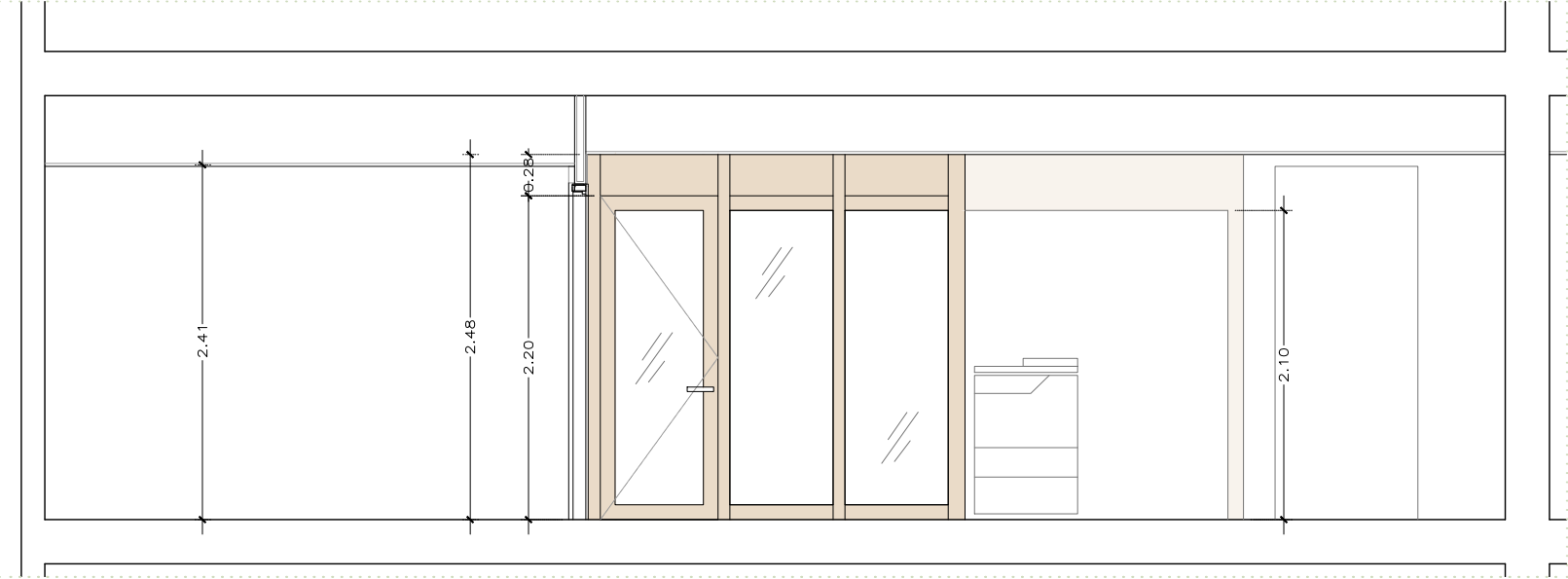
S1_SECCIÓ ACOTACIÓ
