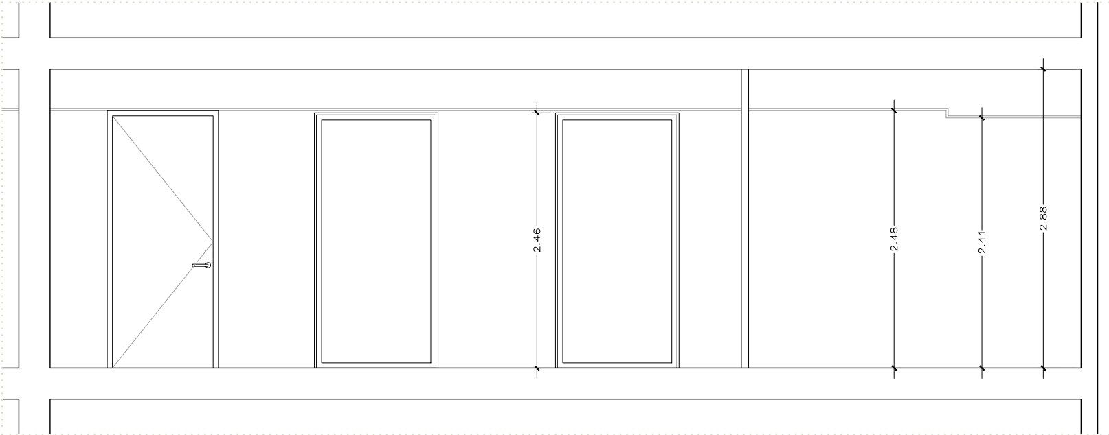
P1_SECCIÓ ACOTACIÓ
