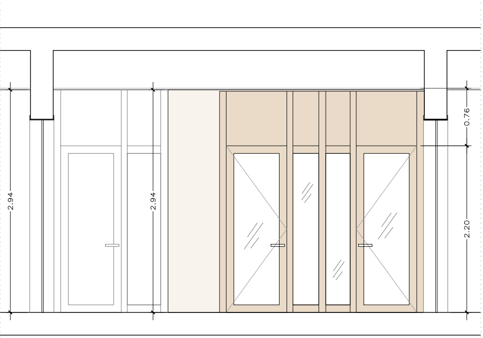
S2_SECCIÓ ACOTACIÓ
