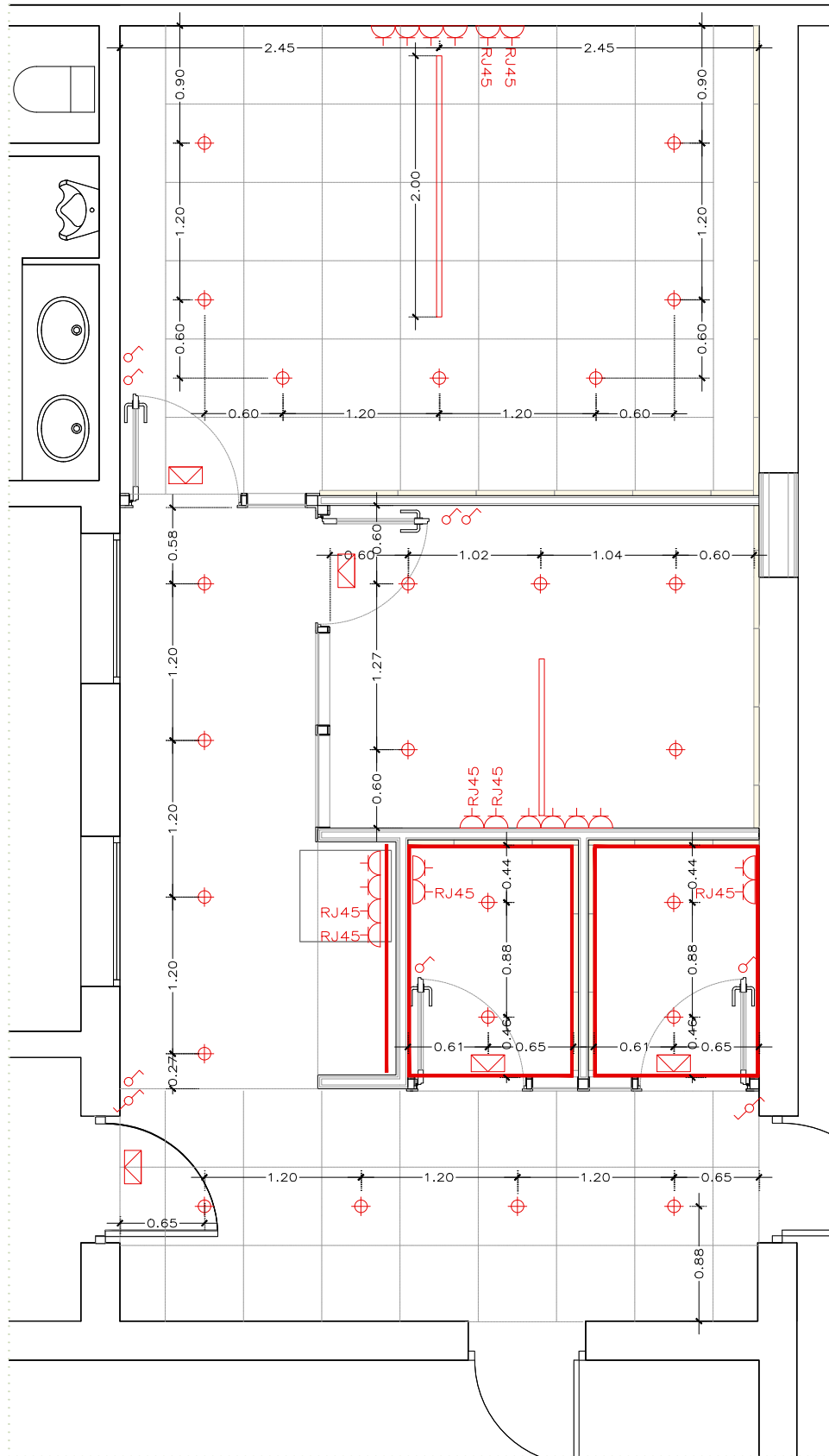
P1 / P2 / P3_ESQUEMA GENERAL ACOTACIÓ ENLLUMENAT
