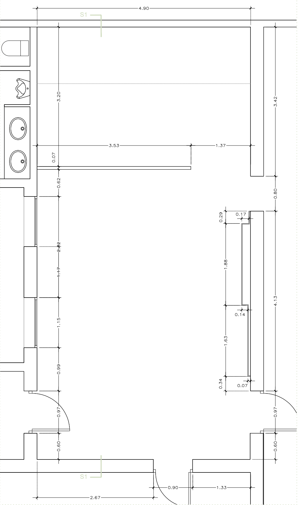
P1_PLANTA ACOTACIÓ
