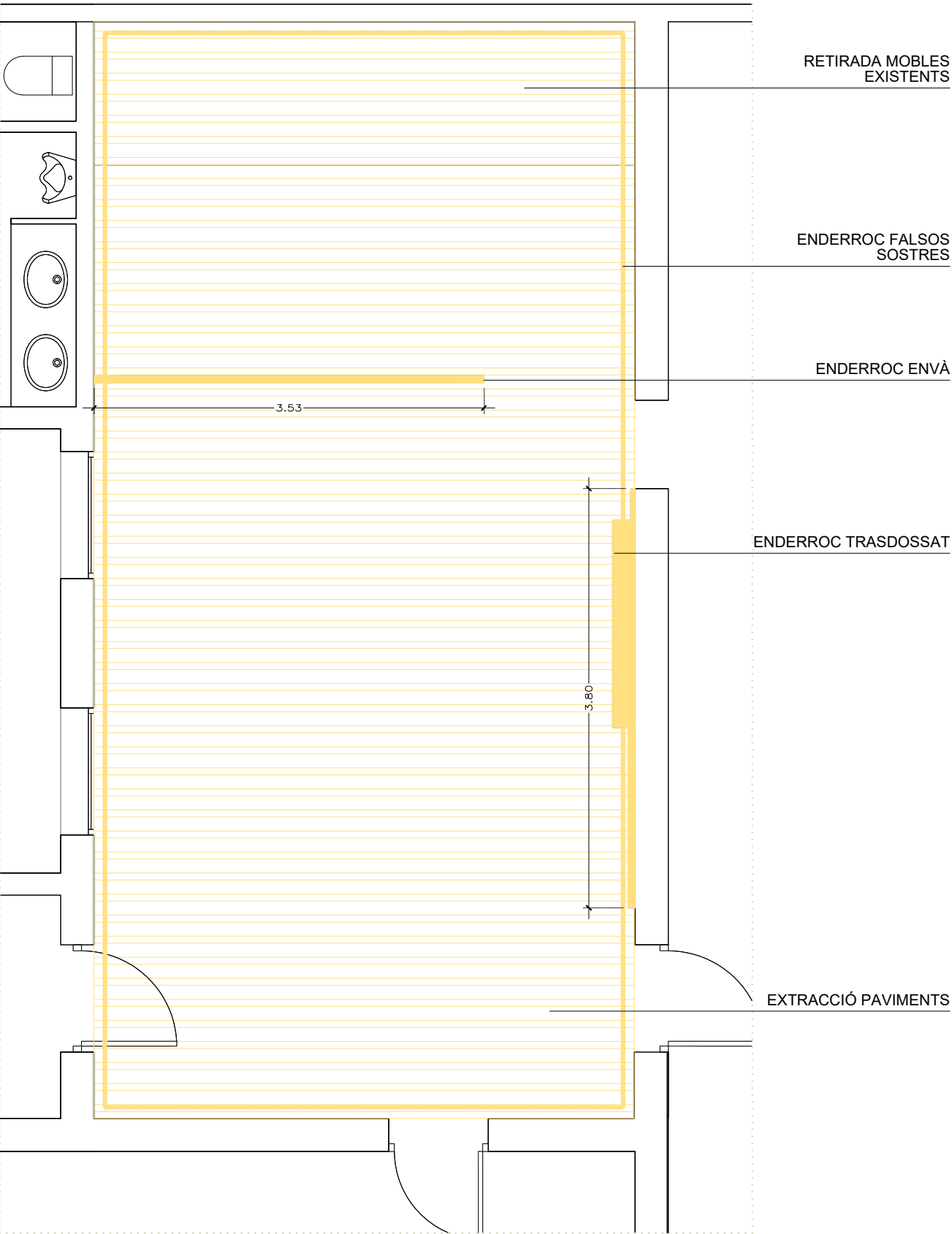
P1_ENDERROCS
