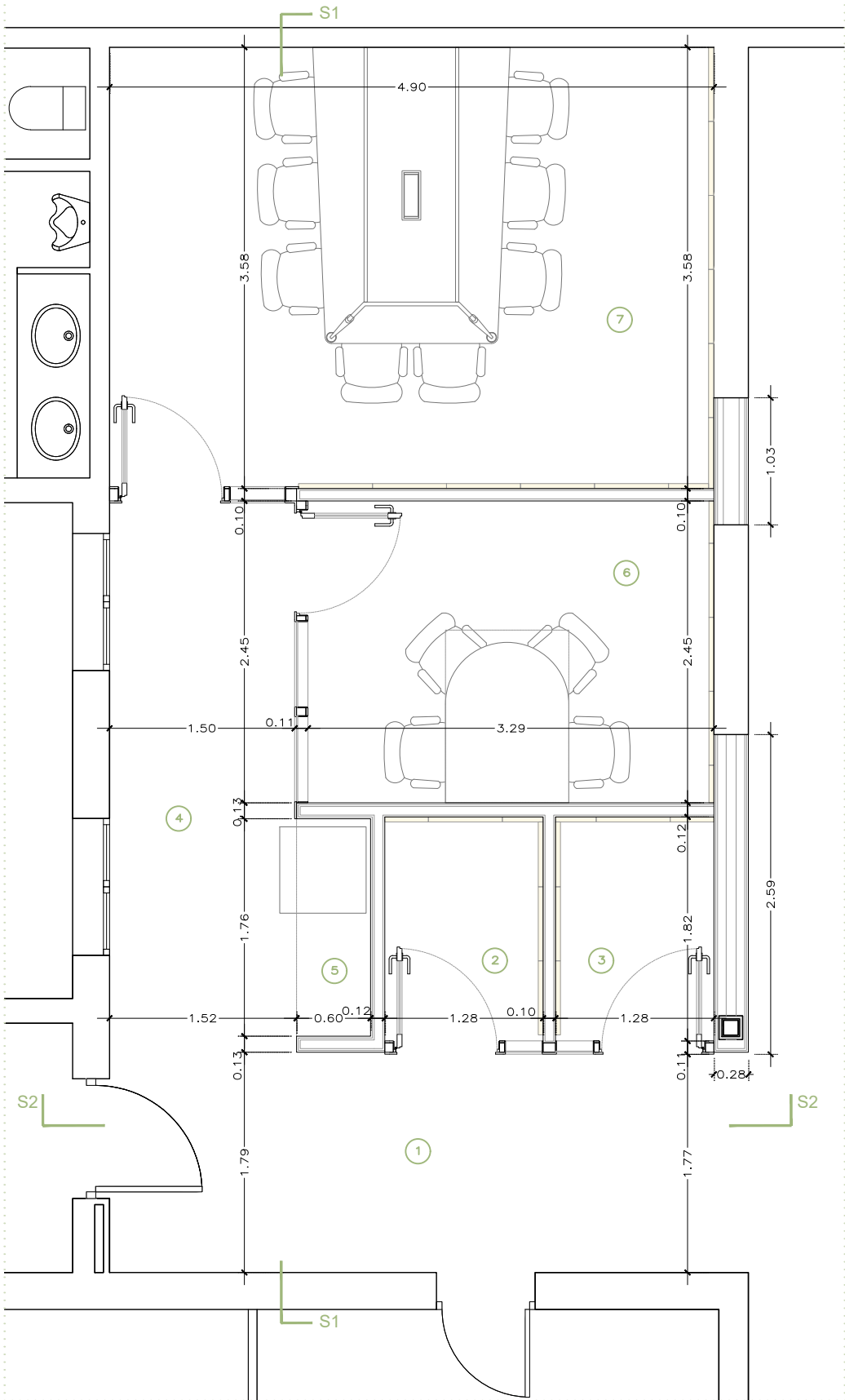
P2_PLANTA ACOTACIÓ
