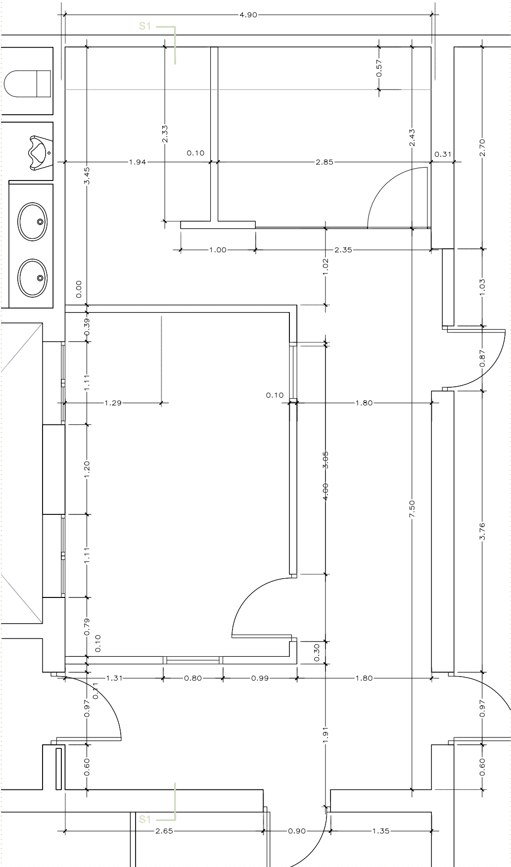
P3_PLANTA ACOTACIÓ
