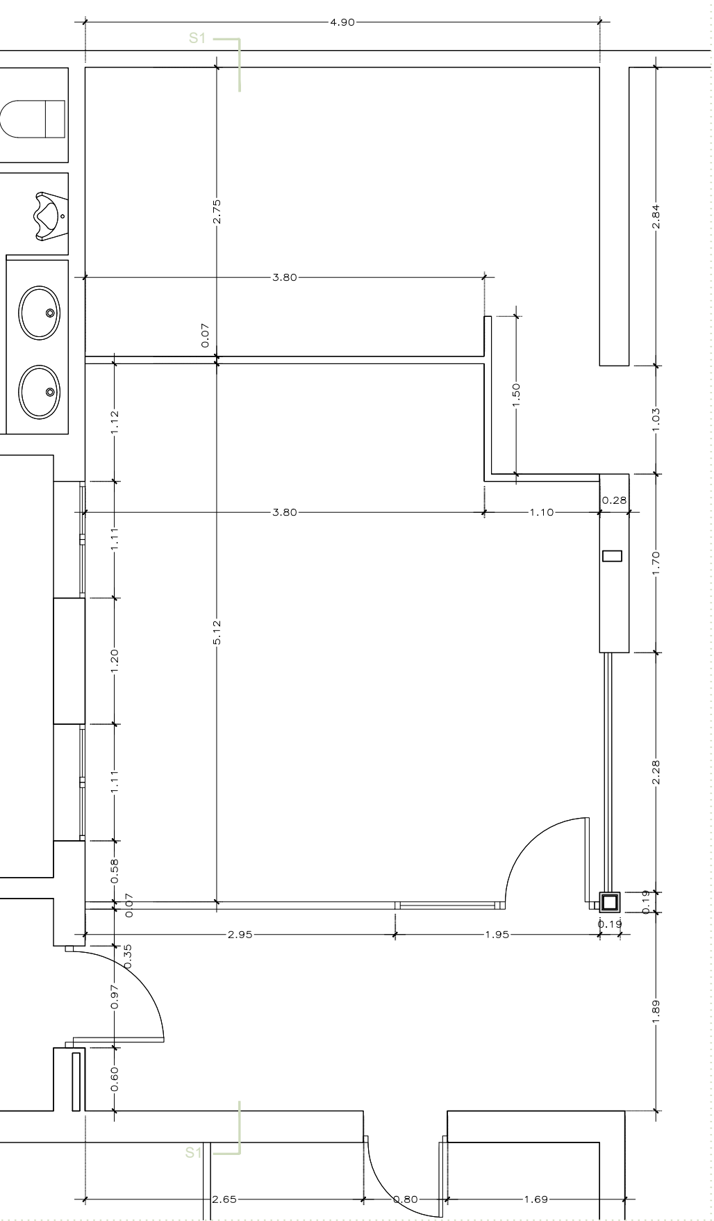
P2_PLANTA ACOTACIÓ
