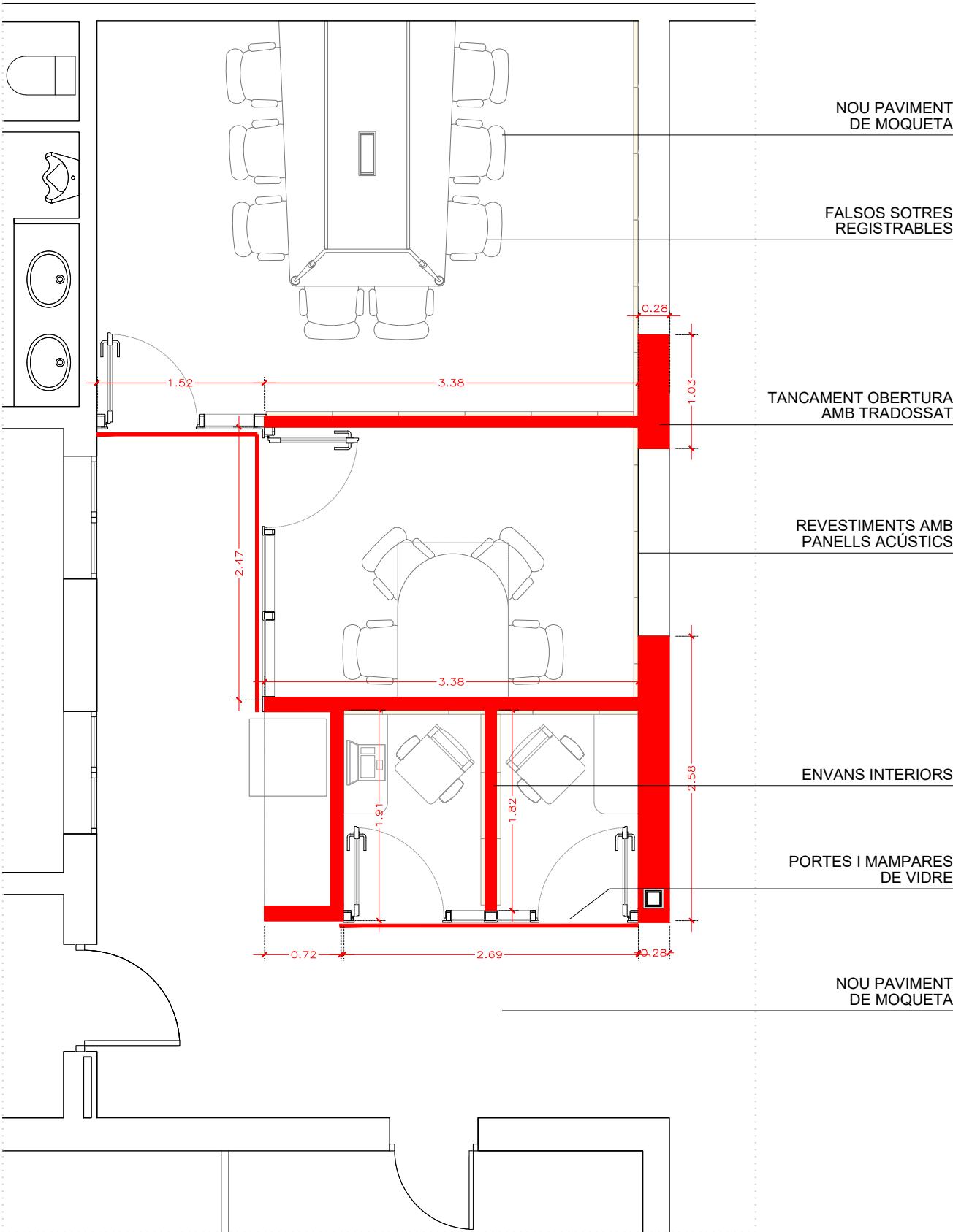
P2_OBRA
