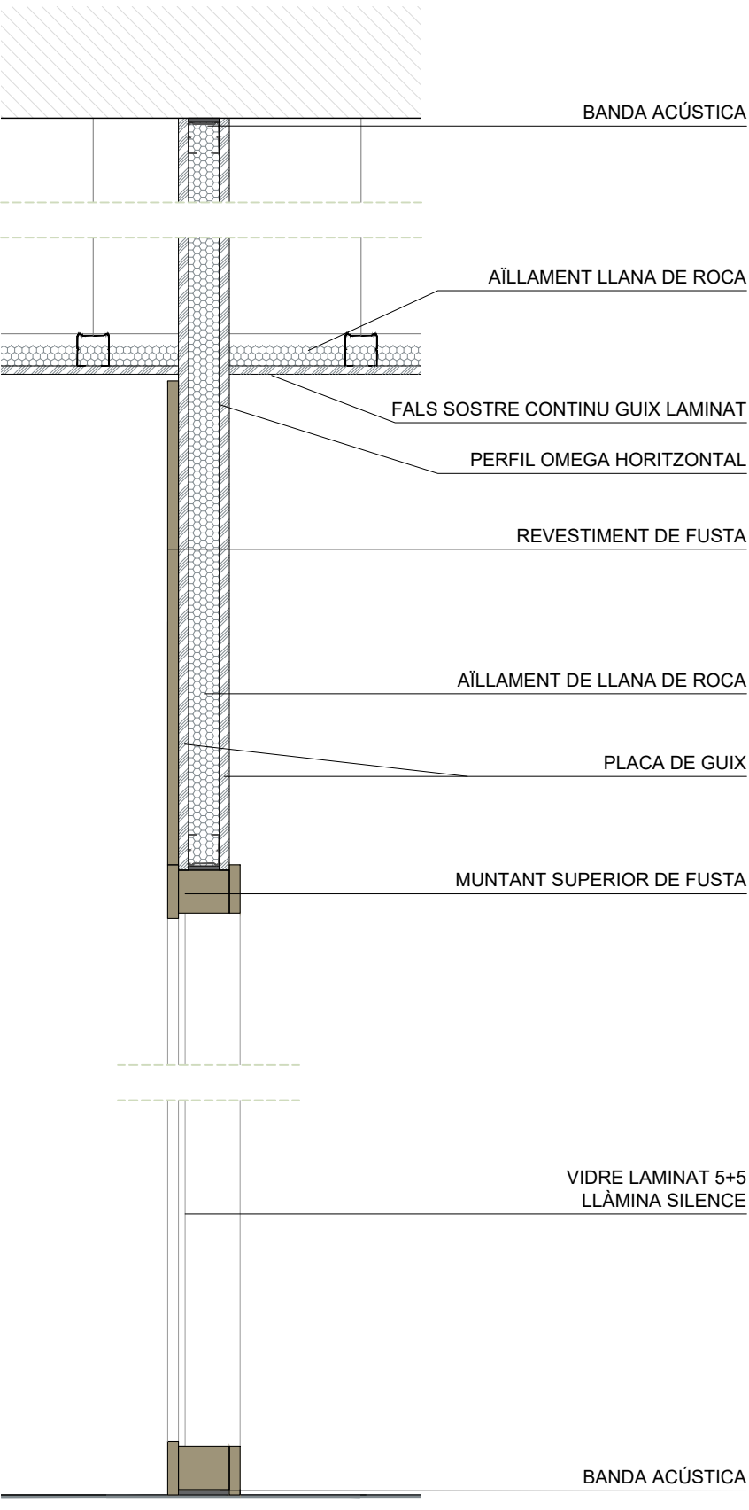
D2_DETALL MAMPARA (amb tabica superior)
