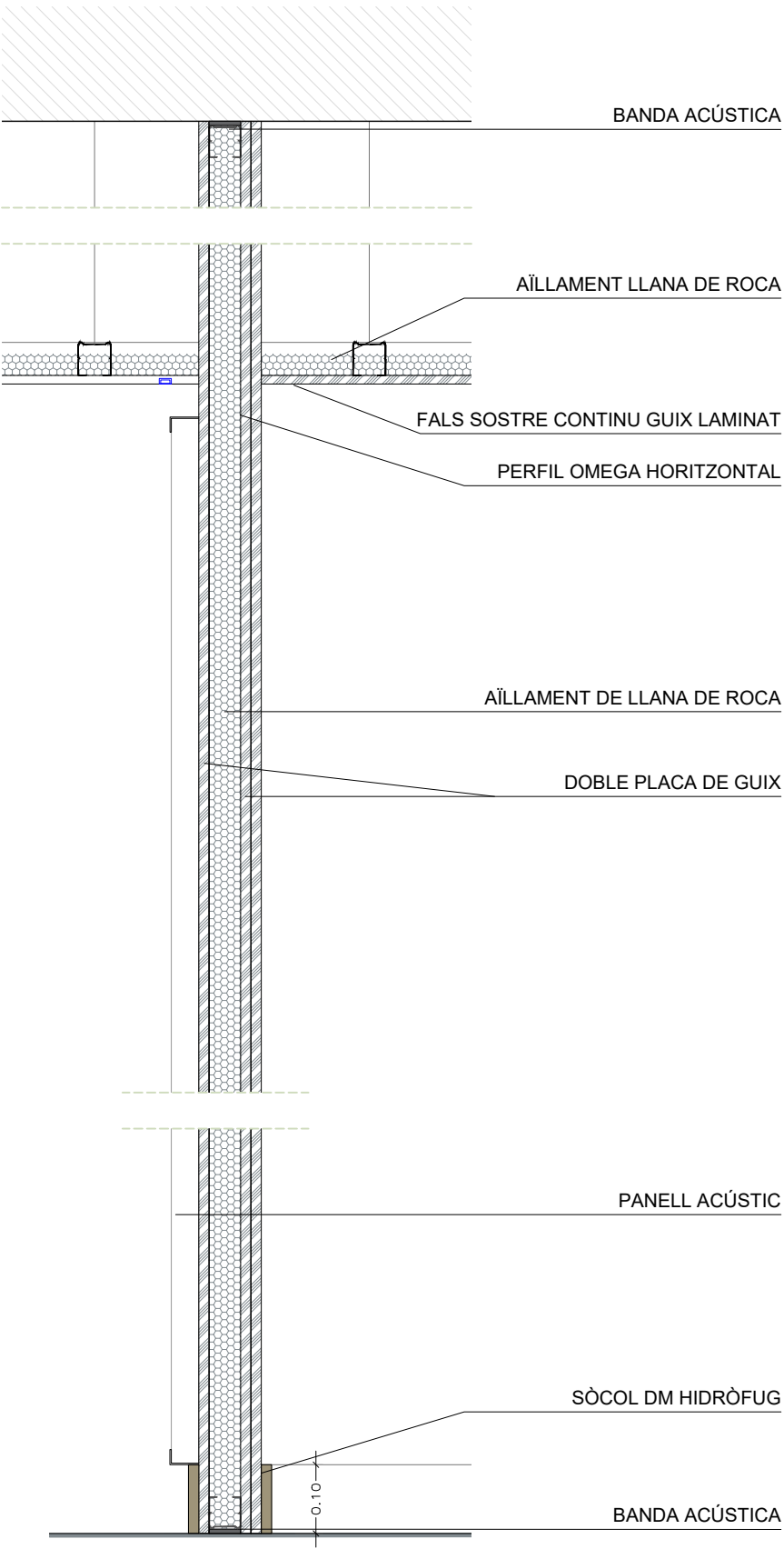
D1_DETALL ENVÀ (doble placa + panell acústic)
