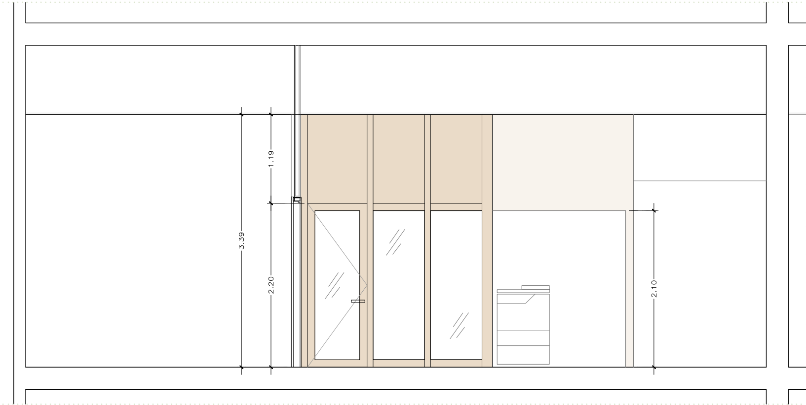
S1_SECCIÓ ACOTACIÓ
