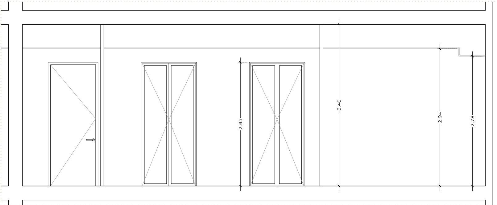
P3_SECCIÓ ACOTACIÓ
