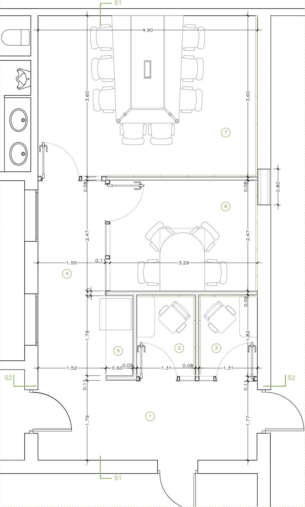
P1_PLANTA ACOTACIÓ
