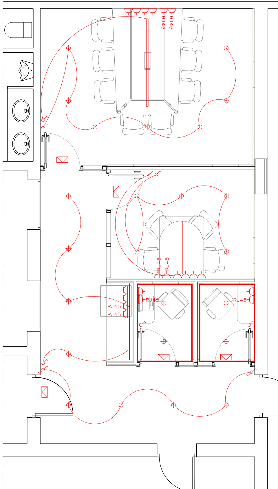
P1 / P2 / P3_ESQUEMA GENERAL ELECTRICITAT, TELECOM. I ENLLUMENAT
