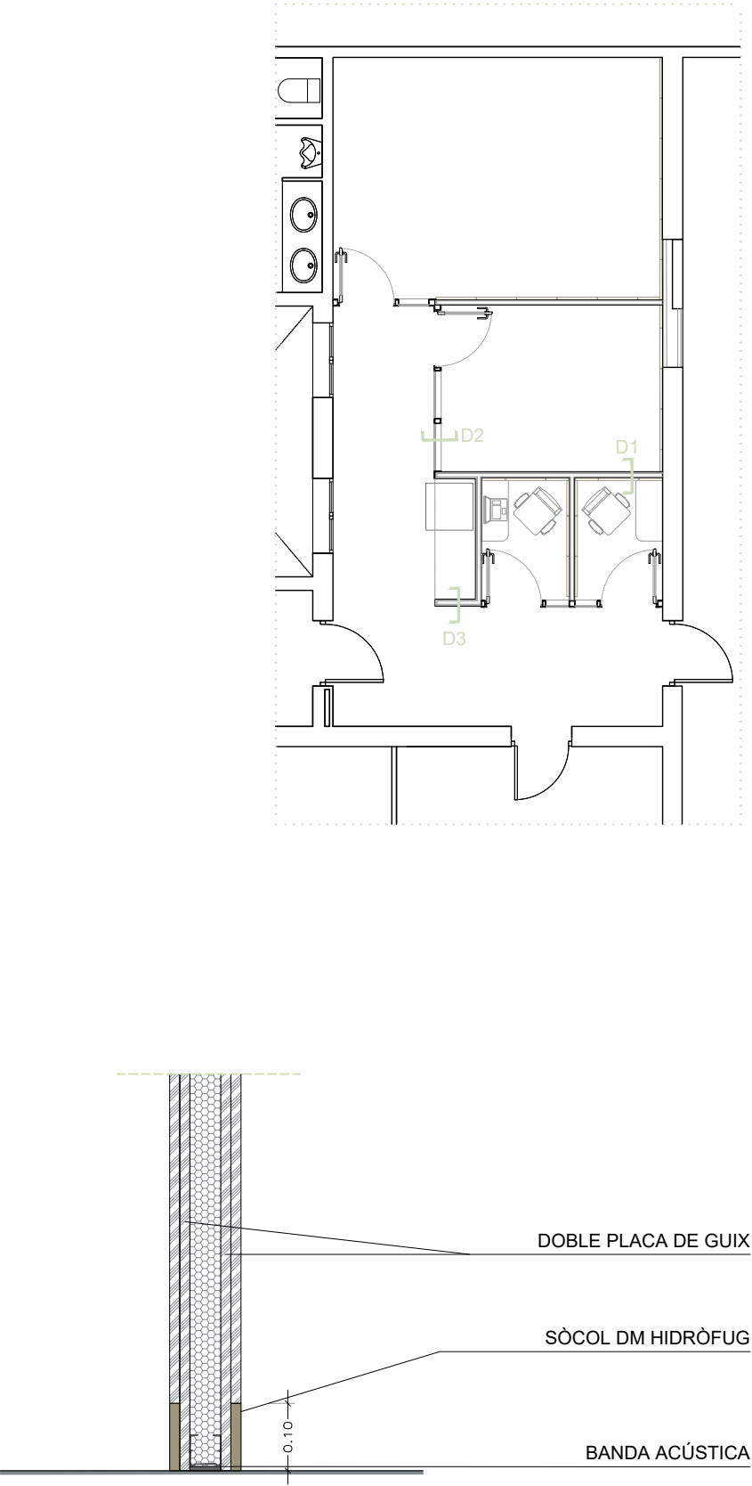
D3_DETALL ENVÀ REPROGRAFIA
