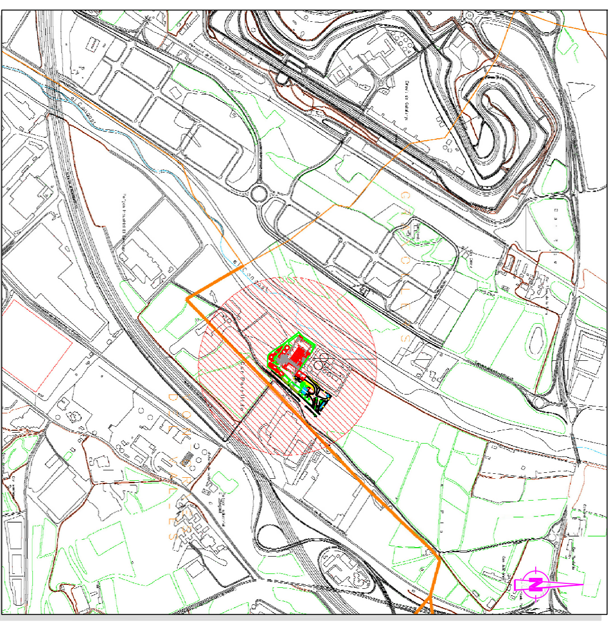
EMPLAÇAMENT ESCALA 1:2.500
