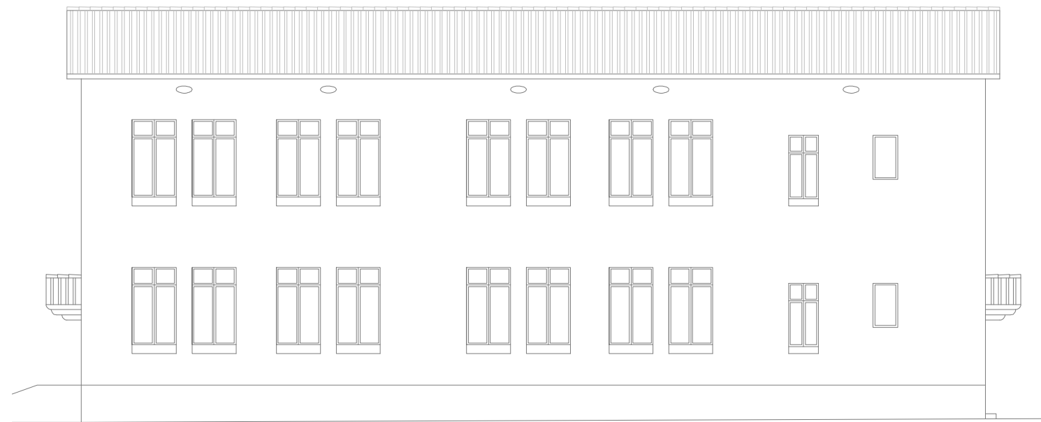
FAÇANA SUD
