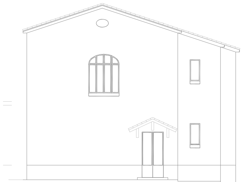
FAÇANA OEST
