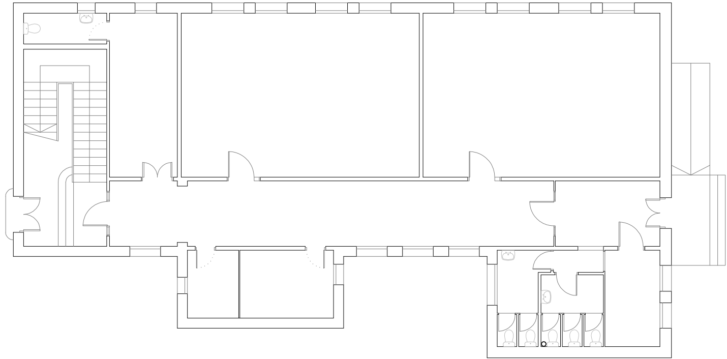
PLANTA BAIXA
