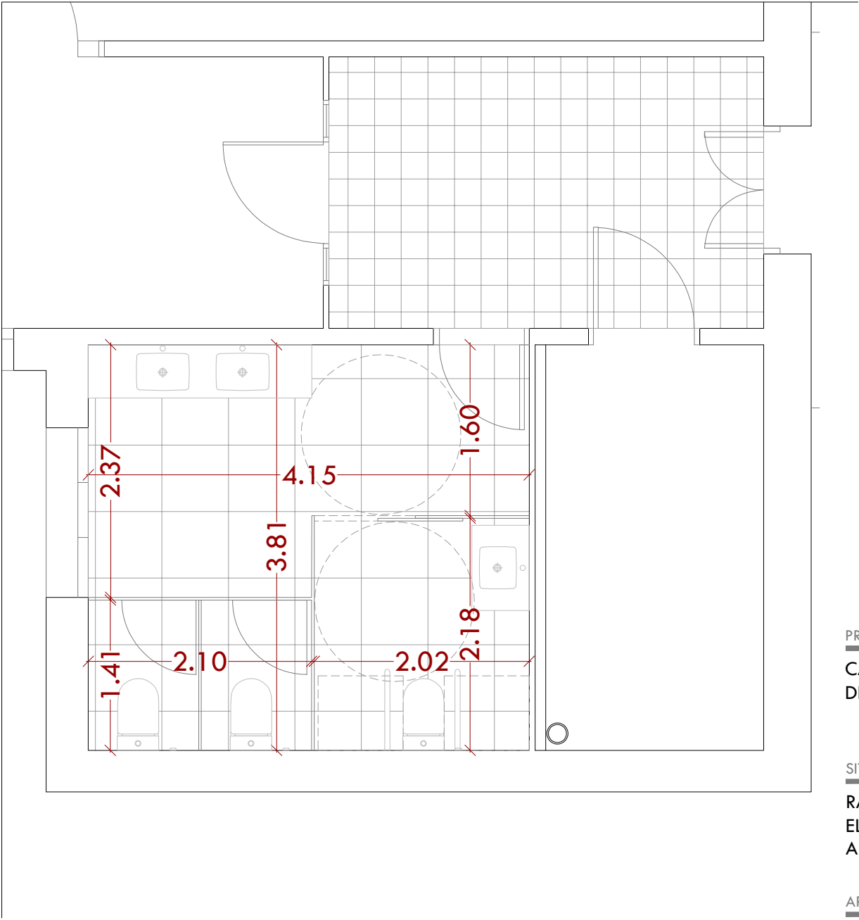
PROPOSTA DISTRIBUCIÓ
