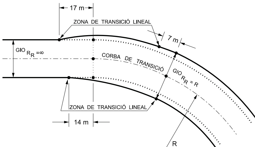
TRANSICIÓ DEL GÀLIB D'IMPLANTACIÓ D'OBSTACLES AMB CORBES DE TRANSICIÓ
