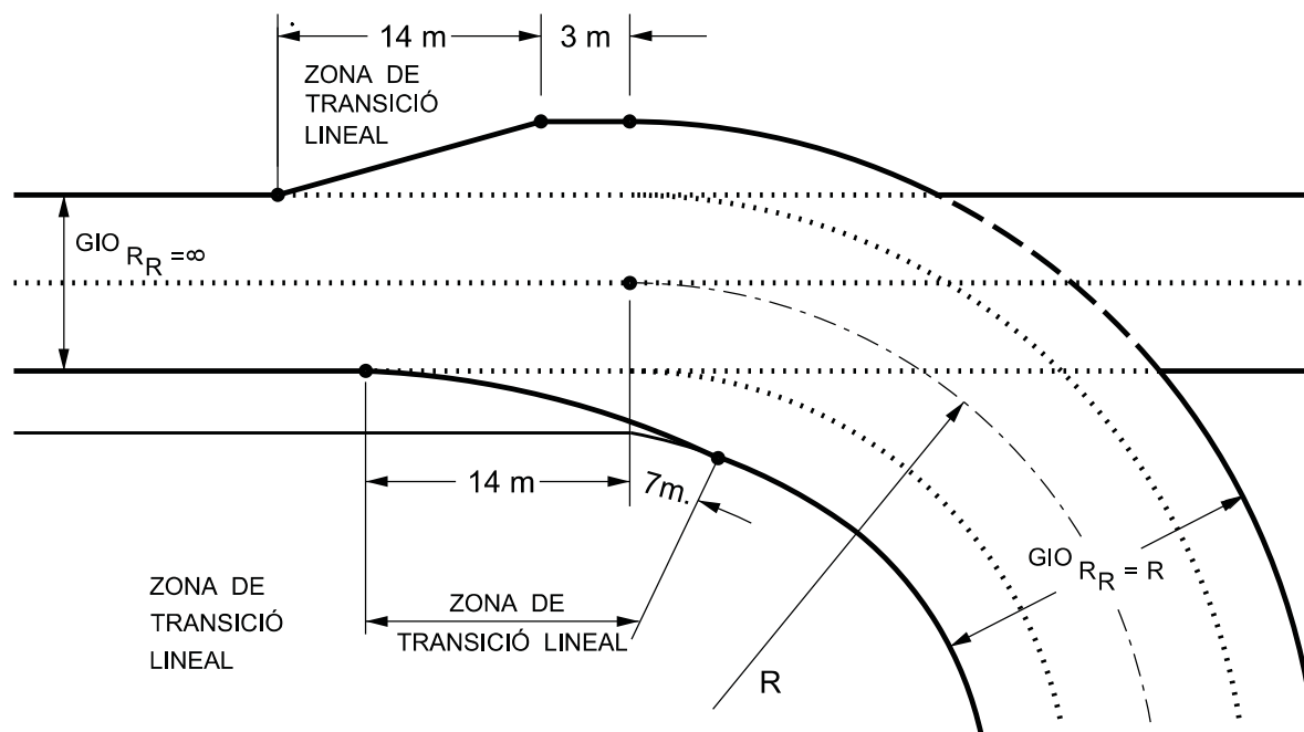
TRANSICIÓ DEL GÀLIB D'IMPLANTACIÓ D'OBSTACLES SENSE CORBES SENSE TRANSICIÓ
